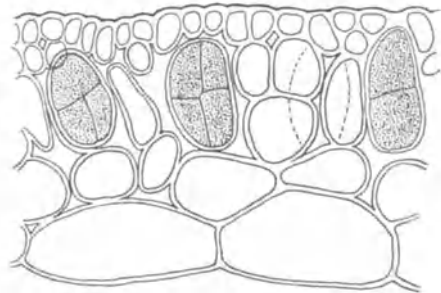
Fig. l. Tetrasporangien von Chrysymenia , in der Außenrinde.
