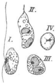
Fig. a. Kopulation von Phaeosporeen—Gameten.
