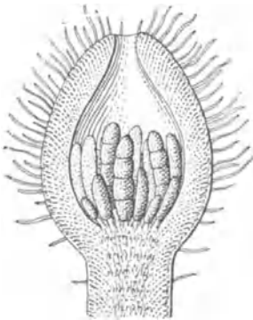
Fig. k. Corallina . Conceptakel mit Tetrasporangien.
