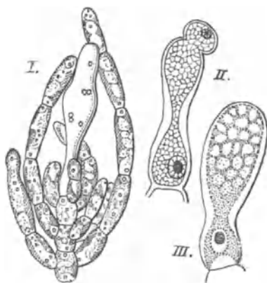
Fig. d. Batrachospermum . I. Karpogonzweig. II. Karpogon mit anhängendem Spermatium. III. Unbefruchtetes Karpogon mit dem Eikern.
