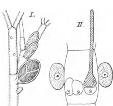
Fig. c. Callithamnium . I. Zweig mit Tetrasporen. II. Zweigzelle mit 2 Auxiliarmutterzellen und Karpogonzweig.
