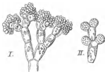
Fig. e. I. Teil eines Antheridienstandes von Helmiothora . II. Antheridien von Batrachospermum .
