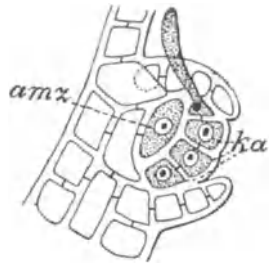
Fig. h. Rhodomela . ka=Karpogonzweig. amz=Auxiliarmutterzelle.
