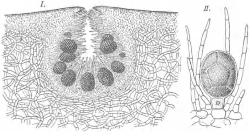
Fig. b. I. ♀ Conceptakel von Fucus . II. Oogonium und Paraphysen.
