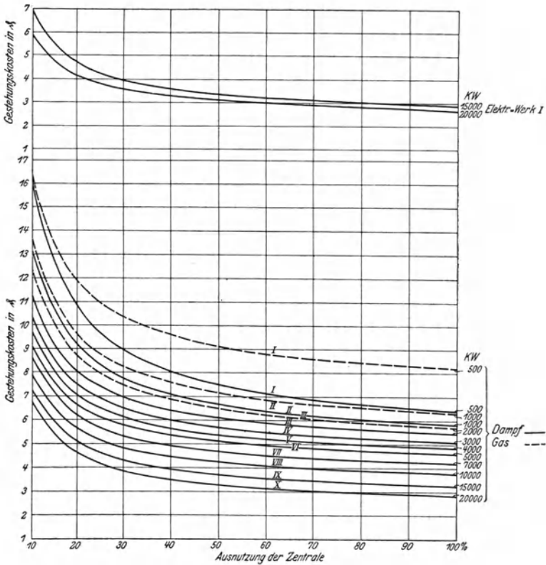
Fig. 12. Gestehungskosten in ihrer Abhängigkeit von der Leistung und Ausnutzung der Zentrale.
