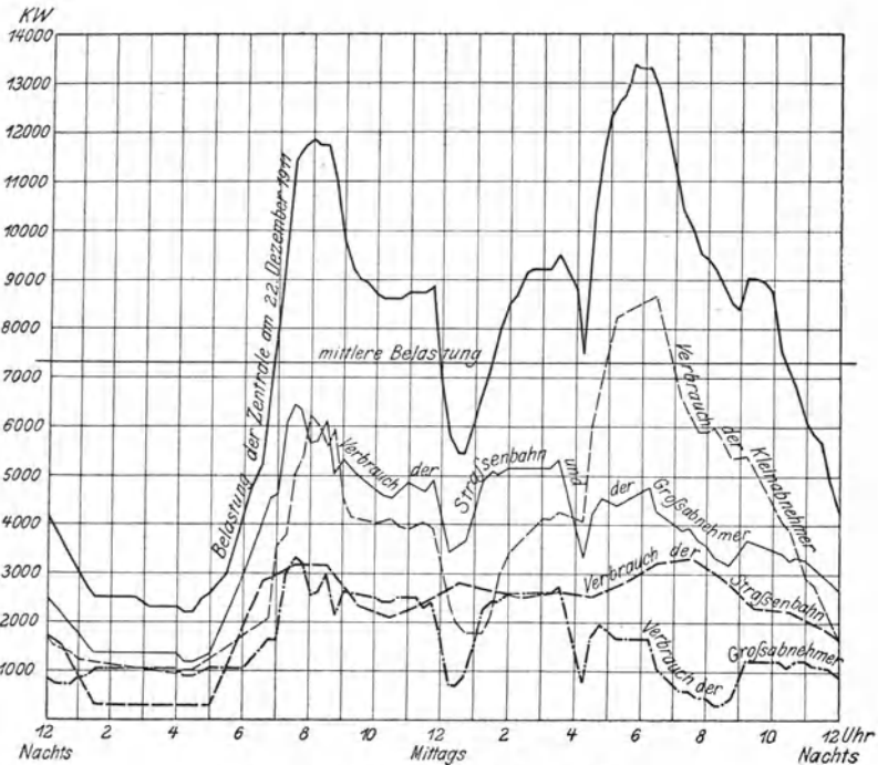
Fig. 2. Elektrizitätswerk I. (Winter.)
