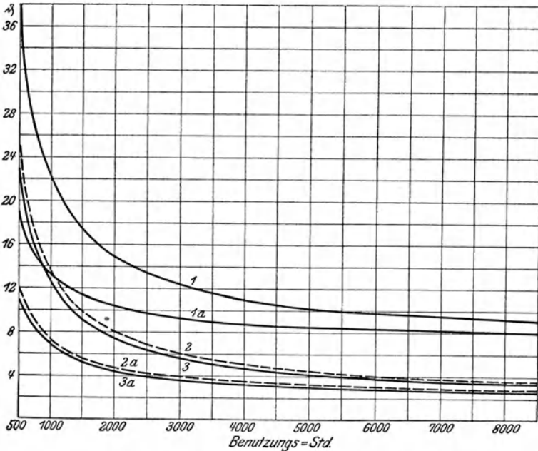
Fig. 16. Gestehungskosten pro nutzbare KWstd.
