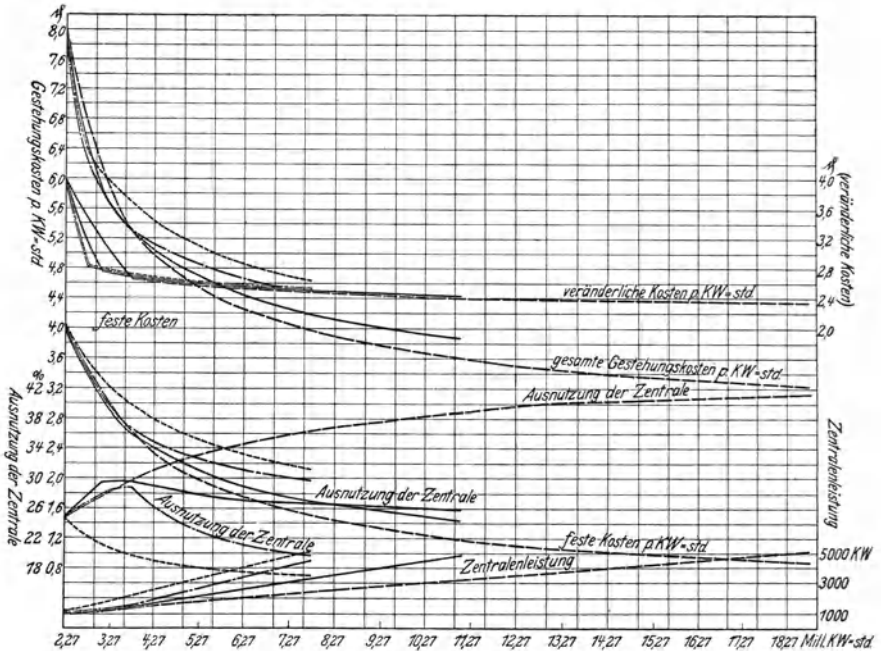
Fig. 10. Elektrizitätswerk III. Stromerzeugungskosten.
