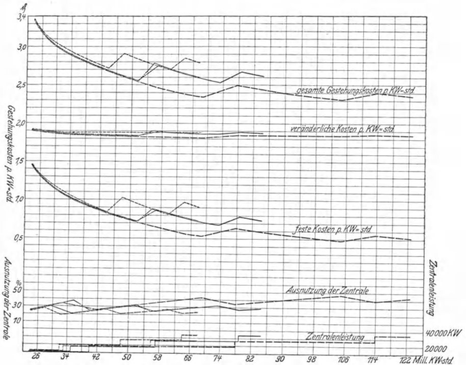
Fig. 9. Elektrizitätswerk II. Stromerzeugungskosten.
