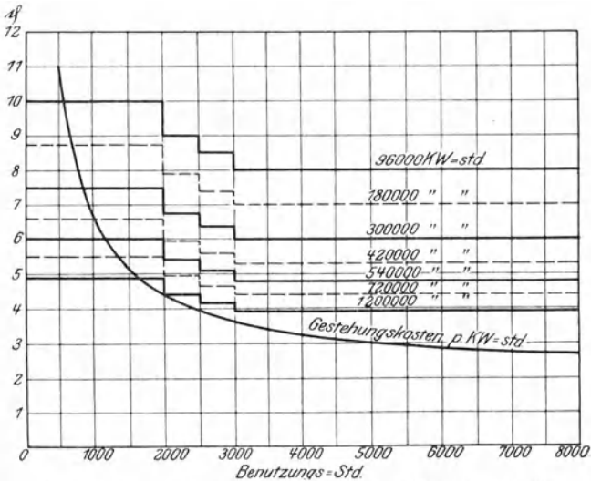
Fig. 24. Großabnehmertarif des Elektrizitätswerkes I.
