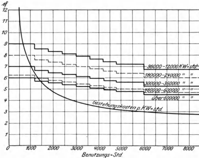
Fig. 25. Sondertarif für Großabnehmer des EW II.
