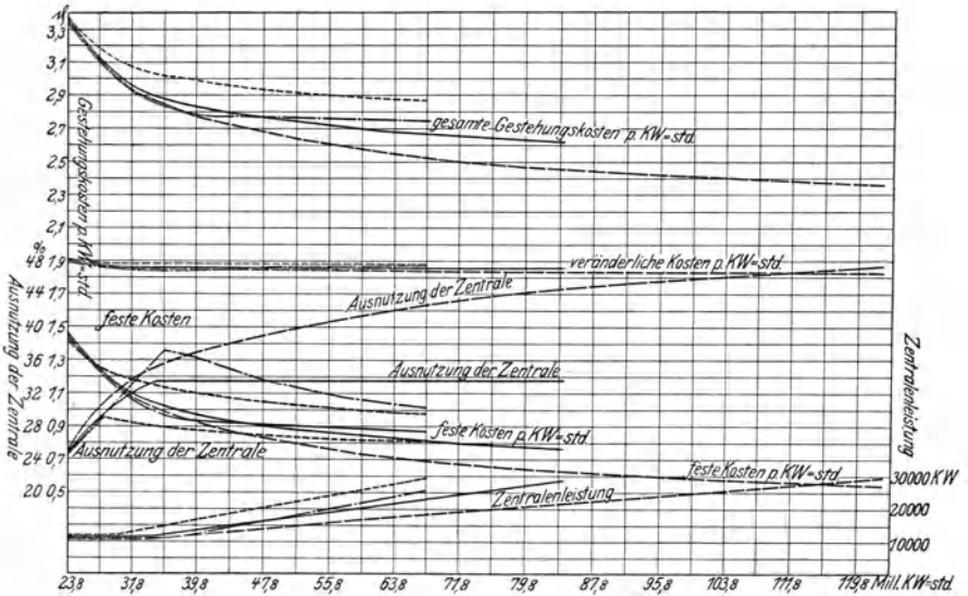
Fig. 8. Elektrizitätswerk II. Stromerzeugungskosten.
