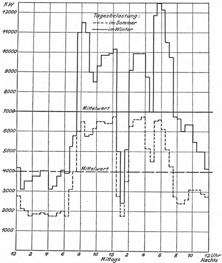
Fig. 4. Elektrizitätswerk II.
