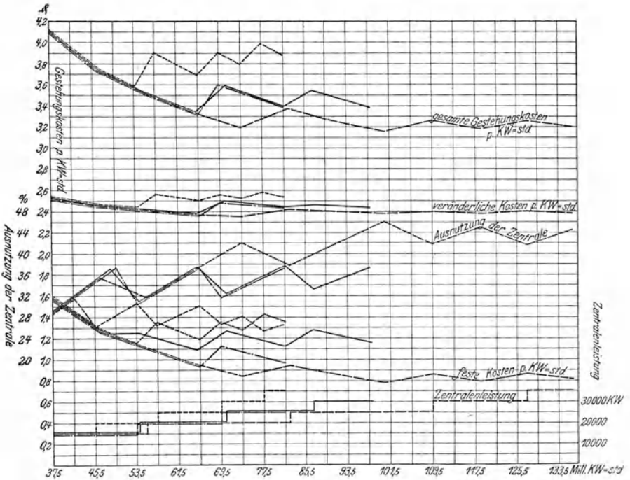
Fig. 7. Elektrizitätswerk I. Stromerzeugungskosten.
