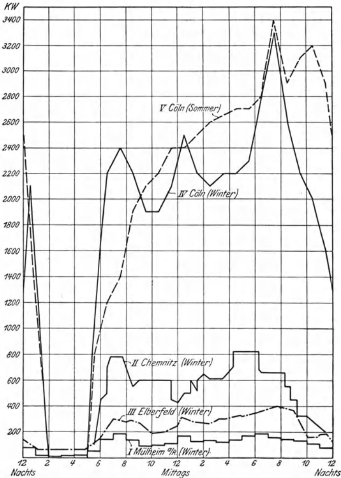
Fig. 13. Stromverbrauch städtischer Straßenbahnen.
