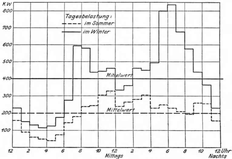
Fig. 5. Elektrizitätswerk III.
