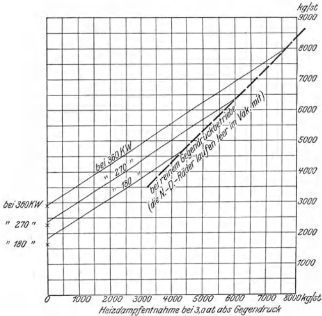
Fig. 26. Gesamt-Dampfverbrauch einschließlich Heizdampf von 3 at. ab Gegendruck und ca. 170° C.
