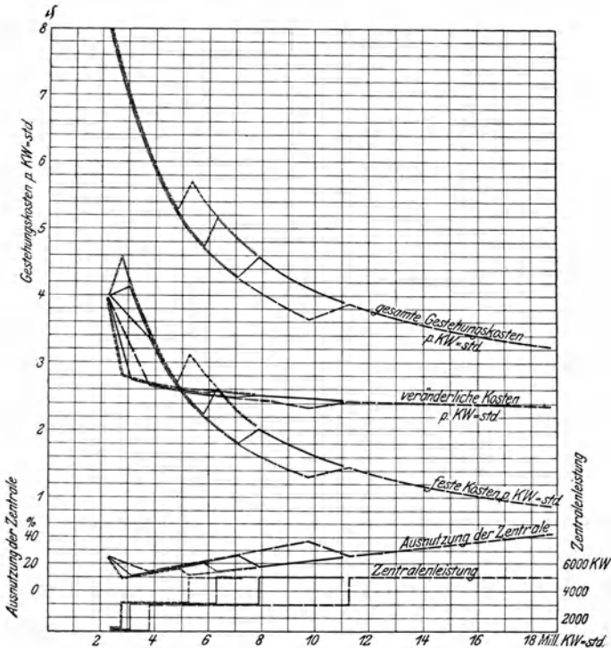
Fig. 11. Elektrizitätswerk III. Stromerzeugungskosten.
