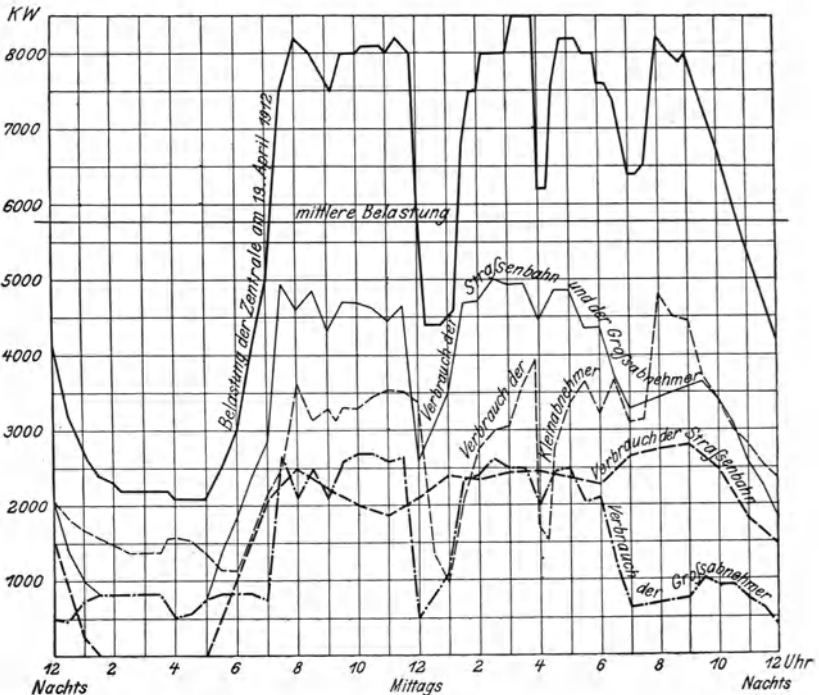
Fig. 3. Elektrizitätswerk I. (Sommer.)
