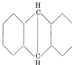
Anthracen.
