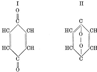
Chinon.
