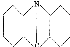
H Acridin.
