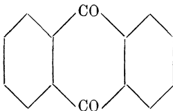
Anthrachinon.
