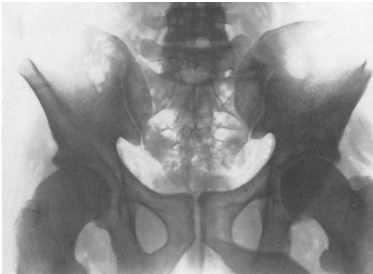
Abb. 9. Einseitige Sacralisation.
