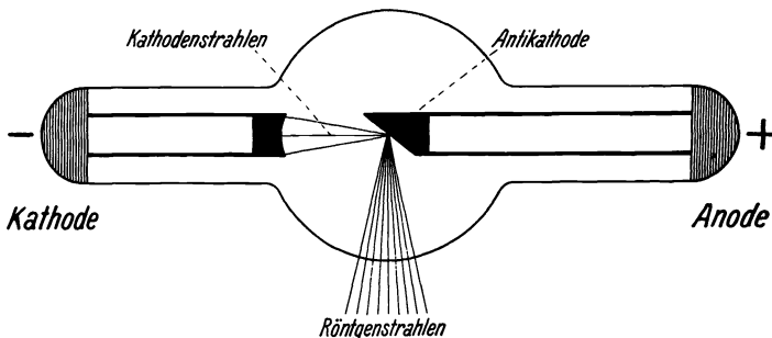
Abb. 1. Röntgenröhre.
