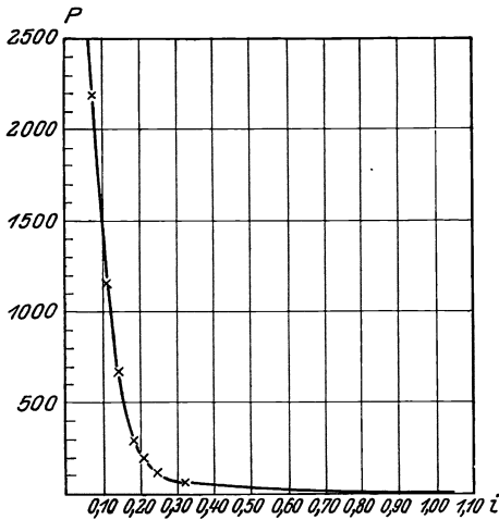
Abb. 32. Quellungsdruck von Kasein.
