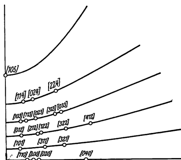
Abb. 9. Die Anordnung der Interferenzen auf Schichtlinien im Diagramm von Zellulose. Fasern, welche eine Orientierung der Kristallite parallel der Faserachse haben. (Nach M. POLANYI, Naturwissenschaften, Jahrg. 9, Heft 18, Abb. 4.)
