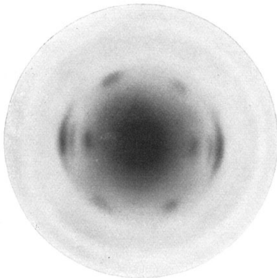
Abb. 21. Diagramm eines Bündels von parallelen Ramiefasern, gequollen (24 Stunden) in Zinkchlorid-Lösung (1,80 spez. Gew.) und im Quellungsmittel aufgenommen. Eigene Aufnahme. Abstand 47\frac{1}{2} m. M., genau gleicher Abstand wie in Abb. 7. Natürliche Größe.
