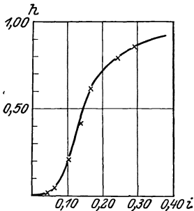
Abb. 24. Isotherme von Serumalbumin.
