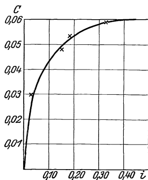
Abb. 31. Volumkontraktion von künstlichen Stärkekörnern.
