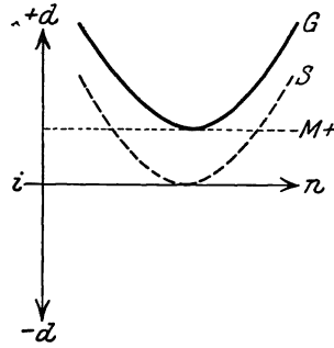
Abb. 2. Schema für das Zusammenwirken von Stäbchendoppelbrechung ( S ) mit positiver Mizellardoppelbrechung ( M+ ) zur Gesamtdoppelbrechung G (im übrigen vgl. Abb. 1). (Aus Naturw. XII, 297, 1924).
