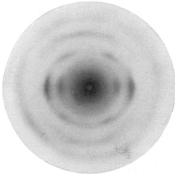
Abb. 7. Das Vierpunktdiagramm von parallel orientierten luftgetrockneten Ramiefasern. Die vertikale Mittellinie fällt mit der Faserrichtung zusammen, die horizontale mit dem Äquator. Abstand 47\frac{1}{2} m. M. Eigene Aufnahme. Natürliche Größe.
