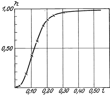
Abb. 22. Isotherme von Kasein.
