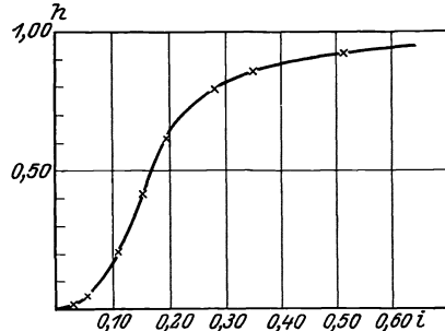
Abb. 25. Isotherme von Gummi arabicum.
