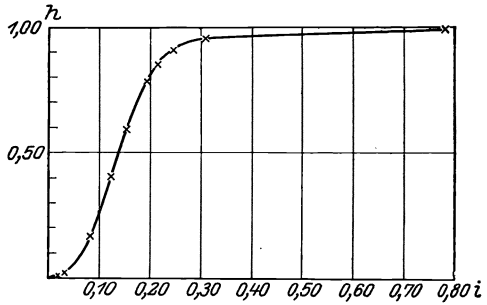
Abb. 23. Isotherme von Nuklein.
