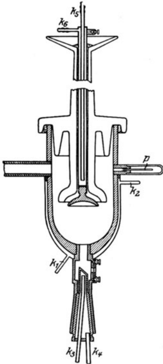
Abb. 4. Röntgenröhre aus Metall nach HADDING und SIEGBAHN (nach CERMAK, die Röntgenstrahlen, S. 31, Abb. 42).
