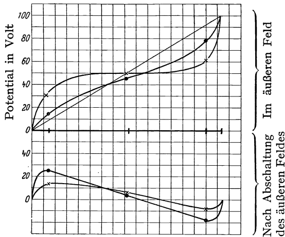
Abb. 2. Zeitliche Änderung der Potentialverteilung in einem Quarzkristall (3 Mittelsonden). Temp. 157^\circ . Aus Annalen der Physik Bd. 72, Arb. JOFFÉ.
