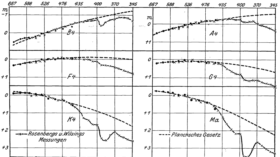
Abb. 2. Mittlere Energiekurven einzelner Spektraltypen (aus Naturwissenschaften, XII, 699, 1924).
