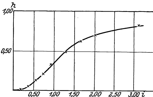
Abb. 33. Isotherme von Schwefelsäure (und Wasser).
