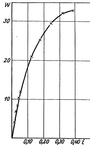
Abb. 29. Quellungswärme von künstlichen Stärkekörnern.
