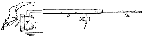
Abb. 1. Behälter für die Thermoelemente in der COBLENTZschen Konstruktion (aus Popular Astronomy, Vol. XXXI, No. 2, Plate V, Fig. 3).
