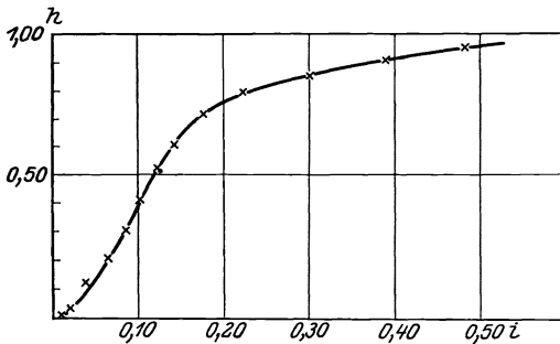
Abb. 26. Isotherme von schön ausgebildeten Kohlenoxydhämoglobin-Kristallen.
