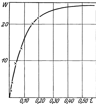
Abb. 28. Quellungswärme von Kasein.
