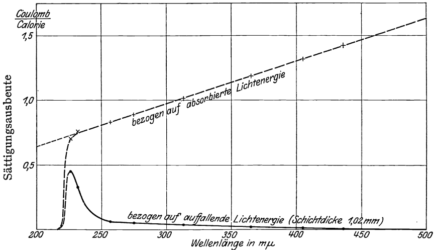
Abb. 4. Spektrale Verteilung der lichtelektrischen Leitfähigkeit (Primärstrom) an einem reinen Diamantkristall.
