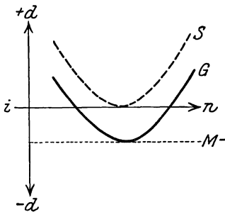
Abb. 3. Schema für das Zusammenwirken von Stäbchendoppelbrechung ( S ) mit negativer ( M- ) zur Gesamtdoppelbrechung G (im übrigen vgl. Abb. 1).
