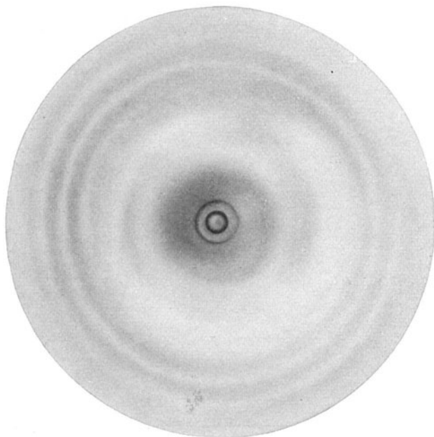
Abb. 20. Diagramm eines Bündels von parallelen Ramiefasern, gequollen (24 Stunden) in gesättigter Lösung von LiOH und im Quellungsmittel aufgenommen. Eigene Aufnahme. Abstand 47\frac{1}{2} m. M., genau gleicher Abstand wie in Abb. 7. Natürliche Größe.
