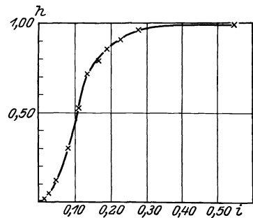
Abb. 27. Isotherme von schön ausgebildeten Vitellin-Kristallen (aus Kürbissamen).
