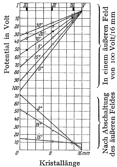
Abb. 1. Zeitliche Änderung der Potentialverteilung in einem Kalkspatkristall. Aus Annalen der Physik, Bd. 72, Arb. JOFFÉ. II, III, IV sind Sonden. Temp. 157^\circ .
