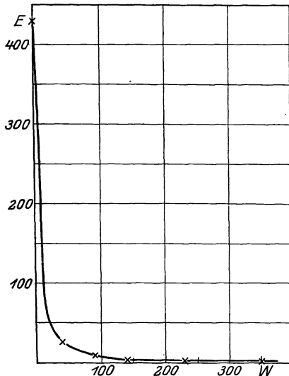
Abb. 38. Elastizitätsmodul von Laminaria.
