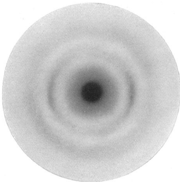
Abb. 19. Diagramm eines Bündels von parallelen Ramiefasern nach 24-stündiger Quellung in 12% NaOH, im Quellungsmittel aufgenommen. Eigene Aufnahme. Abstand 47\frac{1}{2} m. M., genau gleicher Abstand wie in Abb. 7. Natürliche Größe.
