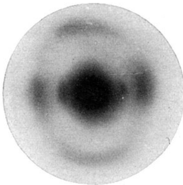
Abb. 14. Diagramm eines aus parallelen Fasern bestehenden Bündels von Nitroramie. Luftgetrocknet. Eigene Aufnahme. Abstand 36 m. M. Natürliche Größe.
