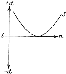
Abb. 1. Schema für den Verlauf reiner Stäbchendoppelbrechung ( S ) bei Durchtränkung des Stäbchensystems mit Flüssigkeiten vom steigenden Brechungsindex -n ; i Linie der Isotropie +d positive, -d negative Doppelbrechung.
