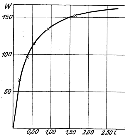
Abb. 34. Mischungswärme von Schwefelsäure (und Wasser).
