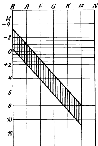
Abb. 1. Das Russellsche Diagramm in schematischer Darstellung. Abszisse ist das Spektrum, Ordinate die absolute Helligkeit. Die große Masse der Sterne ist auf zwei Streifen verteilt: Die häufigen Zwergsterne auf dem vertikal-schraffierten Streifen, die selteneren Riesen auf dem horizontal-schraffierten Streifen.
