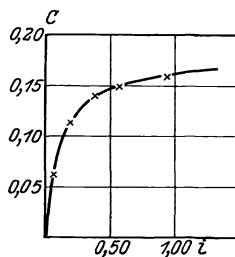
Abb. 35. Volumkontraktion von Schwefelsäure (und Wasser).
