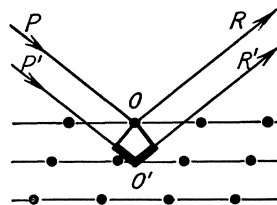
Abb. 5. Zur Braggschen Reflexionsformel.
