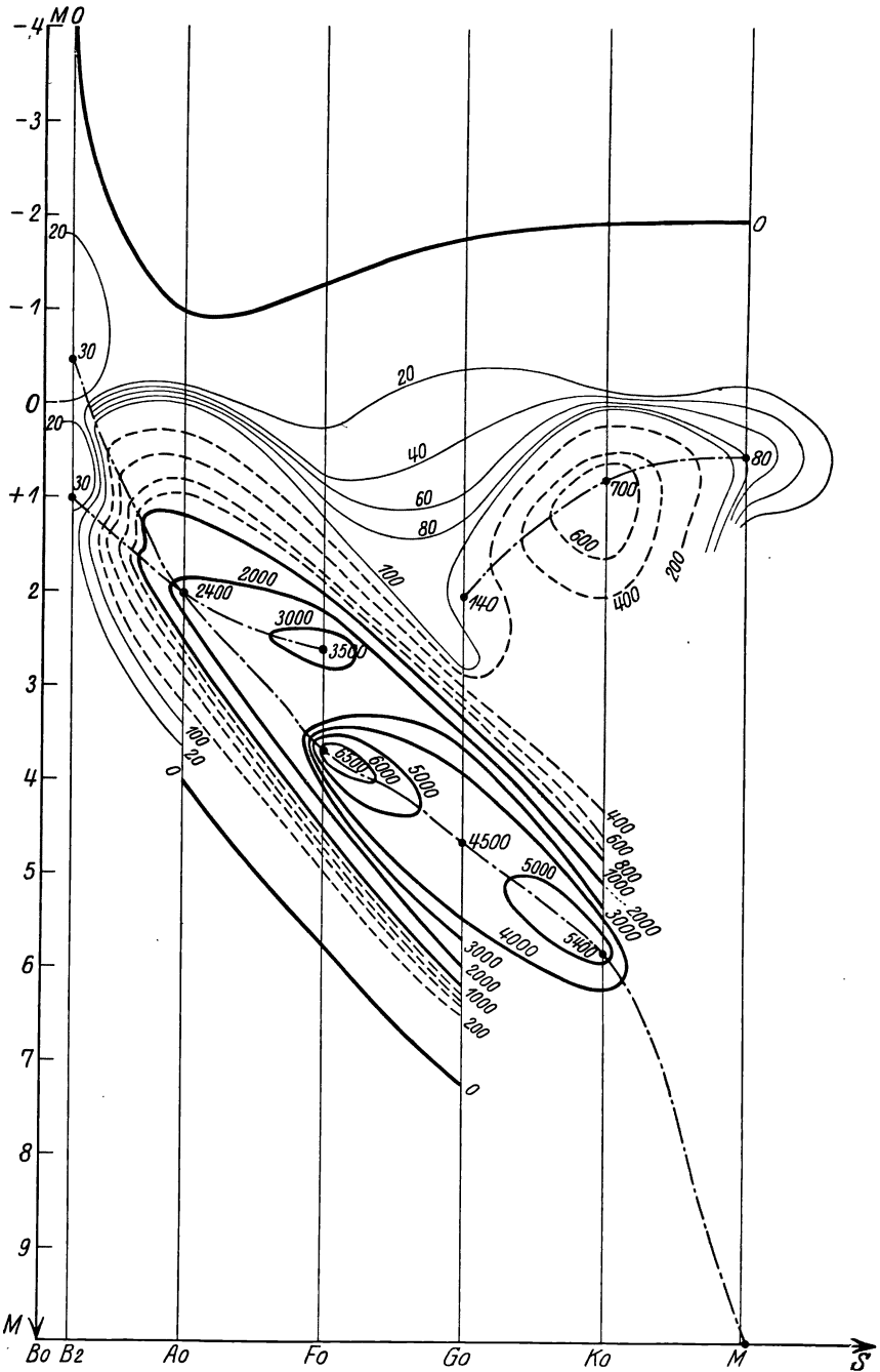
Abb. 2. Die Verteilungsfläche \Psi(M, S) der absoluten Helligkeiten und der Spektren. Die Linien parallel zur M -Achse deuten die Spektraltypen an, für die Querschnitte durch die Fläche bekannt sind. Die strichpunktierten Linien geben den Verlauf der Kammlinien der Flächen an, also der Häufigkeitsmaxima der einzelnen Spektraltypen. Die dickausgezogenen Linien sind Höhenlinien (Linien gleicher Häufigkeit von 1000 zu 1000) die gestrichelten von 200 zu 200 und die dünnausgezogenen von 20 zu 20.
