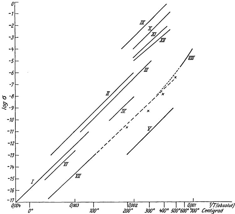
Abb. 3. Temperaturabhängigkeit der Leitfähigkeit \sigma verschiedener kristallisierter Stoffe.
