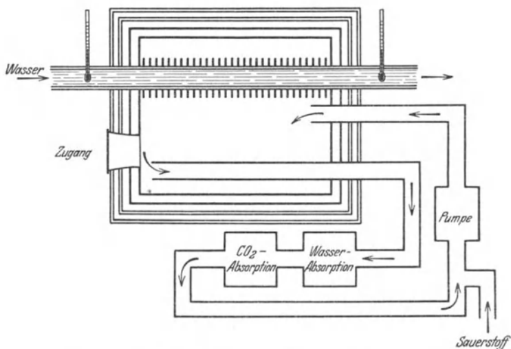
Abb. 80. Respirationkalorimeter nach ATWATER und BENEDICT.
