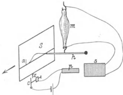
Abb. 112. Anordnung zur Aufzeichnung einer Muskelkurve. (Nach HERMANN.)
