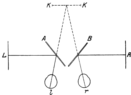
Abb. 263. WHEATSTONESCHES Spiegelstereoskop.
