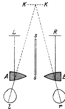
Abb. 264. BREWSTERSCHES Prismenstereoskop.
