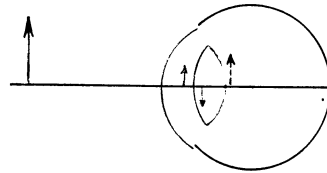
Abb. 195. Die Lage der PURKINJE-SANSONSchen Bildchen im Auge. (Nach HEINE.)
