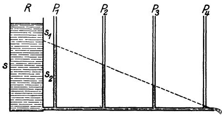
Abb. 56. Piezometer-Schema des Kreislaufsystems.
