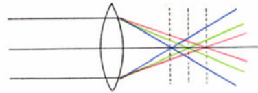
Abb. 209. Chromatische Aberration.
