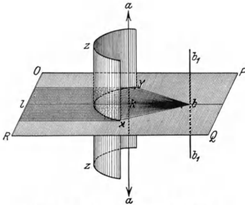
Abb. 211. Brechung an einer Zylinderfläche.
