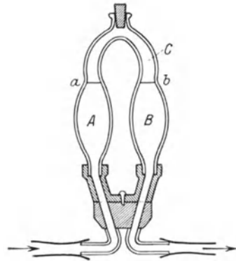
Abb. 67. Stromuhr von C. LUDWIG.
