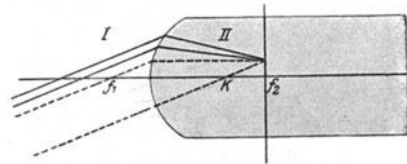
Abb. 187. Strahlengang in einem einfachen optischen System.
