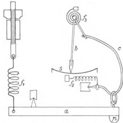
Abb. 62. Sphygmograph (Nach FRANK und PETTER.)
