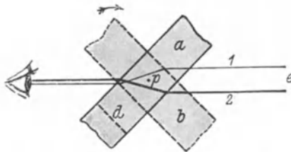
Abb. 192. Schema des Ophthalmometers von HELMHOLTZ.
