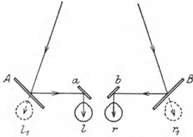
Abb. 265. Telestereoskop.
