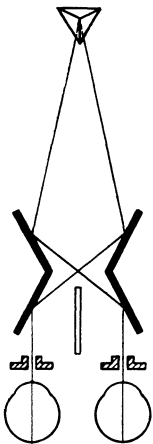
Abb. 267. Pseudoskop nach J. R. EWALD.
