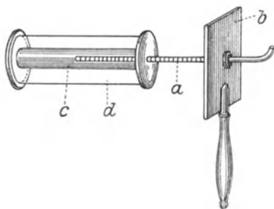
Abb. 289. Olfaktometer von ZWAARDEMAKER.
