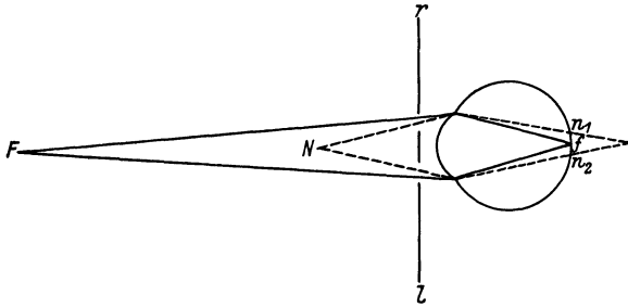
Abb. 204. Schema für den SCHEINERSchen Versuch I.
