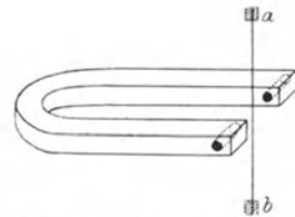
Abb. 48. Saitengalvanometer. (Schematisch.)
