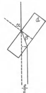
Abb. 193. Strahlenverschiebung durch eine planparallele Platte.
