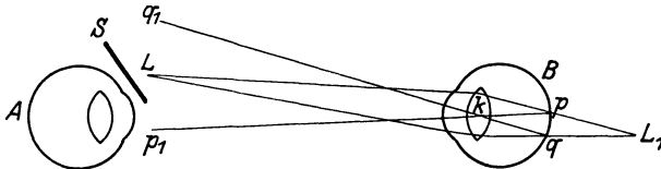
Abb. 216. BRÜCKES Versuch des Augenleuchtens.
