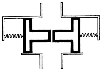
Abb. 283. Polsterpfeife nach EWALD.
