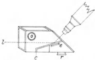
Abb. 280. Camera acustica nach EWALD.
