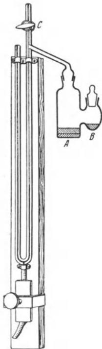
Abb. 24. Blutgasmanometer nach BARCROFT.
