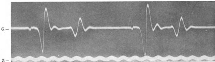
Abb. 146. Messung der Reflexzeit für die Kontraktion der Tibialismuskulatur bei induktiver Reizung des N. tibialis. (Nach P. HOFFMANN.) Zeitschreibung (Z) mit einer Stimmgabel von der Frequenz 100. G = Galvanometerkurve.
