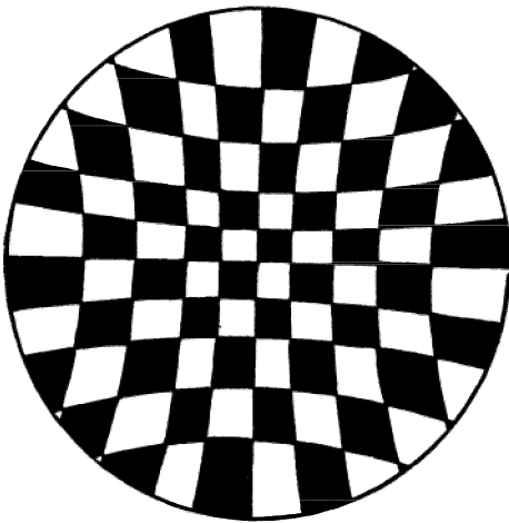
Abb. 243. HELMHOLTZsche Schachbrettfigur.
