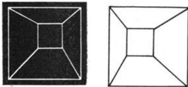
Abb. 266. Stereoskopischer Glanz.
