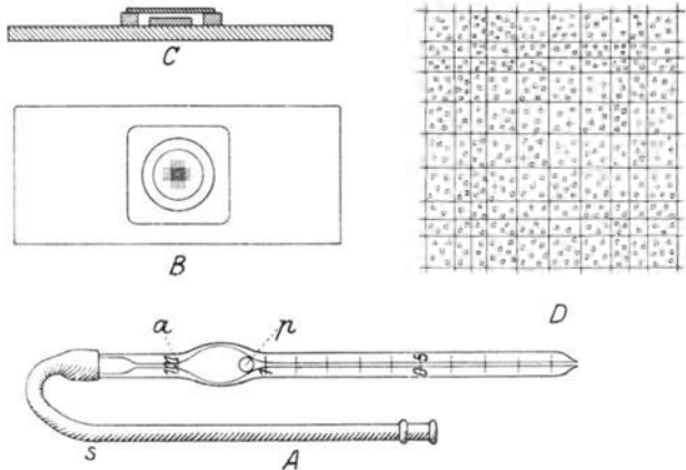
Abb. 17. Blutkörperchen-Zählapparat nach ZEISS-THOMA. A Mischpipette; B Zählkammer in der Aufsicht, ohne Deckglas; C im Längsschnitt, mit Deckglas; D Bild der gefüllten Kammer im Mikroskop.
