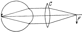
Abb. 219. Augenspiegeln im umgekehrten Bild.
