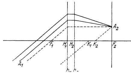
Abb. 189. Strahlengang im zentrierten optischen System.
