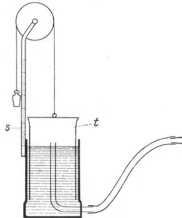
Abb. 33. Spirometer nach HUTCHINSON.
