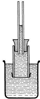
Abb. 14. Osmometer. Innerer Zylinder, unten durch eine semipermeable Membran verschlossen.
