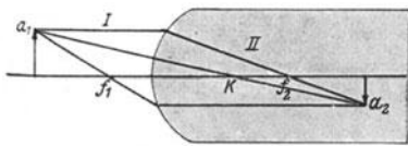
Abb. 186. Strahlengang in einem einfachen optischen System.
