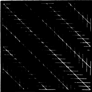
Abb. 246. ZÖLLNERSche Figur.
