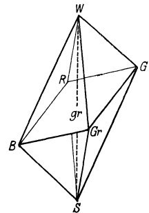
Abb. 226. Farbenkörper.
