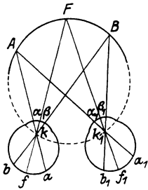
Abb. 256. Horopterkreis.
