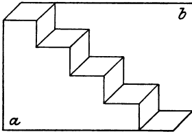
Abb. 260. SCHROEDERSche Treppe.
