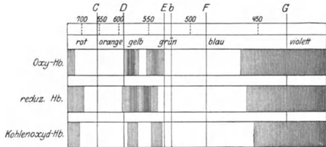
Abb. 25. Blutspektren.
