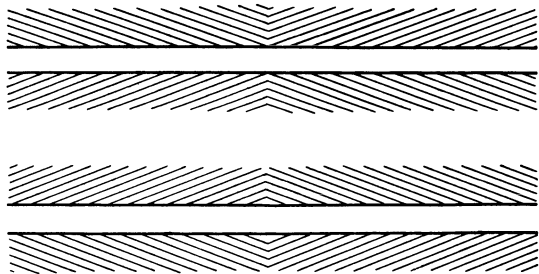
Abb. 247. HERINGSche Figur.
