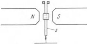
Abb. 49. Schleifenoszillograph. (Schematisch.)
