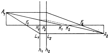
Abb. 188. Strahlengang im zentrierten optischen System.
