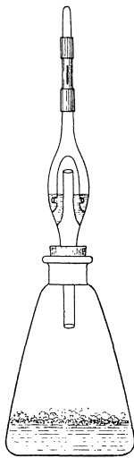
Abb. 41. Gärkolben mit dem MEISLSchen Verschluss. Im erweiterten Teil des Rohres befindet sich konzentrierte Schwefelsäure. Oben ist das Rohr mit einem Gummiventil verschlossen.
