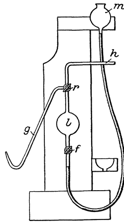
Abb. 38. Gaspipette von KOSTYTSCHEW. Erklärung im Text.
