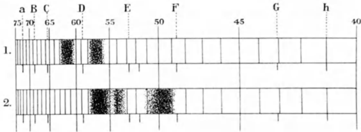
Abb. 16. 1. Absorptionsspektrum des Phycocyanins. 2. Absorptionsspektrum des Phycoerythrins.
