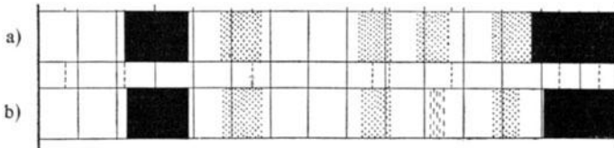
Abb. 9. a) Absorptionsspektrum der komplexen Kaliumverbindungen des Phytochlorins. b) Absorptionsspektrum des Chlorophyllins. (Nach WILSTÄTTER und STOLL.)
