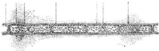
Abb. 13. Anwendung der Bakterienmethode von ENGELMANN. Die nur bei Sauerstoffzutritt beweglichen Bakterien sammeln sich am grünen Algenfaden, auf den ein prismatisches Spektrum reflektiert ist, an. Die Ansammlung der Bakterien ist nur in denjenigen Spektralbezirken sichtbar, in denen das Licht vom Chlorophyll stark absorbiert wird. (Nach ENGELMANN.)
