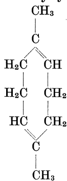
1, 5-Dimethylcyclooctadien
