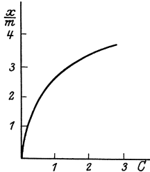
Abb. 1. Adsorptionsisotherme (nach FREUNDLICH).
