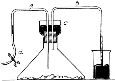
Abb. 37. Kolben von KOSTYTSCHEW. Erklärung im Text.
