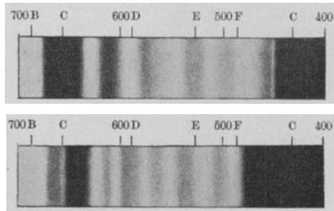
Abb. 7. Oben das Spektrum von Chlorophyll a , unten das Spektrum von Chlorophyll b . (Nach WILLSTÄTTER und STOLL.)
