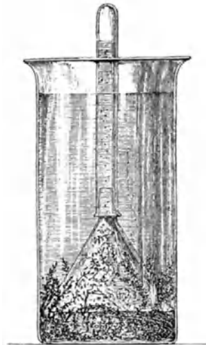
Abb. 6. Der Versuch von INGENHOUSZ. Eine belichtete Wasserpflanze scheidet sauerstoffreiche Gasbläschen aus. (Nach PALLADIN.)
