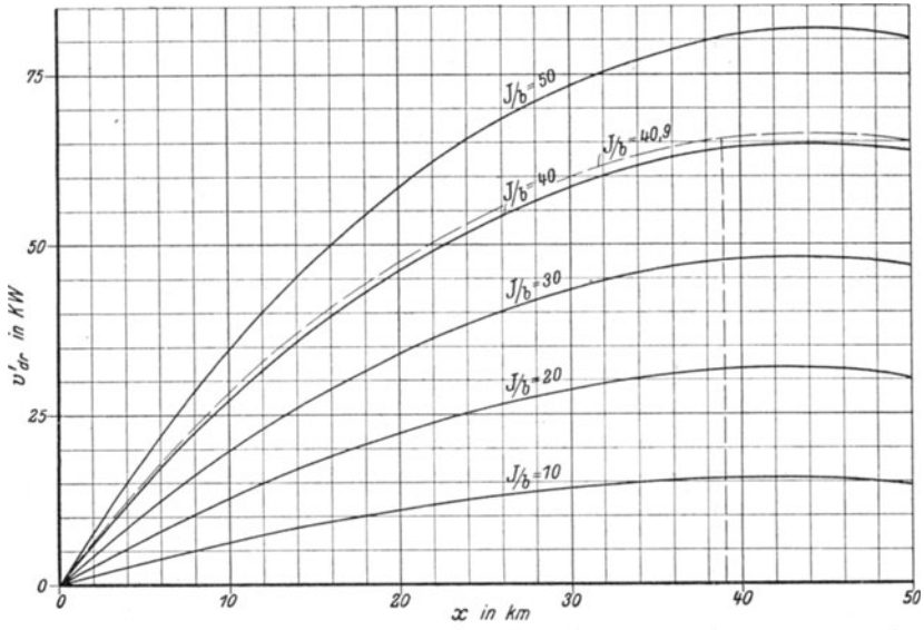
Fig. 52. Vergrößerung der Leitungsverluste bei einer Gesamtleitungslänge von L = 50 km.
