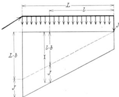
Fig. 15. Gleichmäßige Belastung der Leitung und Großkonsument am Ende der Leitung.
