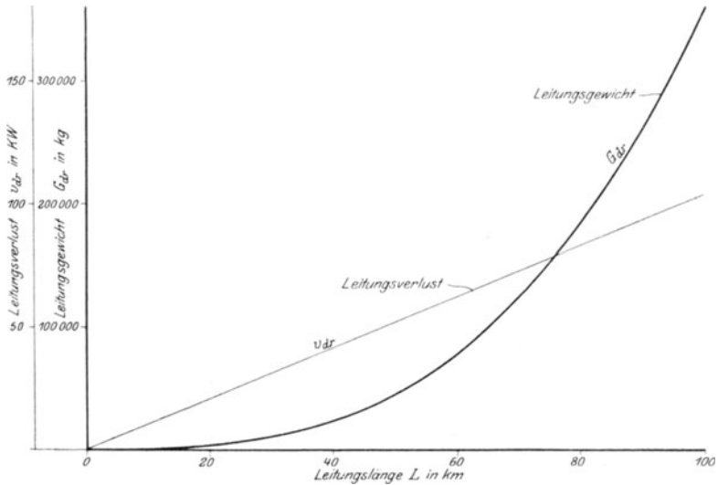
Fig. 14. Leitungsgewichte und Verluste für Drehstromkraftübertragung mit Kupferleitungen bei gleichmäßiger Belastung der Strecke mit b = 1 Amp./km und einem maximalen Spannungsabfall von e_{dr} = 1000 Volt am Ende der Leitung. (Nach Tabelle V.)
