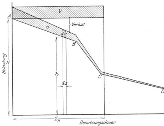
Fig. 4. Verluste durch Stromwärme in den Leitungen.
