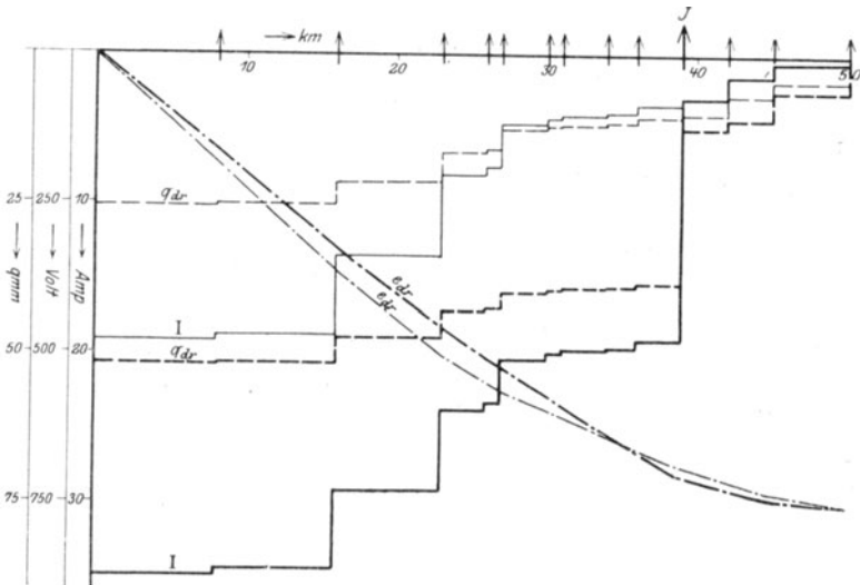
Fig. 12. Günstigste Querschnittsbemessung vor und nach dem Anschluß des Großabnehmers. (Nach den Tabellen III und IV.)
