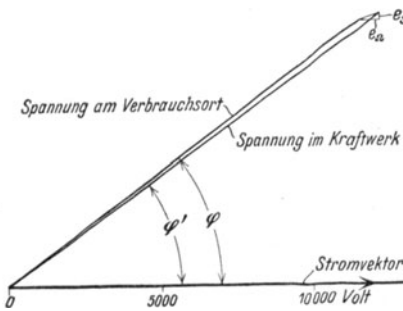
Fig. 5. Spannungsdiagramm der Hochspannungsfreileitung einer Überlandzentrale.
