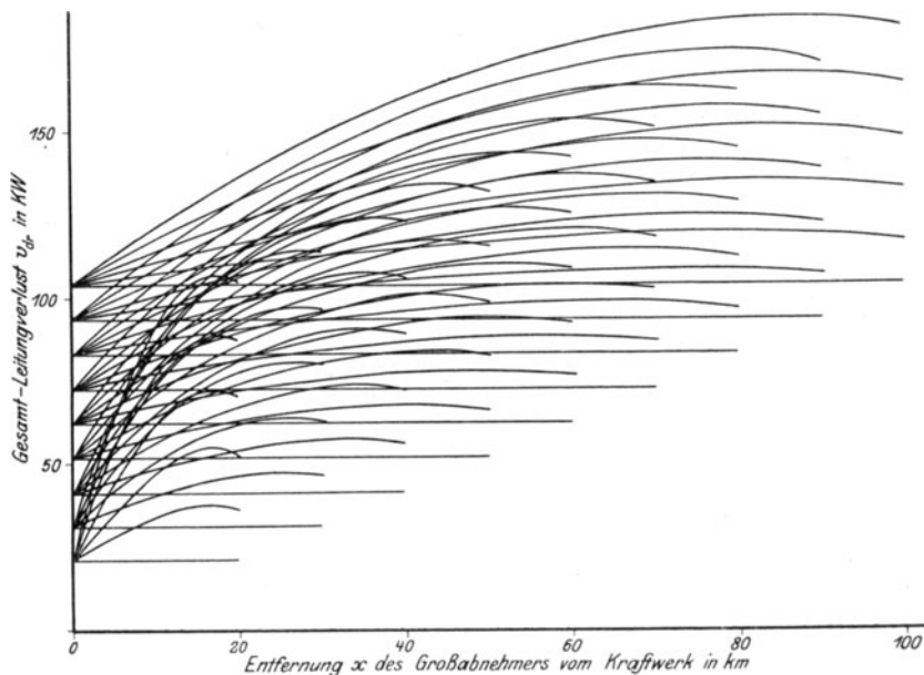
Fig. 19. Leitungsverluste für Drehstromkraftübertragung mit Kupferleitungen bei gleichmäßiger Belastung der Strecke mit b = 1 Amp/km und Belastung durch einen Großkonsumenten mit J Amp. in der Entfernung x vom Kraftwerk bei einem maximalen Spannungsabfall von e_{dr} = 1000 Volt am Ende der Leitung. (Nach Tabelle VIII.)
