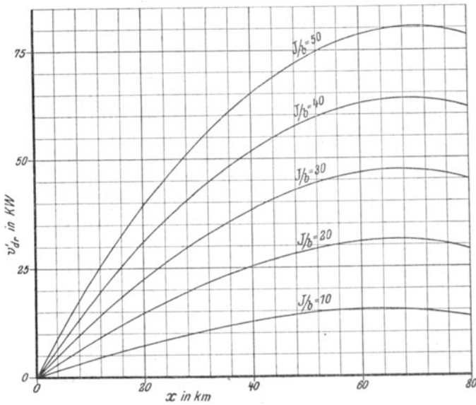
Fig. 49. Vergrößerung der Leitungsverluste bei einer Gesamtleitungslänge von L = 80 km.
