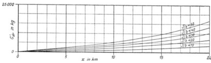
Fig. 46. Mehrbedarf an Leitungsgewicht bei einer Gesamtleitungslänge von L = 20 km.
