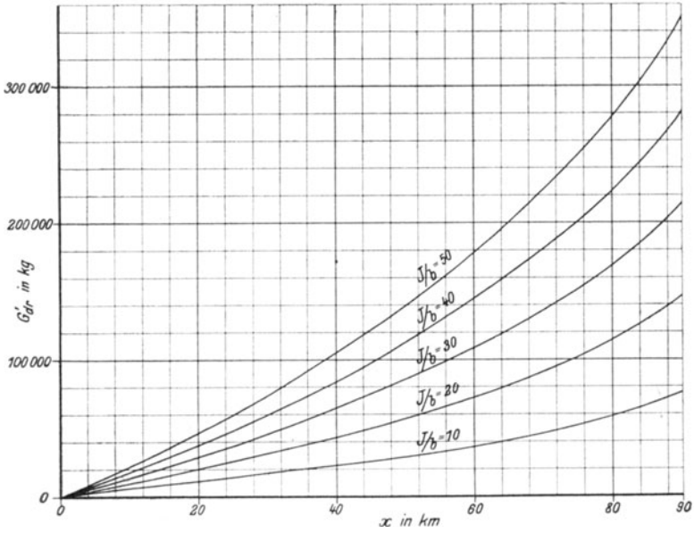
Fig. 39. Mehrbedarf an Leitungsgewicht bei einer Gesamtleitungslänge von L = 90 km.
