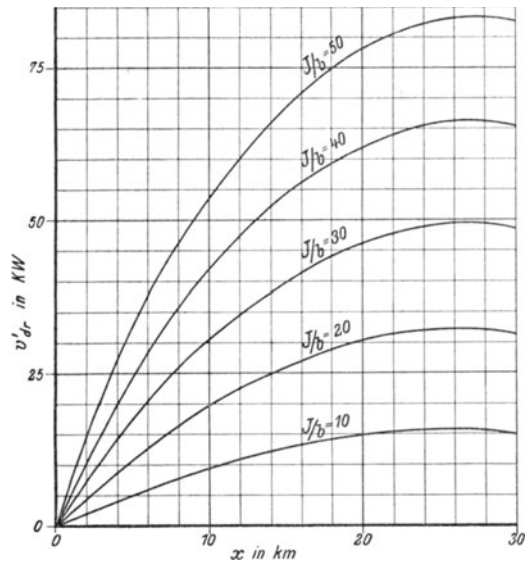
Fig. 54. Vergrößerung der Leitungsverluste bei einer Gesamtleitungslänge von L = 30 km.
