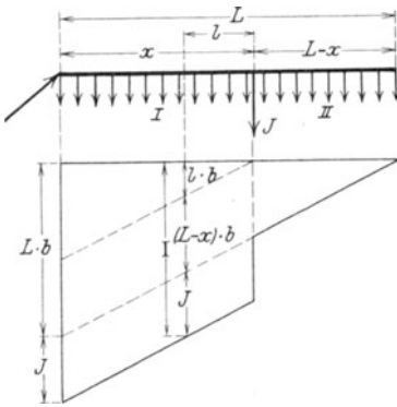
Fig. 17. Gleichmäßige Belastung der Leitung und Großkonsument an einer beliebigen Stelle der Leitung.
