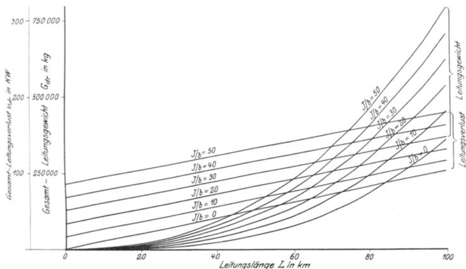
Fig. 16. Leitungsgewichte und Verluste für Drehstromkraftübertragung mit Kupferleitungen bei gleichmäßiger Grundbelastung der Strecke mit b = 1 Amp/km und Belastung durch einen Großkonsumenten am Ende der Leitung mit J Amp. bei einem maximalen Spannungsabfall von v_{dr} = 1000 Volt am Ende der Leitung. (Nach Tabelle VI.)
