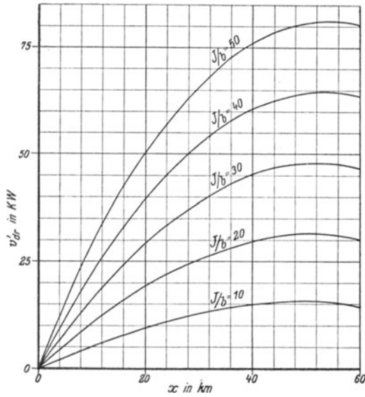
Fig. 51. Vergrößerung der Leitungsverluste bei einer Gesamtleitungslänge von L = 60 km.
