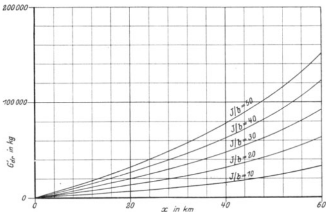
Fig. 42. Mehrbedarf an Leitungsgewicht bei einer Gesamtleitungslänge von L = 60 km.
