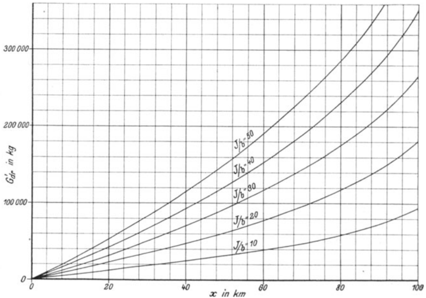
Fig. 38. Mehrbedarf an Leitungsgewicht bei einer Gesamtleitungslänge von L = 100 km.
