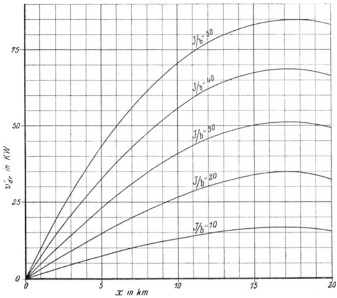
Fig. 55. Vergrößerung der Leitungsverluste bei einer Gesamtleitungslänge von L = 20 km.
