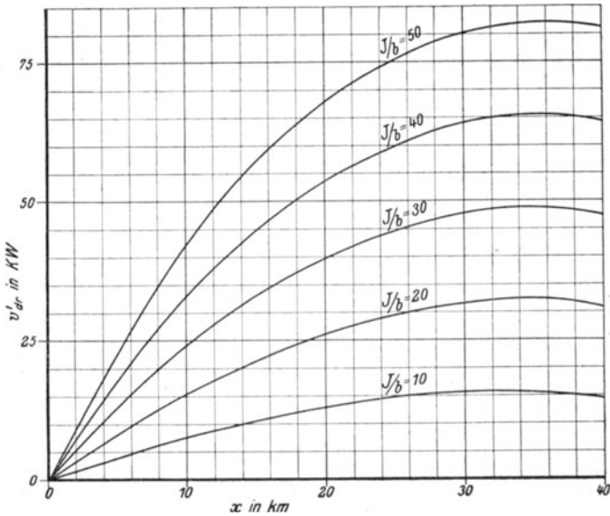
Fig. 53. Vergrößerung der Leitungsverluste bei einer Gesamtleitungslänge von L = 40 km.
