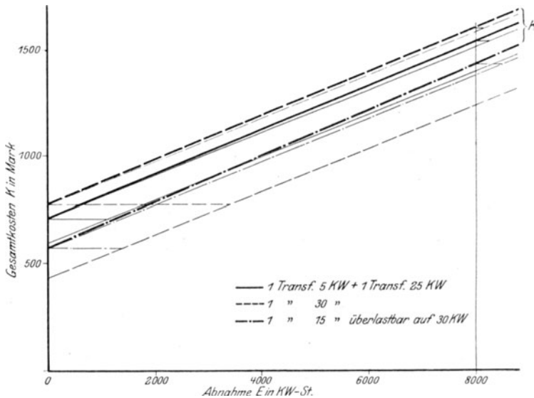
Fig. 9. Selbstkosten des Großabnehmers für verschiedene Transformatoren.
