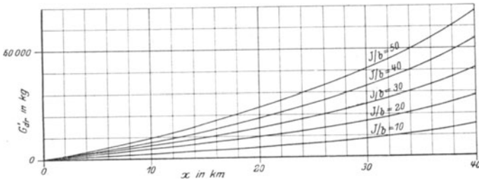
Fig. 44. Mehrbedarf an Leitungsgewicht bei einer Gesamtleitungslänge von L = 40 km.
