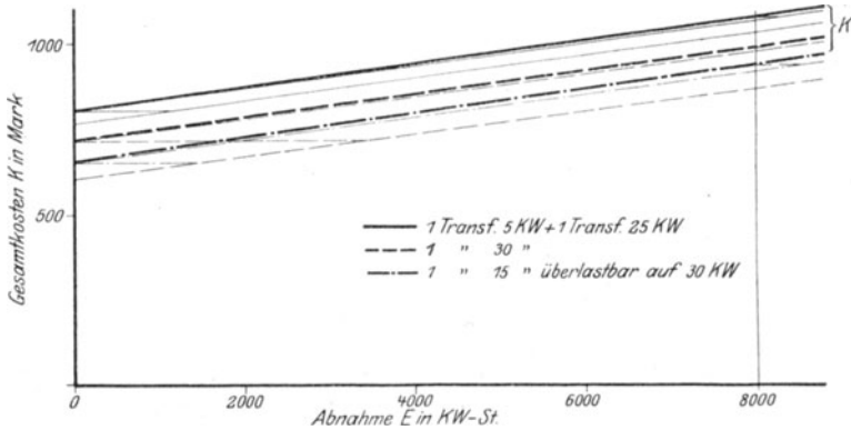
Fig. 8. Selbstkosten der Überlandzentrale für verschiedene Transformatoren.
