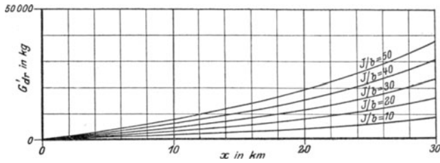
Fig. 45. Mehrbedarf an Leitungsgewicht bei einer Gesamtleitungslänge von L = 30 km.
