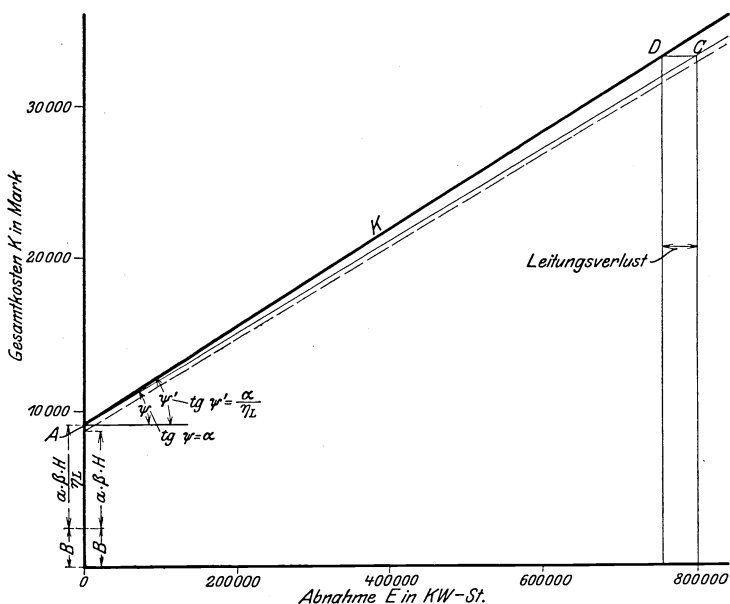
Fig. 6. Selbstkosten am Ende einer besonderen Zuleitung.
