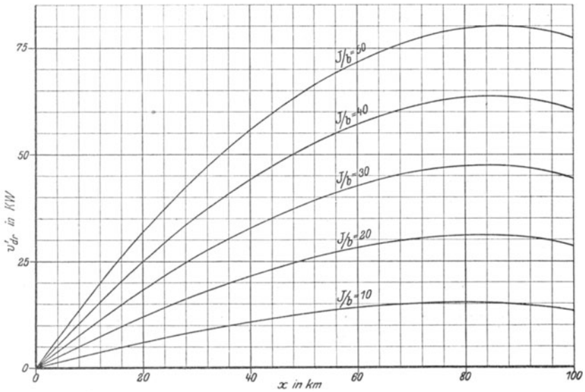
Fig. 47. Vergrößerung der Leitungsverluste bei einer Gesamtleitungslänge von L = 100 km.
