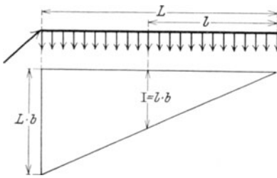
Fig. 13. Gleichmäßige Belastung der Leitungsstrecke.
