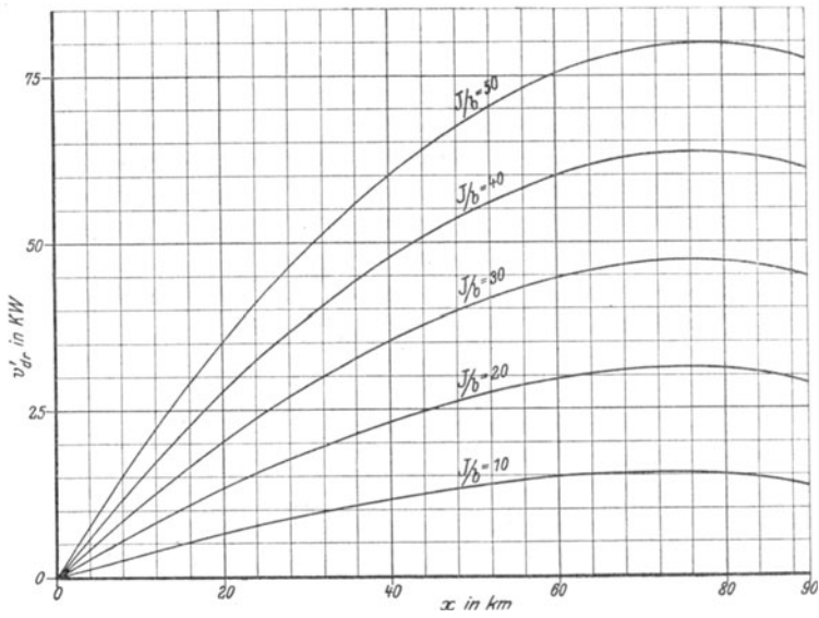
Fig. 48. Vergrößerung der Leitungsverluste bei einer Gesamtleitungslänge von L = 90 km.
