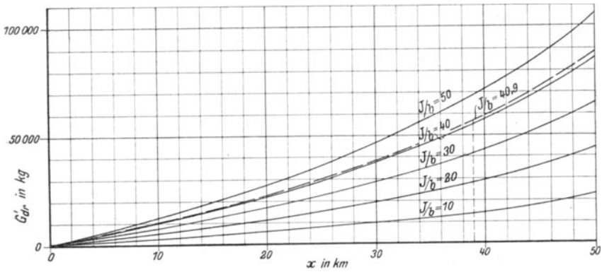
Fig. 43. Mehrbedarf an Leitungsgewicht bei einer Gesamtleitungslänge von L = 50 km.
