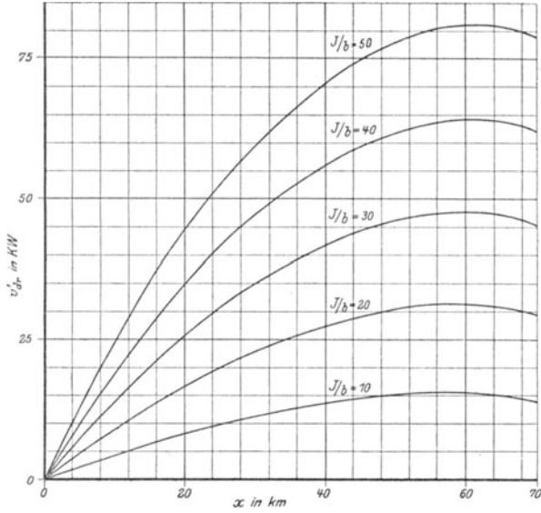
Fig. 50. Vergrößerung der Leitungsverluste bei einer Gesamtleitungslänge von L = 70 km.
