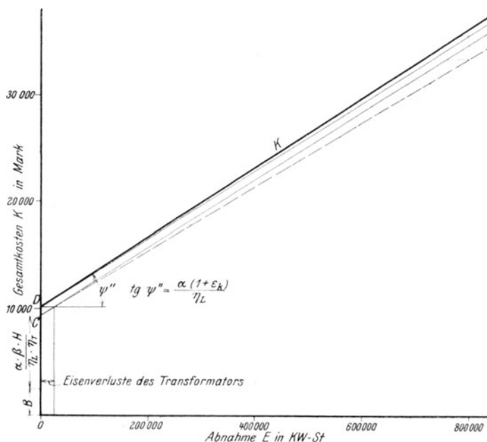
Fig. 7. Selbstkosten hinter dem Transformator.
