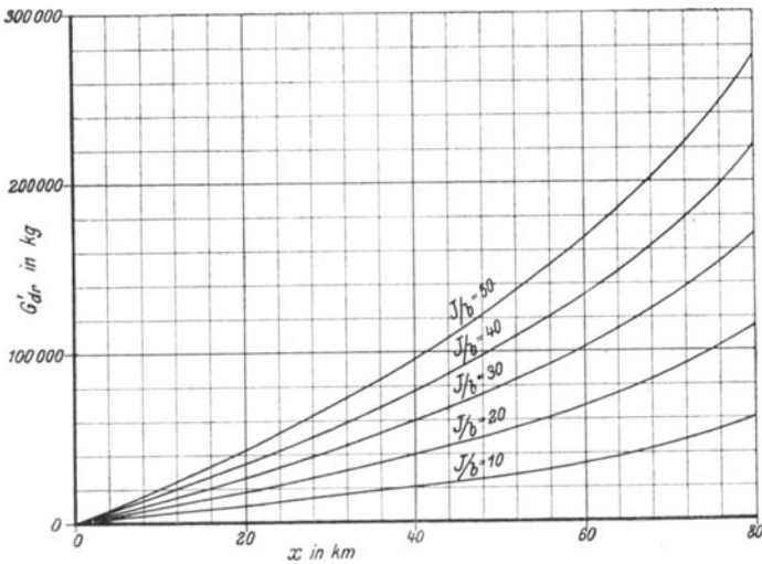
Fig. 40. Mehrbedarf an Leitungsgewicht bei einer Gesamtleitungslänge von L = 80 km.
