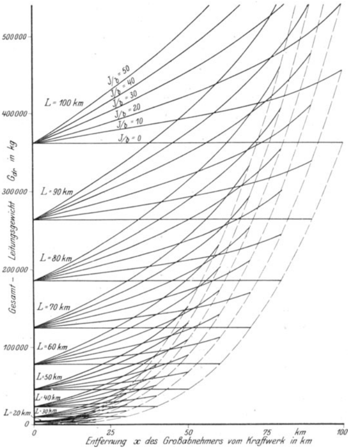
Fig. 18. Leitungsgewichte für Drehstromkraftübertragung mit Kupferleitungen bei gleichmäßiger Belastung der Strecke mit b = 1 Amp/km und Belastung durch einen Großkonsumenten mit J Amp. in der Entfernung x vom Kraftwerk bei einem maximalen Spannungsabfall von e_{dr} = 1000 Volt am Ende der Leitung. (Nach Tabelle VII.)
