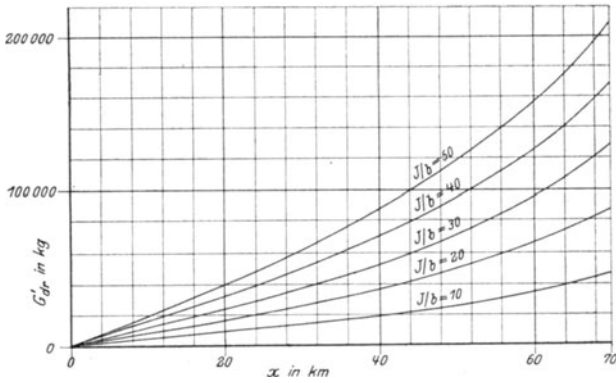
Fig. 41. Mehrbedarf an Leitungsgewicht bei einer Gesamtleitungslänge von L = 70 km.
