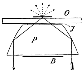
Abb. 4. Strahlengang im Paraboloidkondensator zur Dunkelfelduntersuchung.
