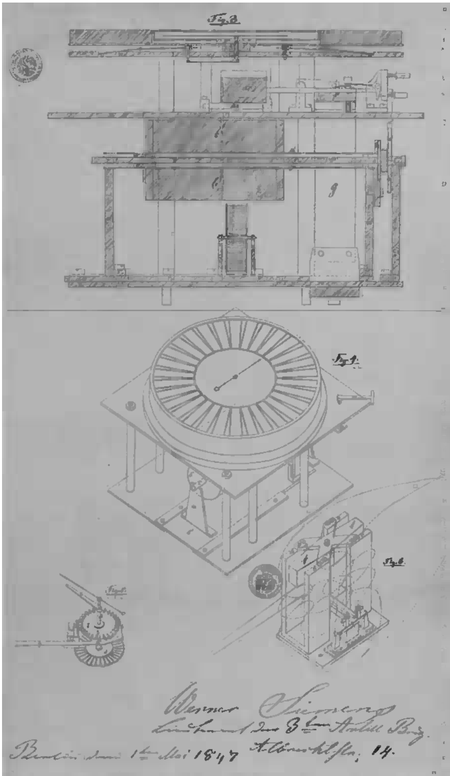
Saksimile und verkleinerte Original-Zeichnung aus der Patentschrift über den Zeigertelegraphen.
