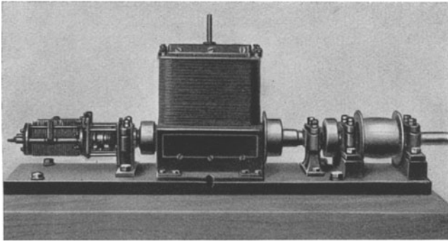
Original einer der ältesten dynamo-elektrischen Maschinen von Werner von Siemens. 1868.
