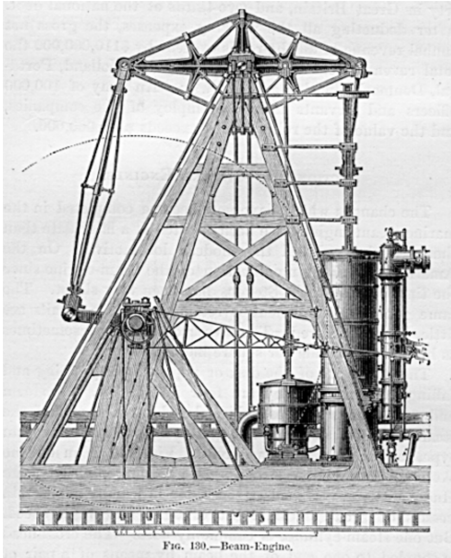
Fig. 130.-Beam-Engine.
