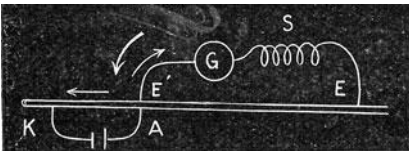
Abb. 31. Versuchsanordnung zur Demonstration der deprimierenden Wirkung der Kathode (oben), der erregenden der Anode (unten). Der dünne Pfeil zeigt die Richtung des elektrotonischen, der dicke die des Aktionsstromes an. Nach Bose, Comparative Electrophysiology .
