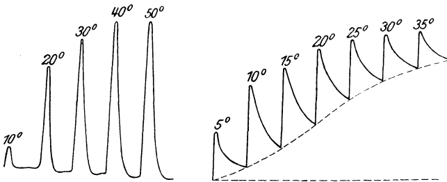
Abb. 24. Kurven der EMK des Aktionsstromes bei Reizung mit Torsion um zunehmende Winkelgrade. Blumenkohlstiel. Nach Bose, Comp. Electrophys.
