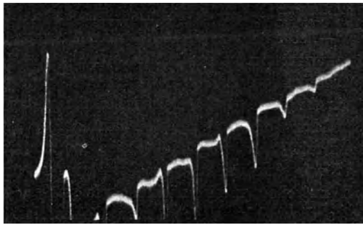
Abb. 26. Übergang von galv. Positivität in Negativität an einem gewelkten Blattstiel des Blumenkohls. Die Kurve ist von rechts nach links zu lesen. Die Ausschläge nach unten bedeuten Positivität, die nach oben Negativität. Nach Bose, Comp. Electrophys.
