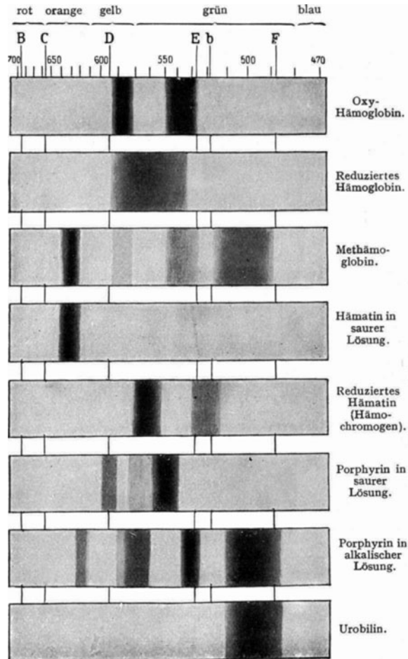
Abb. 59. Spektraltafel.
