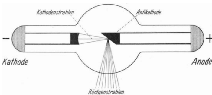
Abb. 1. Röntgenröhre.
