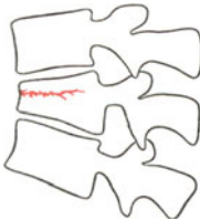
Abb. 6. Kompressionsfraktur eines Wirbels im seitlichen Bild.
