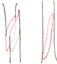
Abb. 4. Bruchlinien der Torsionsfraktur.
