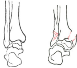
Abb. 9. Typische Malleolarfraktur: Rißbruch am medialen, Biegungsbruch am lateralen Knöchel.
