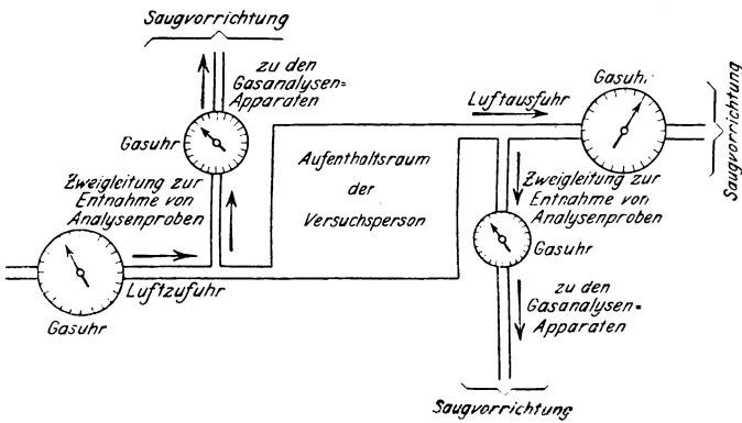
Fig. 11. Apparat zur Bestimmung des Gasstoffwechsels.
