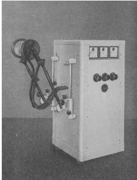
Abb. 45. Kurzwellenapparat für 1 m Wellenlänge und 700 Watt Leistung (Siemens-Reiniger-Werke).
