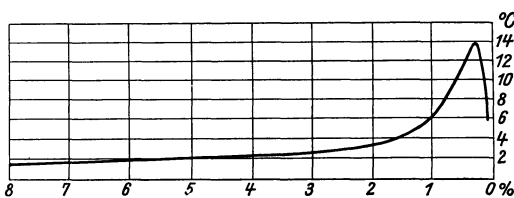
Abb. 79. Erwärmung verschieden konzentrierter Kochsalzlösungen im Felde einer 5 m-Welle.
