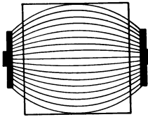
Abb. 55. Der Querschnitt der Elektroden ist kleiner als der des Behandlungsobjektes. Tiefenwirkung kleiner als 100%.
