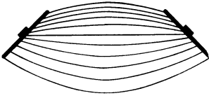
Abb. 61. Feldlinienverlauf bei geneigten Elektroden.
