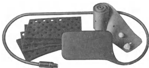
Abb. 49. Weichgummielektrode mit Filzunterlagen und Befestigungsbinde (Siemens-Reiniger-Werke).
