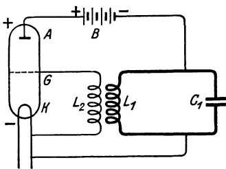
Abb. 40. Die Dreielektrodenröhre als Schwingungserreger.
