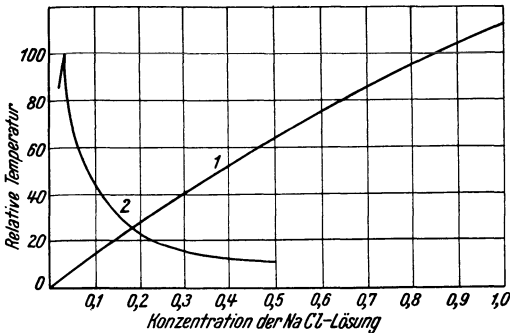
Abb. 71. Erwärmung einer Kochsalzlösung im magnetischen (1) und im elektrischem (2) Feld.
