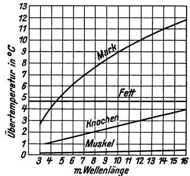
Abb. 81. Einfluß der Wellenlänge auf die Erwärmung verschiedener Gewebe nach Gebbert.
