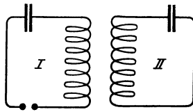
Abb. 27. Induktive Koppelung.
