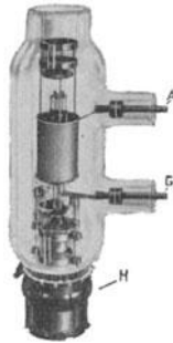
Abb. 38. Ansicht einer Elektronenröhre (Siemens-Keiniger-Werke).
