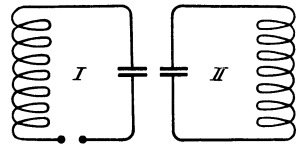
Abb. 28. Kapazitive Koppelung.
