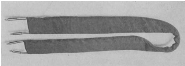
Abb. 134. Schleifenelektrode zur Hyperthermiebehandlung (Sanitas).
