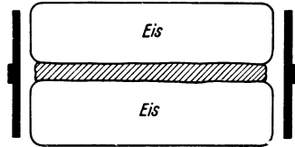
Abb. 83. Rohes Fleisch zwischen zwei Eisblöcken wird verkocht, ohne daß das Eis schmilzt.
