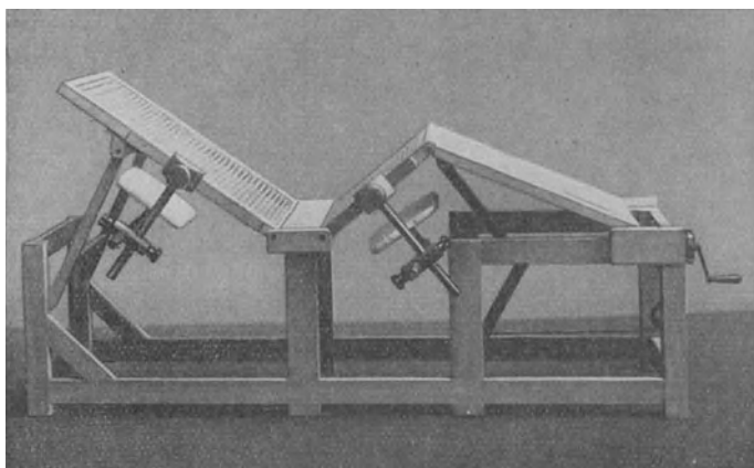
Abb. 70. Verstellbarer Behandlungstisch mit Untertischelektroden (Siemens-Reiniger-Werke).
