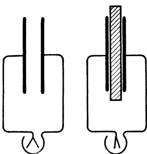
Abb. 6. Die Luft zwischen den Kondensatorplatten wird durch eine Glasscheibe ersetzt. Die Spannung sinkt.
