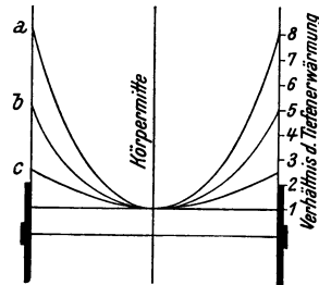
Abb. 64. Elektrodenabstand und Tiefenwirkung: a anliegende Elektroden; b 10 mm Luftabstand; c 20 mm Luftabstand (nach Pätzold und Betz).
