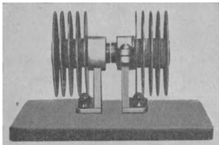
Abb. 32. Löschfunkenstrecke.
