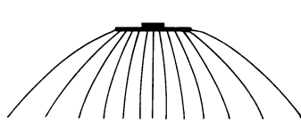
Abb. 60. Feldlinienverlauf bei der unipolaren Behandlung.
