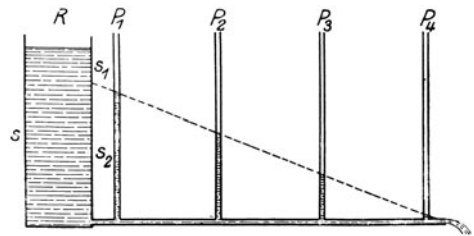
Abb. 54. Piezometer-Schema des Kreislaufsystems.
