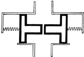
Abb. 274. Polsterpfeife nach EWALD.
