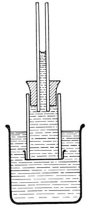
Abb. 14. Osmometer. Innerer Zylinder, unten durch eine semipermeable Membran ver- schlossen.
