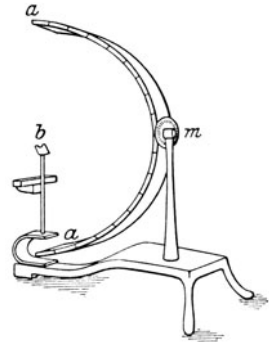
Abb. 229. Perimeter nach FOERSTER.
