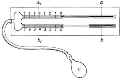
Abb. 71. Viskosimeter nach W. R. HESS.
