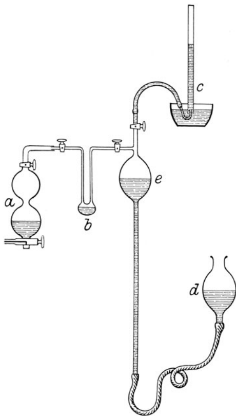
Abb. 23. Quecksilberpumpe. a Blutrezipient; b Gefäß mit konzentrierter Schwefelsäure zur Absorption von Wasserdampf; c Quecksilberwanne mit Eudiometerrohr. Durch abwechselndes Senken und Heben der Quecksilberfüllkugel d kann die anfänglich in a und b enthaltene Luft abgesogen und nach der Quecksilberwanne hinausgetrieben werden. Sind a und b völlig evakuiert, so wird der untere Hahn von a mit einem Blutgefäß verbunden, und durch Drehung des Hahns das Blut direkt aus dem Tier in a einströmen gelassen; das Blut kocht schäumend in den Kugeln von a in die Höhe. Darauf werden die Blutgase durch mehrmaliges Senken und Heben von d in das Eudiometer über der Quecksilberwanne befördert.
