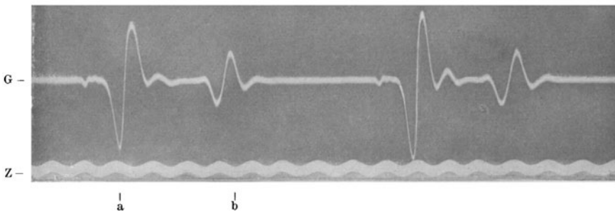
Abb. 139. Messung der Reflexzeit für die Kontraktion der Tibialismuskulatur bei induktiver Reizung des N. tibialis. (Nach P. HOFFMANN.) Zeitschreibung (Z) mit einer Stimmgabel von der Frequenz 100. G = Galvanometerkurve.
