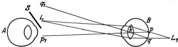
Abb. 207. BRÜCKES Versuch des Augenleuchtens.
