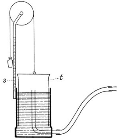
Abb. 33. Spirometer nach HUTCHINSON.
