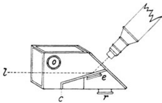
Abb. 271. Camera acustica nach EWALD.
