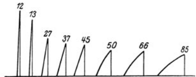
Abb. 127. „Dreieckige“ Stromstöße, bei denen die physiologische Wirkung gleich, die bewegte Elektrizitätsmenge sehr verschieden groß ist. (Nach GILDEMEISTER.)
