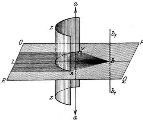
Abb. 202. Brechung an einer Zylinderfläche.
