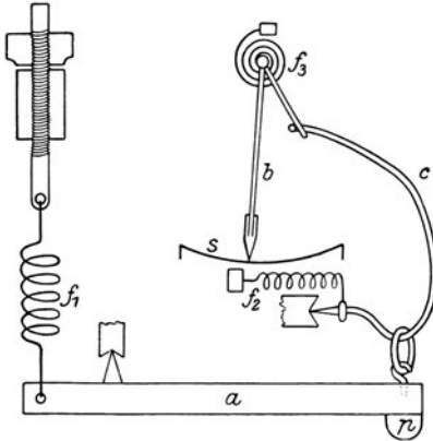
Abb. 60. Sphygmograph (Nach FRANK und PETTER.)
