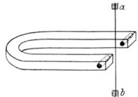
Abb. 48. Saitengalvanometer. (Schematisch.)
