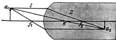
Abb. 177. Strahlengang in einem einfachen optischen System.
