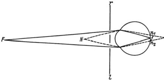
Abb. 195. Schema für den SCHEINERSchen Versuch I.
