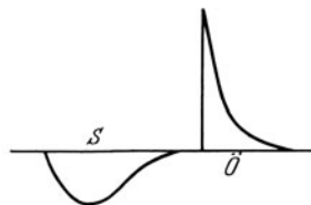
Abb. 128. Verlauf des Schließungs- und Öffnungsinduktionsstroms in der Sekundärspule. Die Flächen, d. h. die bewegten Elektrizitätsmengen, sind gleich groß.
