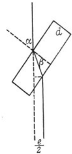
Abb. 184. Strahlenverschiebung durch eine planparallele Platte.
