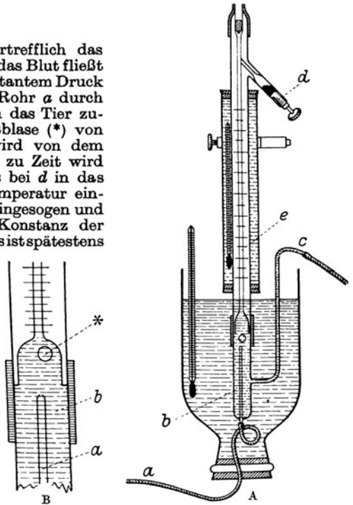
Abb. 30. Mikrotonometer von KROGH.
