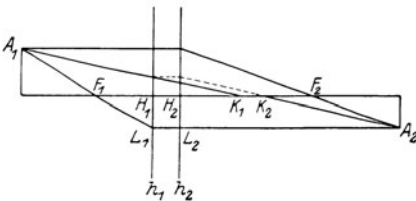
Abb. 179. Strahlengang im zentrierten optischen System.
