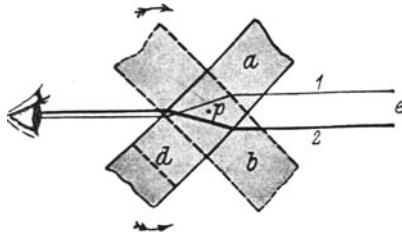
Abb. 183. Schema des Ophthalmometers von HELMHOLTZ.
