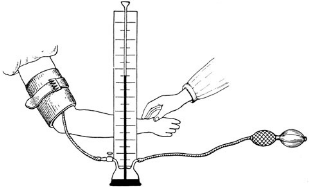
Abb. 59. Sphygmomanometer von RIVA-ROCCI.
