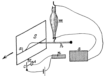
Abb. 106. Anordnung zur Aufzeichnung einer Muskelkurve. (Nach HERMANN.)
