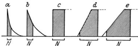
Abb. 126. Abhängigkeit der Nutzzeit (N) von der Stromform. (Nach GILDEMEISTER.)
