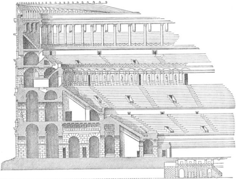
Fig. 3. Amphitheatrum Flavium im Längendurchschnitt (nach Schreiber).
