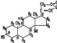
a Digitoxigenin
