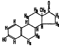
e Follikelhormon
