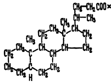
b Cholansäure
