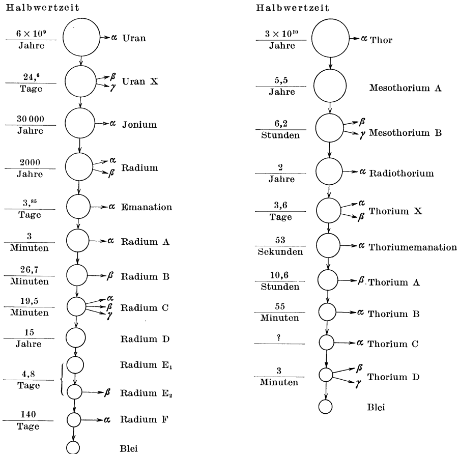
Abb. 105. Umwandlungsreihe von Uran und Thorium.
