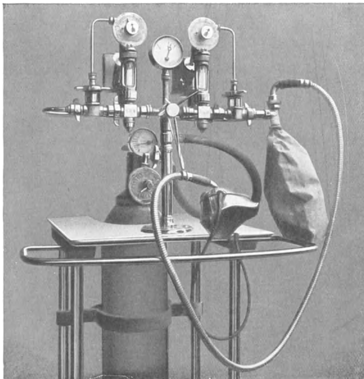
Abb. 84. Narkoseapparat nach Roth-Dräger-Krönig.
