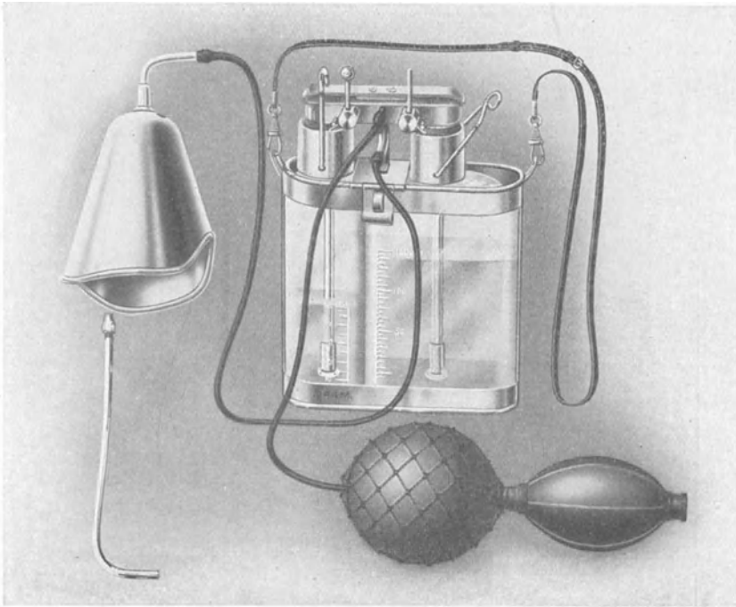
Abb. 83. Braunscher Apparat.
