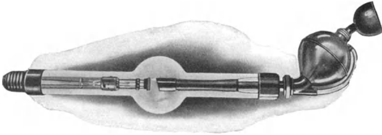
Abb. 8. Coolidge-Diagnostikröhre (C. H. F. Müller) mit Wasserkühlung. Links die Glühkathode, rechts die Antikathode.
