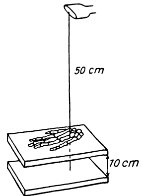
Abb. 69. Durch die in der Abb. gegebene Anordnung kann die Zeichenschärfe eines Brennflecks geprüft werden.
