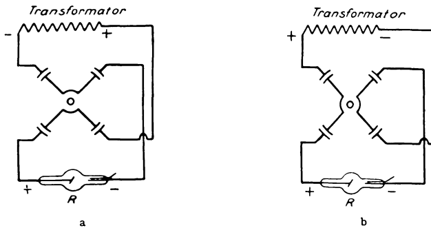
Abb. 26 a und b. Die Funktion des Hochspannungsgleichrichters.
