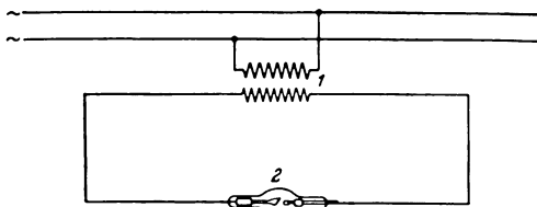
Abb. 30. Halbwellenapparat ohne Hochspannungsventil. Die Röntgenröhre sperrt selbst die negativen Phasen. 1 = Transformator, 2 = Röntgenröhre.
