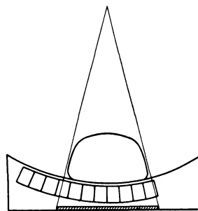
Abb. 76. Die Zylinderblende.
