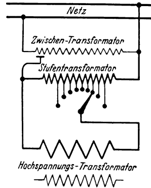
Abb. 21. Ergänzung der Grobregulierung durch den Zwischentransformator (Feinregulierung).
