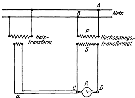
Abb. 18. Anlage einer Röntgenapparatur.
