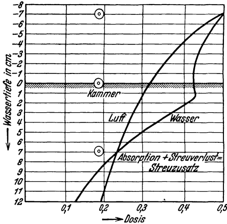
Abb. 290. Verlauf der Dosiskurve in Luft und in Wasser (nach JÄGER und RUMP). Man beachte den Knick der Kurve unterhalb der Wasseroberfläche.
