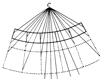
Abb. 73. Die Abschirmung der von C ausgehenden Streustrahlung ist eine um so vollständigere, je tiefer die Lamellen der Blende sind.
