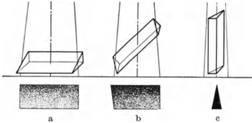
Abb. 91. Die Projektion des Keiles im Zentralstrahl.
