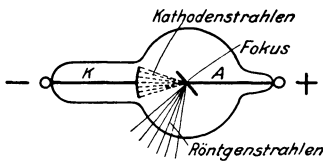
Abb. 6. Primitives Modell einer Röntgenröhre.
