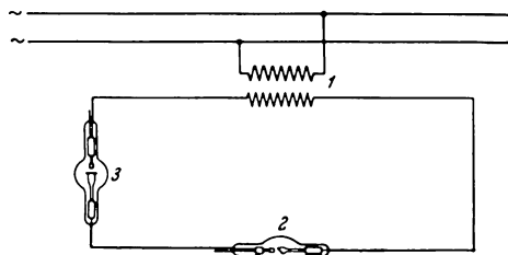
Abb. 31. Halbwellenapparat mit Ventilröhre. Das in Serie geschaltete Ventilrohr sperrt die negativen Phasen des Transformators. 1 = Transformator, 2 = Röntgenröhre, 3 = Ventilrohr.
