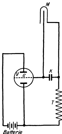
Abb. 301. Das Meka- pion von S. STRAUSS.
