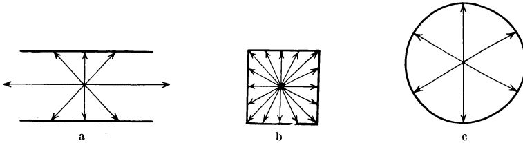
Abb. 74. Einfluß der Form und Anordnung der Lamellen auf die Abschirmung der Streustrahlung. In Anordnung a wird der Teil der Streustrahlung, der parallel zu den Lamellen verläuft, nicht abgeschirmt. Am gleichmäßigsten ist die Wirkung auf die Streustrahlung bei der Kreisform c.
