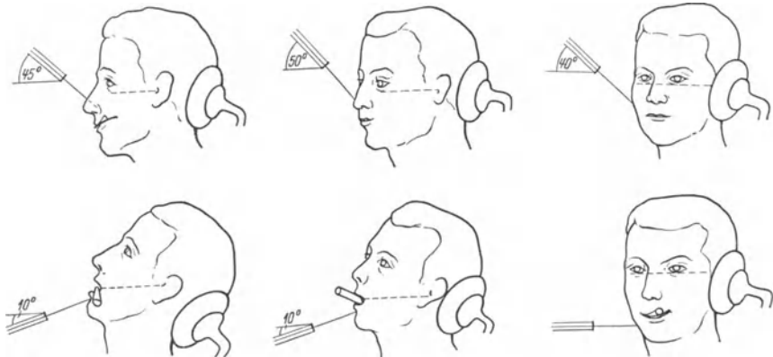
Abb. 120. Schema zur Einstellung der Zähne des Oberkiefers (obere Reihe) und des Unterkiefers (untere Reihe). Die erste Stellung zeigt die Aufnahme der Frontzähne, die zweite die des Eckzahns und der Prämolaren, die dritte die der Molaren. Die äußere Orientierung des Kopfes geschieht nach Linien, die parallel zur Bißebene verlaufen, also für den Oberkiefer nach der deutschen Horizontalen, für den Unterkiefer in der Gegend der Front- und Eckzähne nach einer Linie, die vom Mundwinkel zum äußeren Gehörgang zieht. (Berichtigung: erstes Bild lies 55^{\circ} .)
