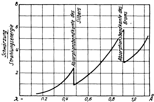
Abb. 63. Schwärzung einer photographischen Platte in Abhängigkeit von der Wellenlänge der Strahlung bei gleicher einfallender Strahlungsenergie (nach GLOCKER).
