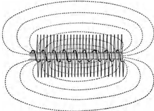
Abb. 15. Transformatorspule mit Kraftfeld.
