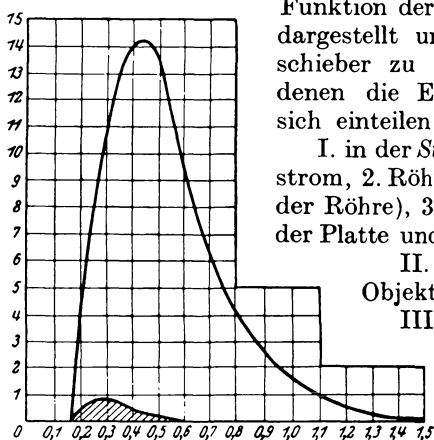
Abb. 65. Der Flächeninhalt der schraffierten Kurve gibt denjenigen Teil einer bei 75 kV erzeugten Strahlung an, der nach Durchtritt durch eine 10 cm dicke Gewebeschicht der Absorption entgeht und auf die photographische Platte einwirken kann. (Nach H. KÜSTNER.)
