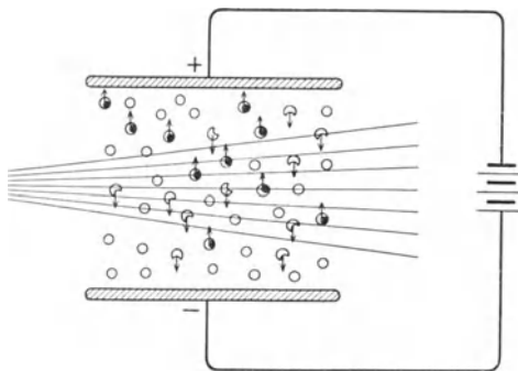
Abb. 54. Der Ionisationsstrom. ○ = neutrales Gasmolekül; • = Elektron; ⊕ = positiver Elektrizitätsträger; ⊖ = negativer Elektrizitätsträger.
