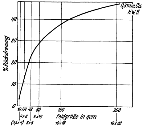
Abb. 288. Größe der Rückstreuung an der Einfallsfläche der Strahlung, in Prozenten der Primärstrahlung in Abhängigkeit von der Feldgröße, gültig für eine Strahlung von 2—1,5 mm Cu HWS (in der Abb. irrtümlich 0,3 mm Cu).
