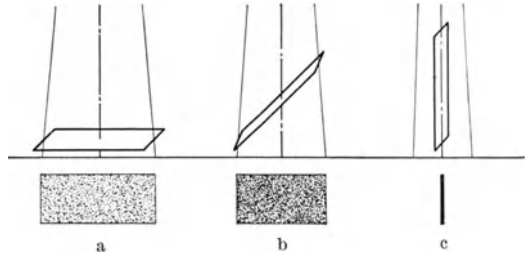
Abb. 90. Die Projektion eines flächenhaften Gebildes im Zentralstrahl.
