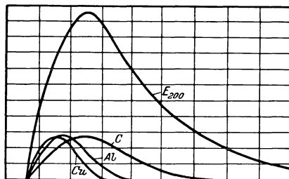
Abb. 286. Spezifische Wirkung des Filtermaterials. Eine bei 200 kV erzeugte Strahlung E_{200} wird mit 44 mm Kohlenstoff, 17,5 mm Aluminium und 1 mm Kupfer gefiltert. Die Kurven C, Al und Cu zeigen die Schwächung und Einengung des Strahlenspektrums durch Kohlenstoff (C), bzw. Aluminium (Al), bzw. Kupfer (Cu). (Nach G. GROSSMANN: Physikalische und technische Grundlagen der Röntgentherapie.)
