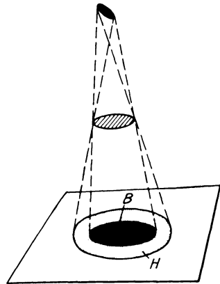
Abb. 61. Eine flächenhafte Strahlenquelle führt zu Schlagschatten- ( B ) und Halbschattenbildung ( H ).
