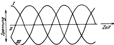
Abb. 33. Strombild des Dreiphasendrehstroms. I, II und III = die um 120 elektrische Grade verschobenen Wechselstromphasen.
