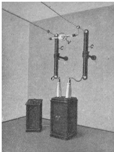
Abb. 39. Halbwellen-Kondensatorapparat (Siemens-Reiniger-Veifa).
