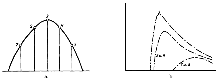
Abb. 45a u. b. Abhängigkeit der Strahlenemission einer Röntgenröhre vom Verlauf der Hochspannungskurve.
