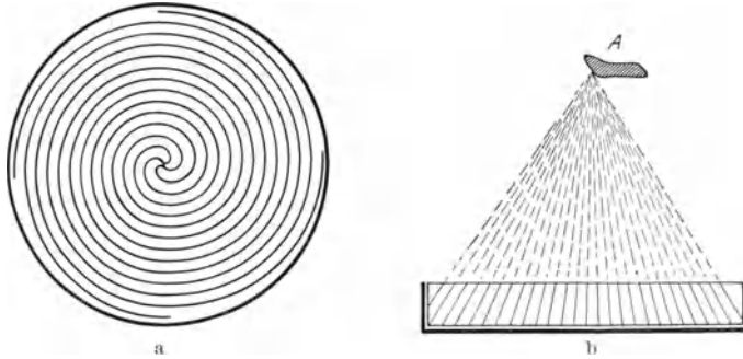
Abb. 77. Die Spiralblende. a Aufsicht; b Querschnitt.
