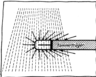
Abb. 264. Der Kammerträgerschatteneffekt. - - - = direkte Strahlung; → = gestreute Strahlung.
