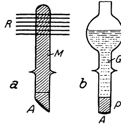
Abb. 7. Kühlung der Antikathode. a Metallkühlung. b Wasserkühlung.
