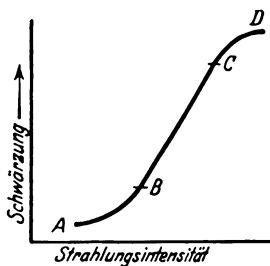
Abb. 64. Schwärzung einer photographischen Platte in Abhängigkeit von der Strahlungsintensität. Der Verlauf der Kurve gibt die Gradation der Emulsion an.
