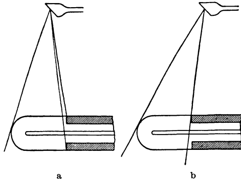
Abb. 265. a Falsche, b richtige Stellung der Kammer zur Ausschaltung des Bleieffektes.
