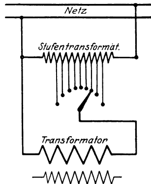
Abb. 20. Regulierung der Transformatorspannung mittels des Stufentransformators (Grobregulierung).
