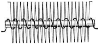
Abb. 14. Übereinandergestülpte Spulen eines Transformators.
