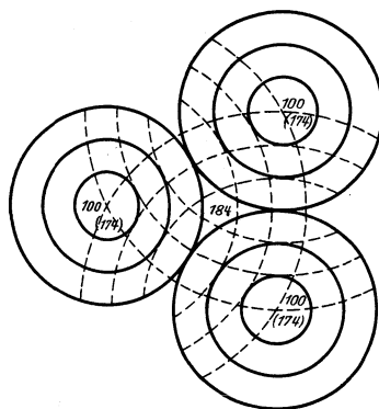
Abb. 283. Intensitätsverteilung bei der Totalbestrahlung. Die Totalbestrahlung führt bei Hinter- und Nebeneinanderreihung mehrerer Felder zu recht beträchtlichen Dosensumationen. Bei einer Intensität von 100 pro Feldmittelpunkt herrscht am Berührungspunkt der drei Felder die Intensität 184, in den Feldmittelpunkten selbst steigt die Intensität infolge Einwirkung der Randzonen der Nachbarfelder auf 174. Dieser Umstand ist bei Bestrahlung mit Dosen, die 30% der HED überschreiten, zu berücksichtigen. (Nach SCHREUS und BERGERHOFF.)
