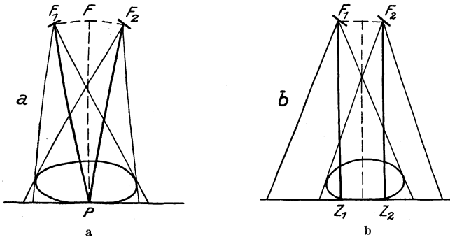
Abb. 258a und b. Die Methode der stereoskopischen Reproduktion.
