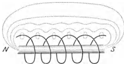
Abb. 13. Kraftlinien eines Solenoids.
