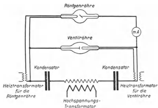
Abb. 40. Schaltungsschema nach VILLARD zum Halbwellen-Kondensatorapparat.
