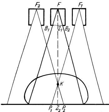
Abb. 255. Die Blendenrandmethode. In der Stellung F wird bei enger Blende der dem Fremdkörper K entsprechende Projektionspunkt Z_2 (orthodiographischer Fußpunkt) bestimmt. Sodann wird bei schlitzförmig geöffneter Blende die Röhre nach F_1 , so weit verschoben, bis der Randstrahl durch den Körper K hindurchgeht; es resultiert auf dem Schirm der Projektionspunkt P_1 . Indem man das gleiche bei Verschiebung nach der anderen Seite vornimmt, erhält man den Punkt P_2 . Aus der Distanz der Punkte P_1 und P_2 läßt sich, wenn Blendenweite ( B_1, B_2 ) und Fokus-Blendenabstand ( FZ_1 ) bekannt sind, die Entfernung des Körpers K vom Punkte Z_2 berechnen.
