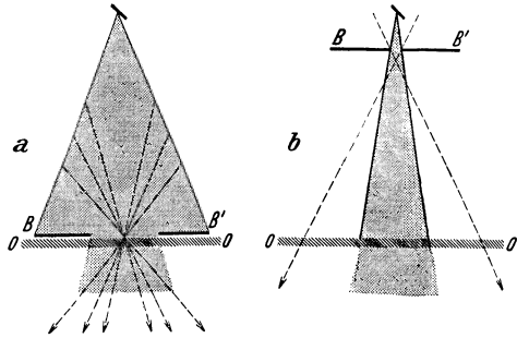
Abb. 296. Wirkung der Abblendung auf die Nebenstrahlung (gestrichelt), a bei körperaufliegender Blende, b bei röhrennaher Blende. BB' = Blende, OO = Körperoberfläche.
