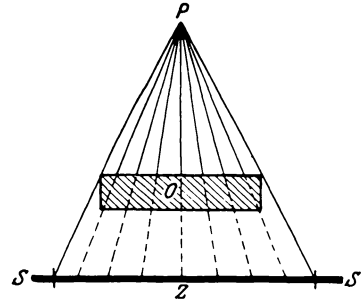
Abb. 60. Die Bildgröße in Abhängigkeit von der Objekt-Platten- und Fokus-Plattenentfernung.
