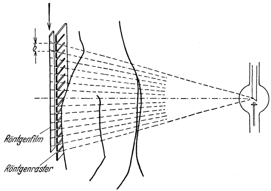
Abb. 260. Anordnung zur kymographischen Aufnahme. b = Weglänge des Rasters entsprechend einem Schlitzabstand.
