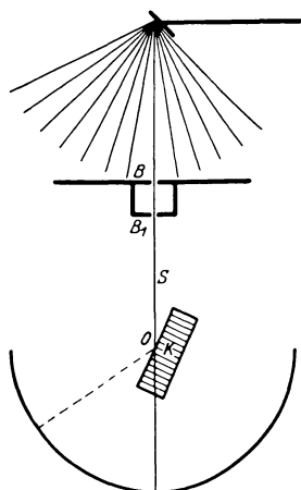
Abb. 50. Der Spektrograph.
