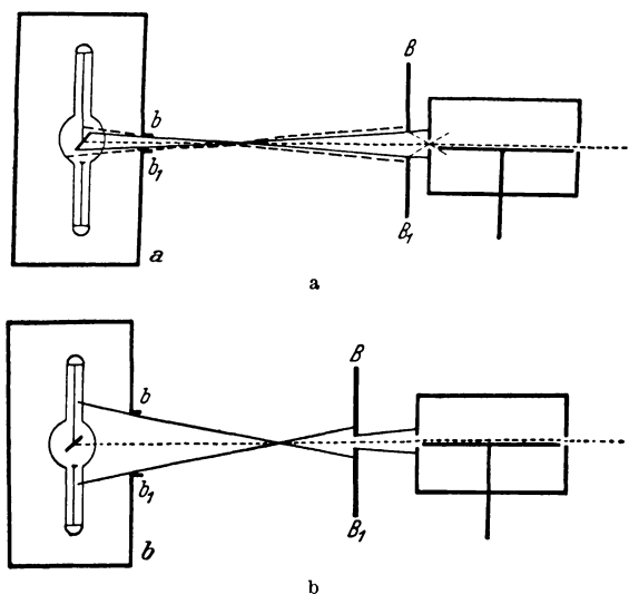
Abb. 262. Anordnung zur Messung der Einfallsstrahlung. a Unrichtige Anordnung: die röhrennahe Blende bb_1 ist zu eng geschlossen; die Zwischenblende BB_1 steht zu nahe an der Kammer; die Sekundärstrahlung, die von der Blende ausgeht, kann in die Kammer gelangen. b Richtige Anordnung.
