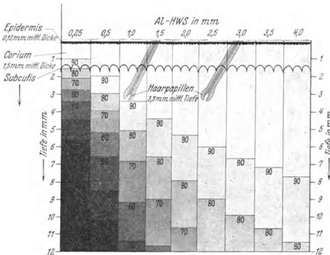
Abb. 277. Intensitätsverteilung der Röntgenstrahlen in der Haut in Abhängigkeit von der Al-HWS (nach WUCHERPENNIG).
