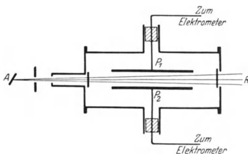
Abb. 55. Die große Ionisationskammer.
