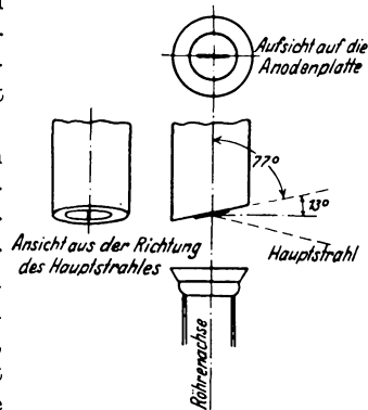
Abb. 68. Gestaltung und Wirkungsweise des bandförmigen Brennflecks nach GOETZ.
