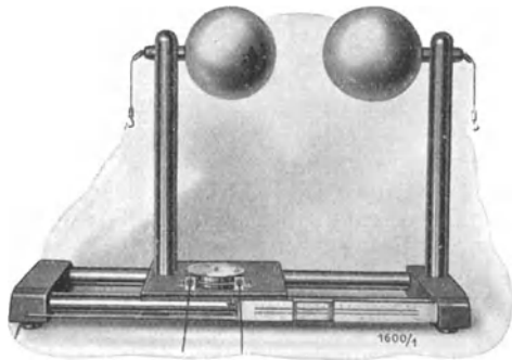
Abb. 41. Die Kugelfunkenstrecke.
