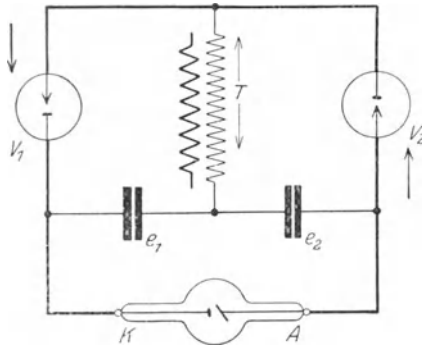
Abb. 37. Schaltungsschema z. Kondensatorapparat. Während der einen Phase ist der Stromkreis für den Transformator T über V_1 und C_1 geschlossen, während der anderen Phase bleibt nur der Weg über C_2 und V_2 .
