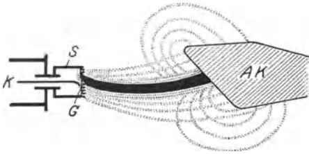
Abb. 9. Die Innenteile einer Elektronenröhre. K = Kathode, AK = Antikathode, G = Glühdraht, S = Sammelkelch.
