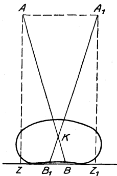
Abb. 257. Die Verschiebungsaufnahme. Es wird das gleiche Objekt zweimal exponiert, und zwar das eine Mal von A , das andere Mal von A_1 aus; dabei wird der Körper K nach B , bzw. nach B_1 projiziert. Durch Rekonstruktion des Strahlenganges läßt sich der Schnittpunkt K der Strahlen AB und A_1B_1 , der der Lage des Körpers K entspricht, jeweils bestimmen.
