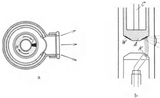
Abb. 67a und b. Die Rotalixröhre. a Querschnitt durch die Drehanode. W Wolframröhre, F die jeweils bei der Drehung als Brennfleck wirkende Fläche der Wolframröhre. b Längsschnitt durch die Rotalixröhre. A Anode, K Kathode, W Wolframröhre, C Drehachse der Anode.
