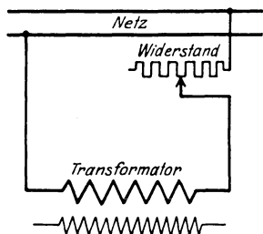
Abb. 19. Regulierung der Transformatorspannung mittels eines der Primärspule vorgeschalteten Ohmschen Widerstandes.
