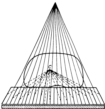
Abb. 72. Wirkungsweise der Vorderblende. Die von Punkt C ausgehende Streustrahlung fällt auf die in der Richtung der Primärstrahlung eingestellten Lamellen und wird von diesen absorbiert.
