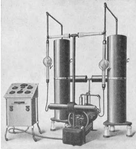
Abb. 36. Der Kondensatorapparat (Stabilivolt der Siemens-Reiniger-Verfa). CC = Kondensatoren; VV = Ventilröhren; T = Transformator.
