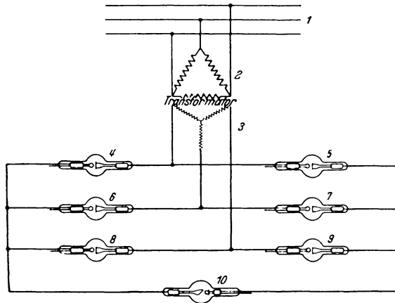
Abb. 34. Gleichrichtung des Drehstroms durch 6 Ventilröhren in GRÄTZSCHER Schaltung. Wirkungsweise wie in Abb. 29.
