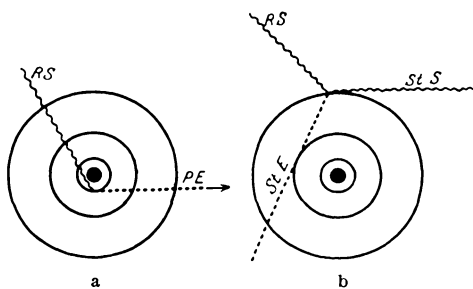
Abb. 48a und b. Links: schematische Darstellung der Emission eines Photoelektrons. Rechts: schematische Darstellung der Emission eines Streuelektrons.
