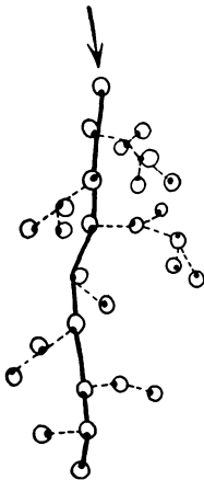
Abb. 268. Die Bahnen eines Photoelektrons (ausgezogene Linie) und seiner Sekundärelektronen (gestrichelte Linien).
