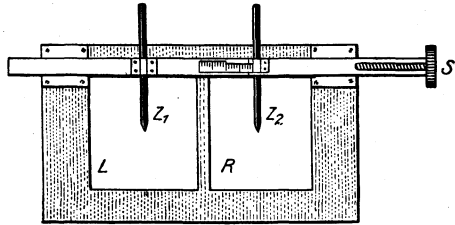
Abb. 259. Vorrichtung zur Messung im stereoskopischen Bilde mit Hilfe der „wandernden Marke“.
