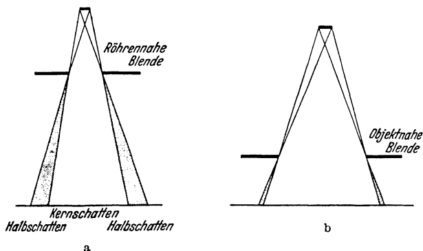
Abb. 71. Wirkungsweise a der röhrennahen, b der objektnahen Blende.
