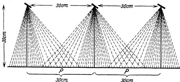
Abb. 282. Die Methode der Totalbestrahlung nach HOLZKNECHT.
