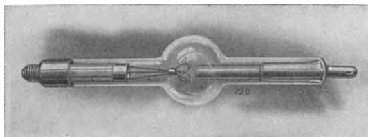
Abb. 22. Glühkathodenventilröhre (C. H. F. Müller). Links die aus drei Wolfram-Drahtschlingen bestehende Glühkathode, rechts die Anode.
