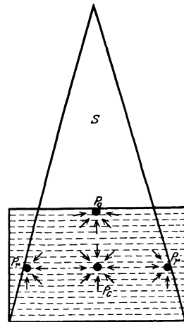
Abb. 289. Schematische Darstellung des Streuzusatzes in Abhängigkeit von der Lage des Raumpunktes im durchstrahlten Medium.
