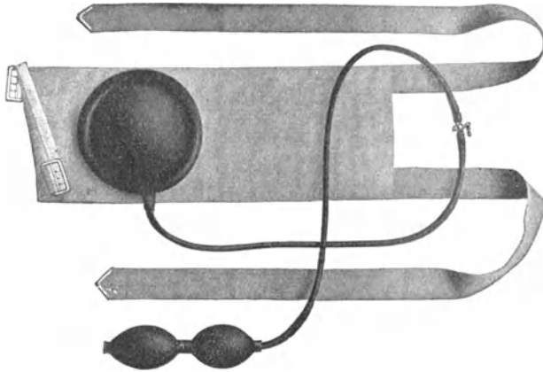
Abb. 169. Der CHAOUlsche Kompressionsgurt.
