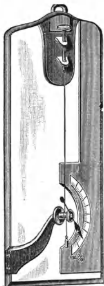
Abbildung 14. Hygrometer.
