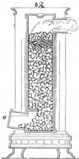
Abbildung 36. Füllöfen.
