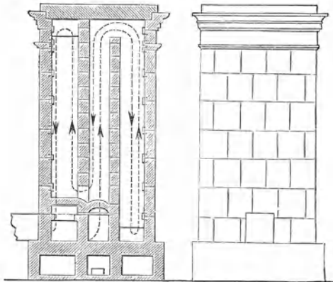
Abbildung 38. Kachelofen im Durchschnitt von vorn.
