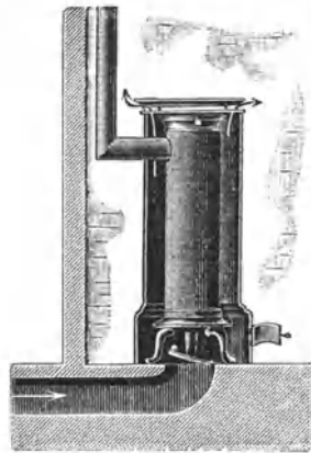
Abbildung 37. Mantelöfen.
