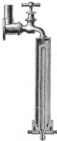
Abbildung 21. Rieselgurfilter nach Berkefeld.
