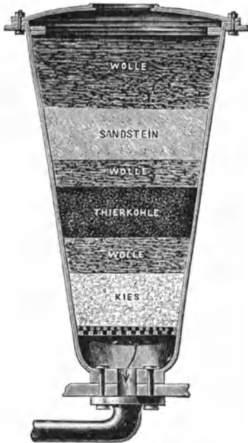
Abbildung 20. Zusammengefügtes Hausfilter.
