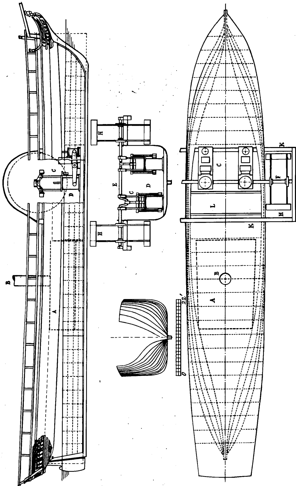
Проект парохода для линии Одесса — Редут-Кале завода Берда.
