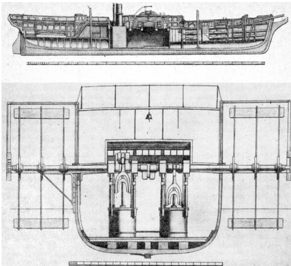
Чертеж парохода «Дарго» Продольный разрез и миделевое сечение.
