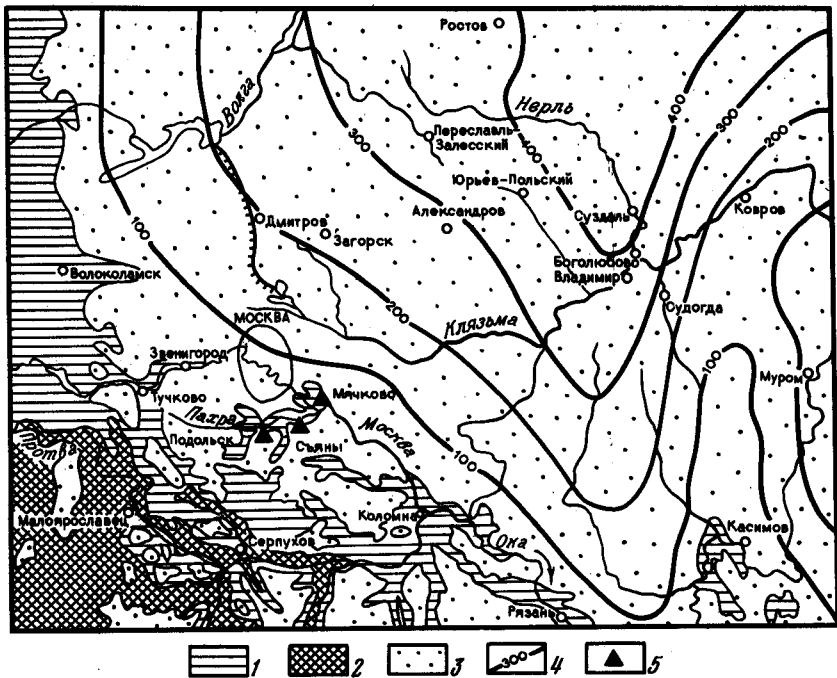
Рис. 1. Схема распространения среднекаменноугольных отложений в Подмосковье и прилегающих областях (составлена с использованием материалов П. В. Флоренского и М. Н. Соловьевой):
