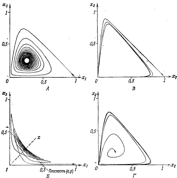
Рис. 34. Траектории динамических систем 4, 5 и 12 для элементарно. (1) n = 4 : начальные условия — x_1(0) = 0,97 , x_2(0) = 0 ; дна траектории на плоскость (x_1, x_2) . Траектория ведет по но затухают. Б. Проекция траектории на плоскость (x_1, x_3) . рис. 31] пересекает плоскость (x_1, x_3) по прямой x_1 + x_3 = 1/2 . рия пересекает плоскость (x, y) только в отдельных точках (табл. 11). (2) n = 5 : проекции на плоскость (x_1, x_2) . В. На- = x_5(0) = 0,0001 . Г. Начальные условия: x_1(0) = 0,2004 , ческая система приближается к одному и тому же предель- (3) n = 12 : проекции на плоскость (x_1, x_2) . Д. Начальные чальные условия: x_1(0) = 0,0848 , x_2(0) = \dots = x_{12}(0) = очень близко к контуру 1—2, 2—3, ..., 11—12, 12—1.
