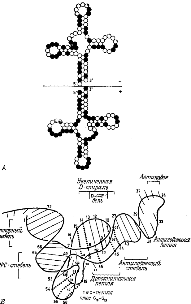
Рис. 14. Симметрия функциональных молекул РНК (рассмотрена на тРНК Phe ) способствует репликации одиночных цепей специфически адаптированными ферментами. Плюс- и минус-цепи симметричной структуры имеют одинаковые фенотипические особенности. Хотя в современных организмах транспортные РНК кодируются генотипически, их симметрия, возможно, еще отражает первичный механизм репродукции одноцепочечных РНК, при котором плюс- и минус-цепи одинаково важны. Эта симметрия наиболее очевидна на уровне вторичной структуры (А), хотя она проявляется также на уровне третичной структуры (Б) (из [46]).
