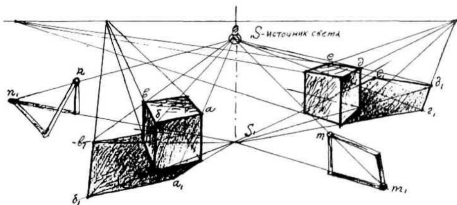
7.1. Схема, поясняющая процесс получения перспективного изображения тени
