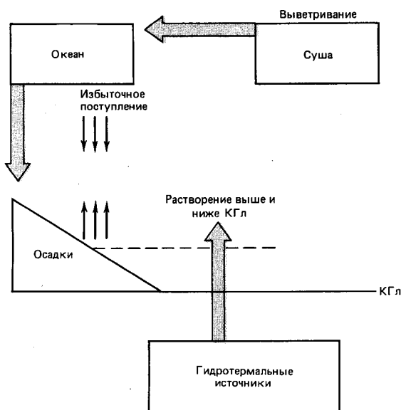
Рис. 14-3. Главные компоненты карбонатной системы океана [862].
