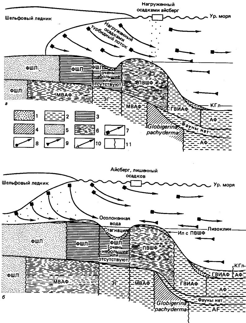
Рис. 13-23. Схематические разрезы через континентальную окраину Антарктиды, демонстрирующие распространение фаций и комплексов бентоносных фораминифер. a – при отступании шельфового ледника с водным основанием (ранняя стадия межледниковья?); б – при отступившем шельфовом леднике с водным основанием (межледниковье?) [9]. Условные обозначения и буквенные индексы те же, что на рис. 13-22.
