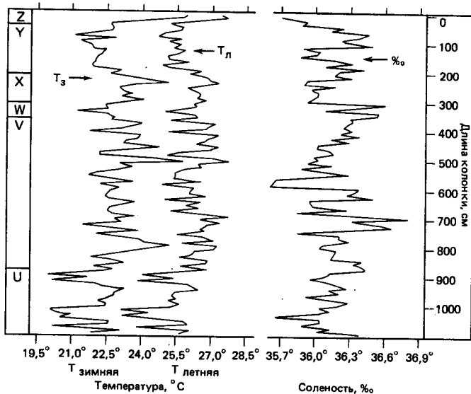
Рис. 17-20. Рассчитанные по приведенным в тексте уравнениям значения палеотемператур (зимней и летней) и палеосолености поверхностных вод в районе колонки из Карибского моря. Индексы слева—фораминиферовые зоны ([506], с. 118; публикуется с разрешения издательства Йельского университета).
