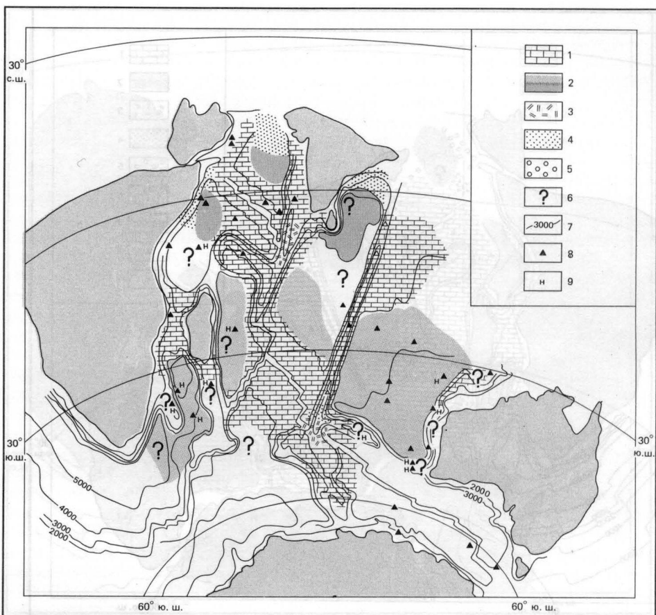
Рис. 18-14. Распространение осадков в Индийском океане в раннем олигоцене [237, с. 41] на палеобатиметрической основе для 36 млн. лет назад [Sclater et al., 1976]. Условные обозначения см. на рис. 18-12.
