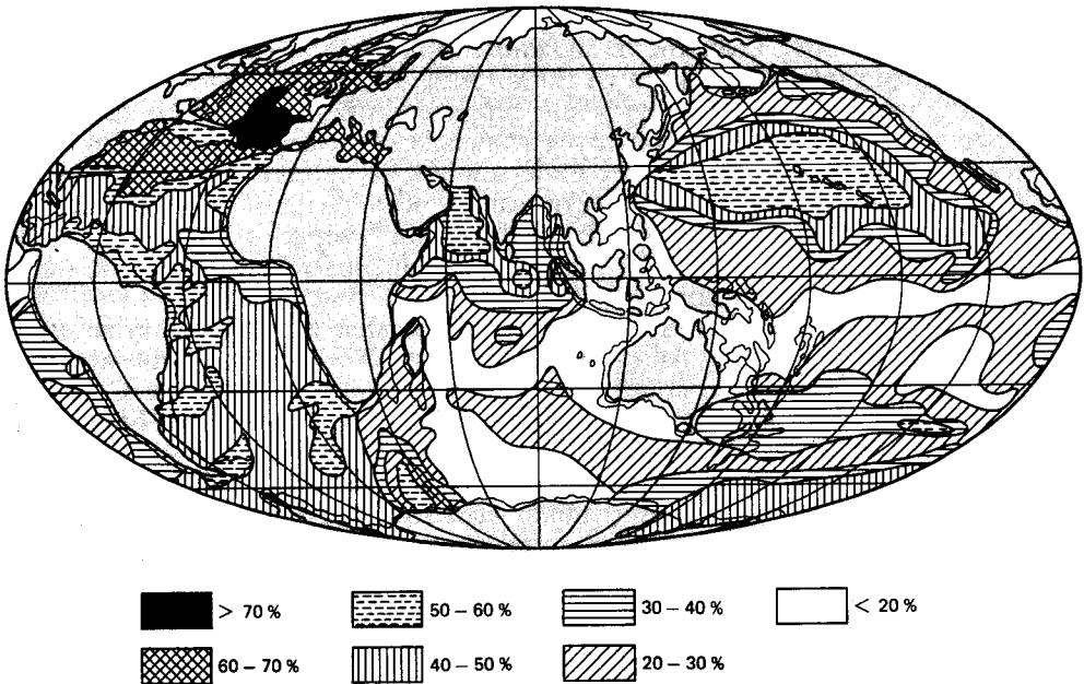
Рис. 13-14. Конкретия иллита во фракции мельче 2 мкм поверхностного слоя осадков Мирового океана. Обращают на себя внимание максимальные концентрации в некоторых районах средних широт [1141].
