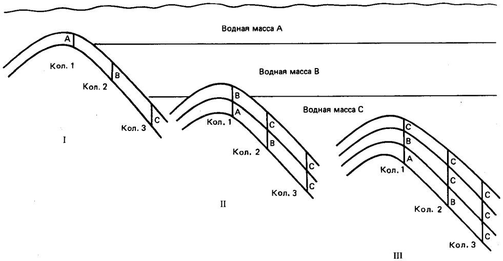
Рис. 17-2. Схема погружающегося океанского хребта для трех временных интервалов, показывающая влияние трех вертикально стратифицированных водных масс на осадконакопление на хребте: А, В, С—водные массы; 1, 2, 3—колонок; I, II, III—временные интервалы.
