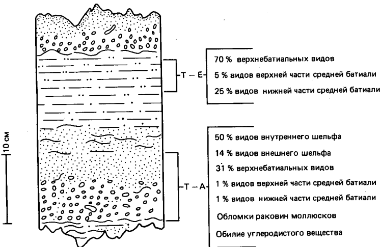
Рис. 13-9. Источники поступления бентосных фораминифер в пласте турбидита из плиоценового разреза формации Пикю в южной Калифорнии (каньон Балком). Предполагается, что баттиальные виды живут на месте осаждения, а остальные принесены турбидными потоками [511].
