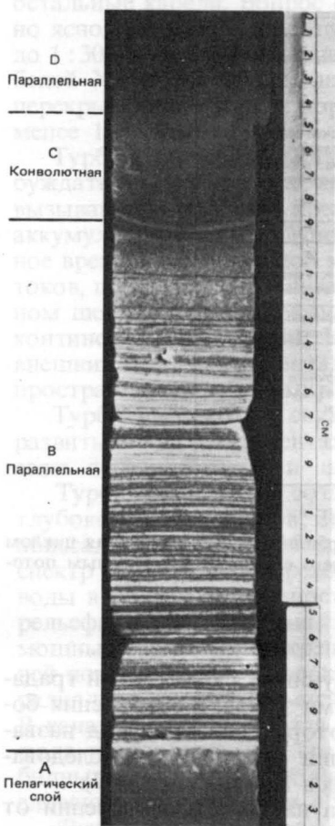
Рис. 13-8. Фотография керна бурения с турбидитами из юго-восточной части Тихого океана. Выделены интервалы полного цикла Боума [1048].
