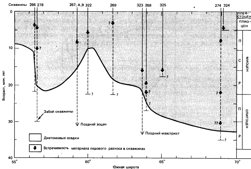
Рис. 19-18. Временное и пространственное распространение диатомовых осадков и материала ледового разнуса в скважинах глубоководного бурения в Южном океане, пробуренных в рейсах 28, 29, 35 «Гломара Челленджера». Прослеживается диахронное меридиональное распространение.
