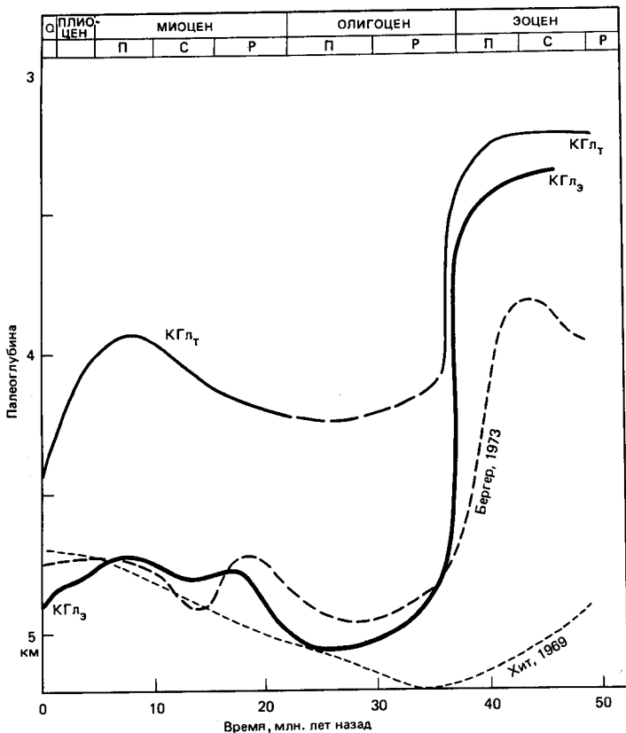
Рис. 19-14. Изменения компенсационной глубины карбоната (КГл) в кайнозое в экваториальной зоне, между 3° с.ш. и 3° ю.ш. (КГл₃), и в Тихом океане, севернее 4° с.ш. и южнее 4° ю.ш. (КГлₜ) [1075]. Для сравнения приведены кривые колебания КГл, полученные Хитом [441] и Бергером [68]. На всех кривых видно резкое опускание КГл у границы эоцено-олигоцен [1075].
