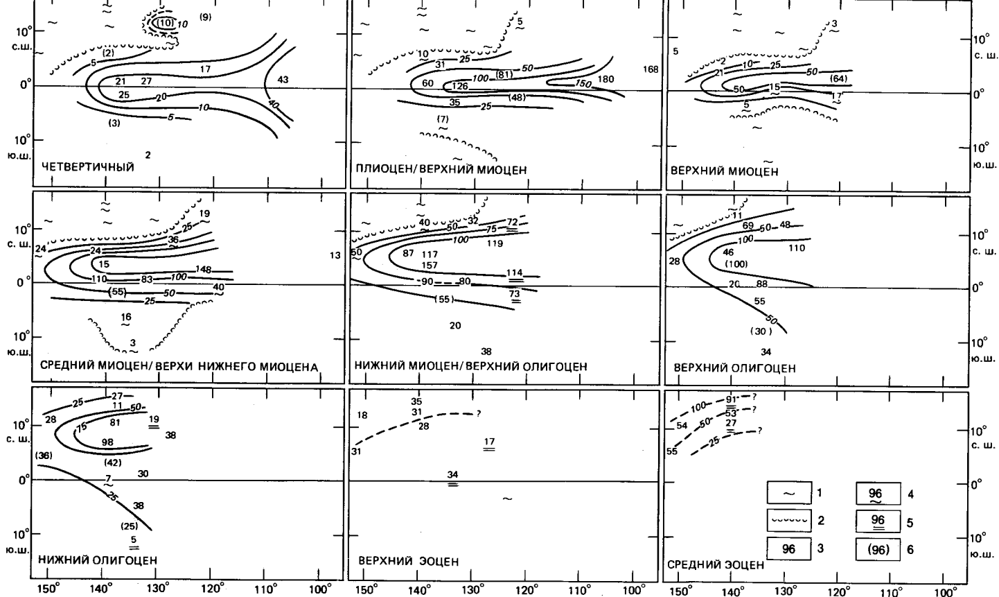
Рис. 17-12. Карты изопахит осадков экваториальной части Тихого океана для девяти кайнозойских временных срезов. Жирным пунктиром на карте эоцена показаны очень неопределенные изопахиты ([1075], публикуется с разрешения Геологического общества США). 1 – интервал отсутствует; 2 – граница полного размыва; 3 – общая мощность интервала в метрах; 4 – то же с учетом эрозии; 5 – то же до фундамента; 6 – то же на основании интерполяции границ.
