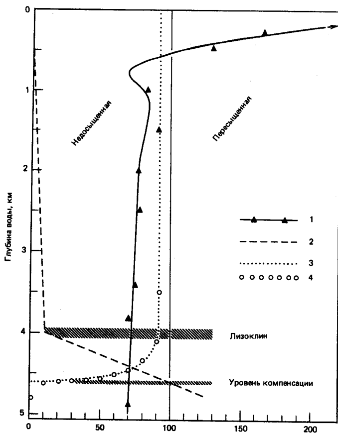
Рис. 14-6. Параметры, влияющие на распространение карбоната кальция в осадках экваториальной области Тихого океана с увеличением глубины [1075]. 1—насыщение кальцитом (%); 2— \frac{\text{скорость растворения}}{\text{скорость поступления}} \times 100 ; 3—содержание CaCO 3 в осадках рассчитанное; 4—содержание CaCO 3 в осадках наблюдаемое.
