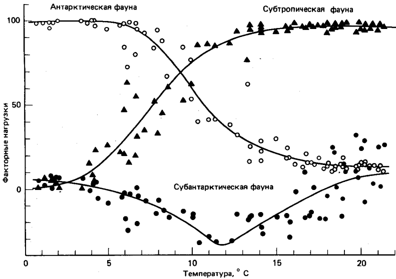
Рис. 16-19. Связь изменений факторов, или комплексов, радиоларий в поверхностных осадках с изменениями февральских температур поверхностных вод в Южном океане. Доминирование выражено в виде факторных нагрузок, \times 100 . Прослеживаются изменения соотношения между тремя доминирующими группами [674].
