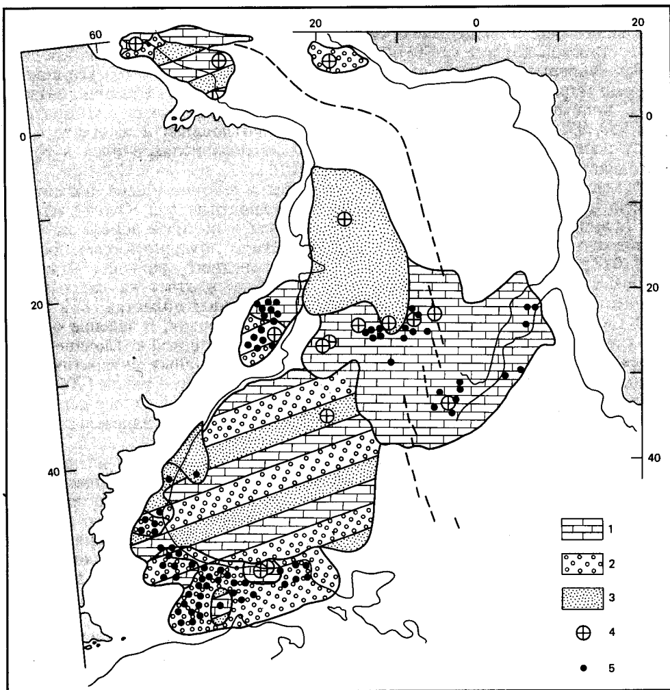
Рис. 18-10. Седиментация в Южной Атлантике в эпоху [709]. 1 – известковый ил; 2 – кремнистый ил; 3 – терригенные осадки; 4 – места проходки скважин; 5 – места взятия колонок (по-ришевыми трубками).
