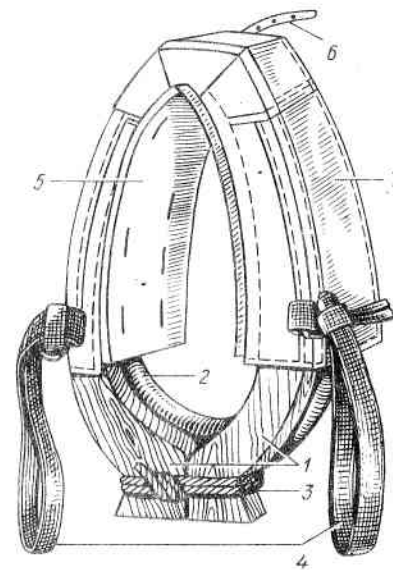
Рис. 21. Хомут неразборный стандартный сельскохозяйственный: 1 — клещи; 2 — хомутина; 3 — супонь; 4 — пара гужей; 5 — хомутная прокладка; 6 — горт; 7 — покрывка
