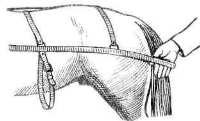
Рис. 23. Проверка степени натяжения ободового ремня шлеи
