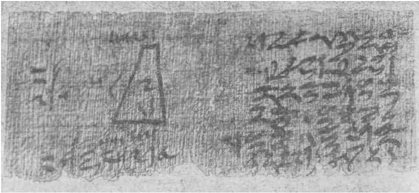
Задача на вычисление объема усеченной пирамиды из Московского математического папируса.
