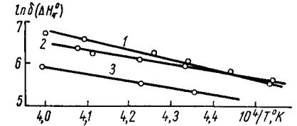
Рис. 24. Температурная зависимость прироста энтальпии, обусловленная образованием вакансий в карбидах ниобия:
