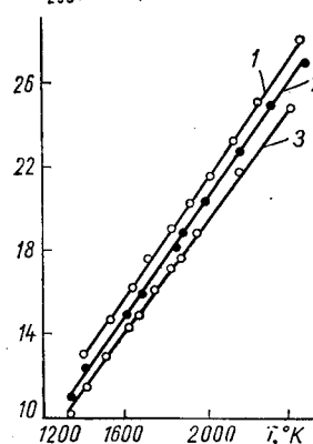
Рис. 20. Энтальпия карбидов ванадия при высоких температурах:
