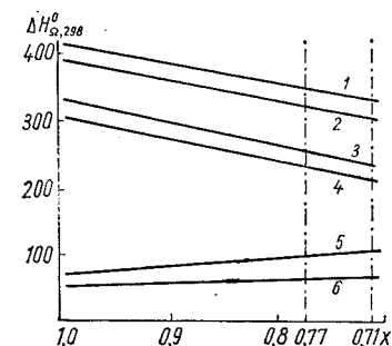
Рис. 47. Характер изменения энергий связи в карбидах ниобия и тантала в области гомогенности:
