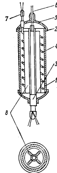
Рис. 6. Низкотемпературный калориметр.
