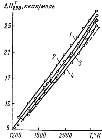
Рис. 23. Энтальпия карбидов ниобия при высоких температурах:
