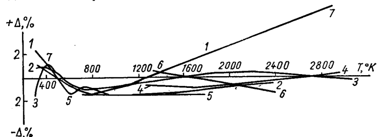
Рис. 25. Отклонение опытных значений теплоемкости карбидов ниобия, по данным различных авторов, от рассчитанных: 1 — [66]; 2 — [65]; 3 — [17]; 4 — [137]; 5 — [136]; 6 — наши данные [68]; 7 — [11].
