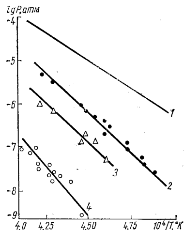
Рис. 28. Парциальные давления пара газообразных компонент над системой бор—углерод: 1 — В; 2 — ВС 2 ; 3 — В 2 С; 4 — ВС.
