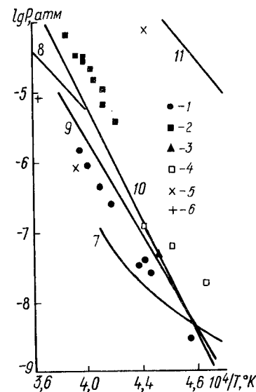
Рис. 33. Парциальные давления пара титана над системой карбид титана — углерод:
