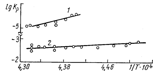
Рис. 31. Температурная зависимость констант равновесия газовых реакций в системе скандий — углерод: 1 — реакция (IV.29); 2 — реакция (IV.28).
