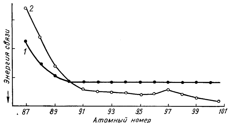
Рис. 48. Качественное сравнение энергии связи: 1 — 6 d - и 2—5 f -электроны [481].
