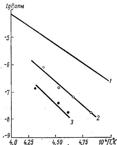
Рис. 29. Парциальные давления пара газообразных компонент над системой карбид бора — углерод: 1 — В; 2 — ВС 2 ; 3 — В 2 С.
