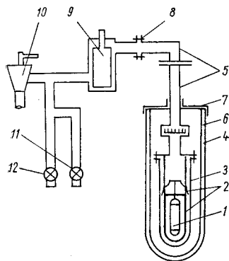
Рис. 5. Схема установки для исследования теплоемкости при низких температурах.
