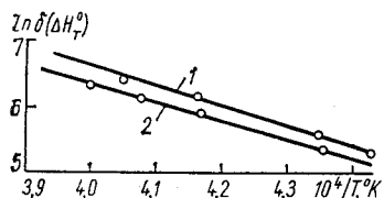
Рис. 15. Температурная зависимость прироста энтальпии, обусловленная образованием вакансий в карбидах титана:
