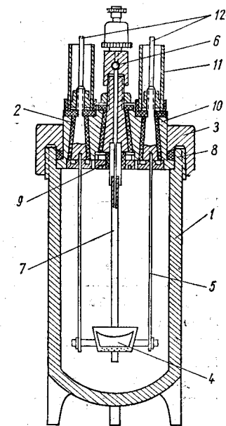
Рис. 13. Калориметрическая бомба:
