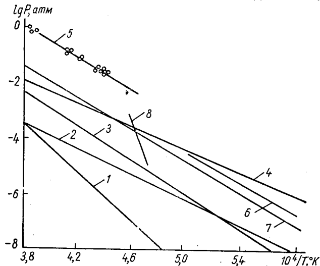
Рис. 30. Парциальное и общее давление пара над системой карбид кремния — углерод: 1 — \text{Si}_2 [184, 185]; 2 — \text{Si}_2\text{C} [184, 185]; 3 — \text{Si}_2 ; [184, 185]; 4 — \text{Si} [184, 185]; 5 — P_{\text{общ}} [180, 181]; 6 — P_{\text{общ}} [186]; 7 — P_{\text{общ}} [191]; 8 — \text{Si} [187].
