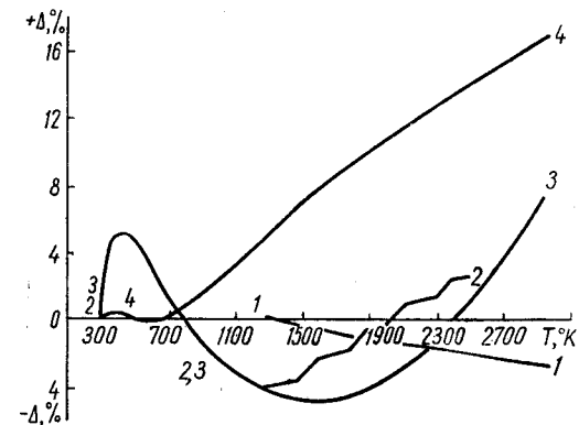
Рис. 27. Отклонение опытных значений теплоемкости карбида тантала, по данным различных авторов, от рассчитанных:
