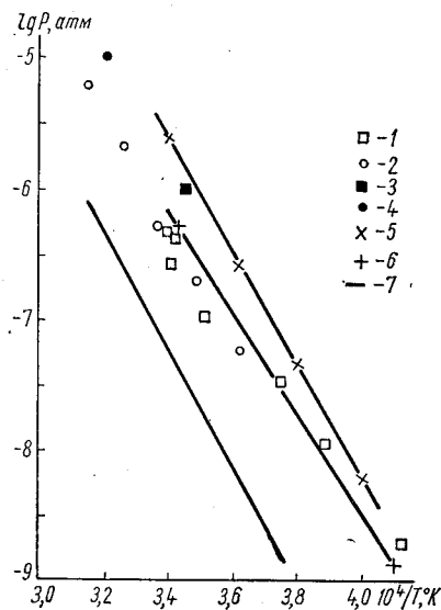
Рис. 36. Парциальные давления пара металла над карбидом ниобия по: 1 — [234]; 2 — [219, 220]; 3 — состав NbC_{0,748} [7]; 4 — состав NbC_{0,735} [7]; 5 — [214]; 6 — [239]; 7 — система NbC_{0,98} - C [7].
