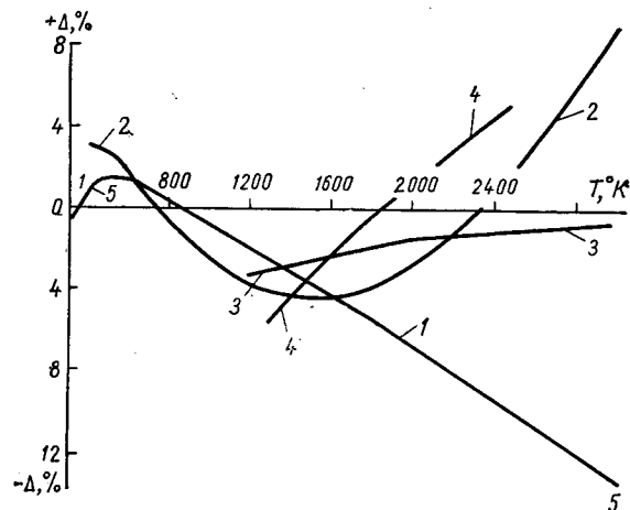
Рис. 16. Отклонение опытных значений теплоемкости карбида титана, по данным различных авторов, от рассчитанных: 1 — [114]; 2 — [7]; 3 — [70]; 4 — [69]; 5 — [11].
