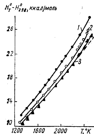
Рис. 17. Энтальпия карбидов циркония при высоких температурах: 1 — ZrC_{0,99} ; 2 — ZrC_{0,76} ; 3 — ZrC_{0,69} .
