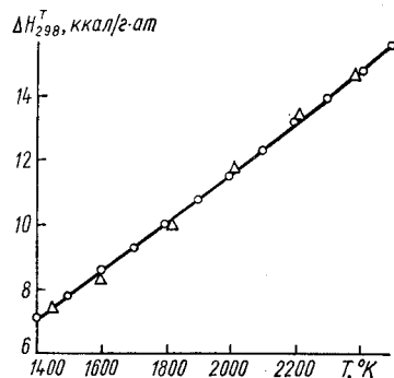
Рис. 11. Энтальпия вольфрама: \Delta — наши данные; \circ — данные работы [80].
