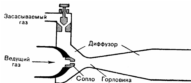
7. Устройство инжектора (схема).
