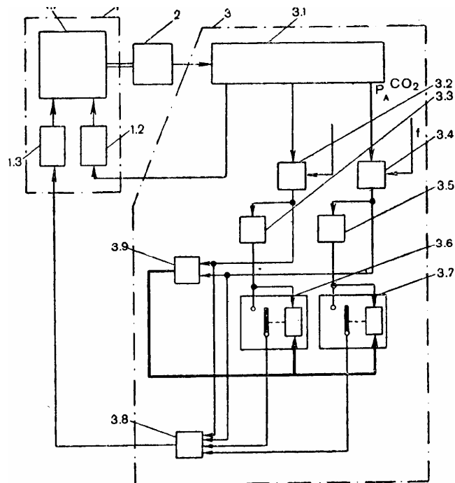
27. Блок-схема аппарата РОЛ-2. Объяснение в тексте.
