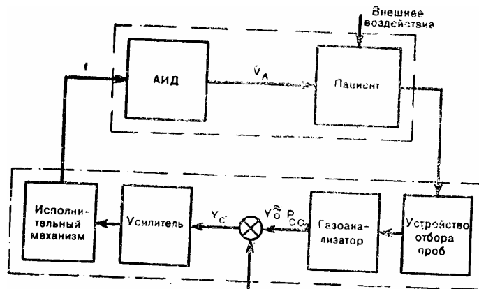
25. Блок-схема аппарата РОА-1. Объяснение в тексте.
