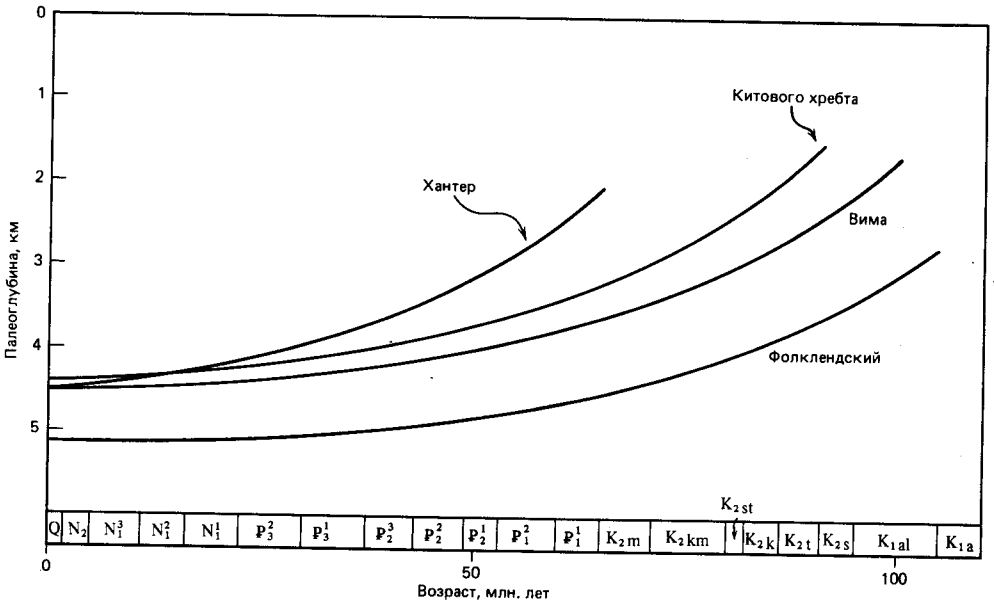
Рис. 17-5. Увеличение глубины проходов в течение мела и кайнозоя в Южной Атлантике, контролирующей циркуляцию придонных и промежуточных водных масс. Канал Фолклендской зоны разлома связывает Южный океан с Аргентинской котловиной, каналы Вима и Хантер соединяют Аргентинскую и Бразильскую котловины, канал Китового хребта располагается между Капской и Аргентинской котловинами. Погружение рассчитано по оценкам возраста в самых глубоких частях каналов и основано на предположении, что каналы сформировались на ранней стадии истории хребтов ([1077]; с разрешения издательства Чикагского университета). Q — четвертичный, N 2 — плиоцен, N 3 1 — поздний миоцен, N 2 2 — средний миоцен, N 1 1 — ранний миоцен, P 3 2 — поздний олигоцен, P 3 1 — ранний олигоцен, P 2 2 — поздний эоцен, P 2 1 — средний эоцен, P 1 2 — ранний эоцен, P 1 1 — поздний палеоцен, P 1 1 — ранний палеоцен, K 2m — маастрихт, K 2km — кампан, K 2st — сантон, K 2k — коньяк, K 2t — турон, K 2s — сеноман, K 1al — альб, K 1a — апт.
