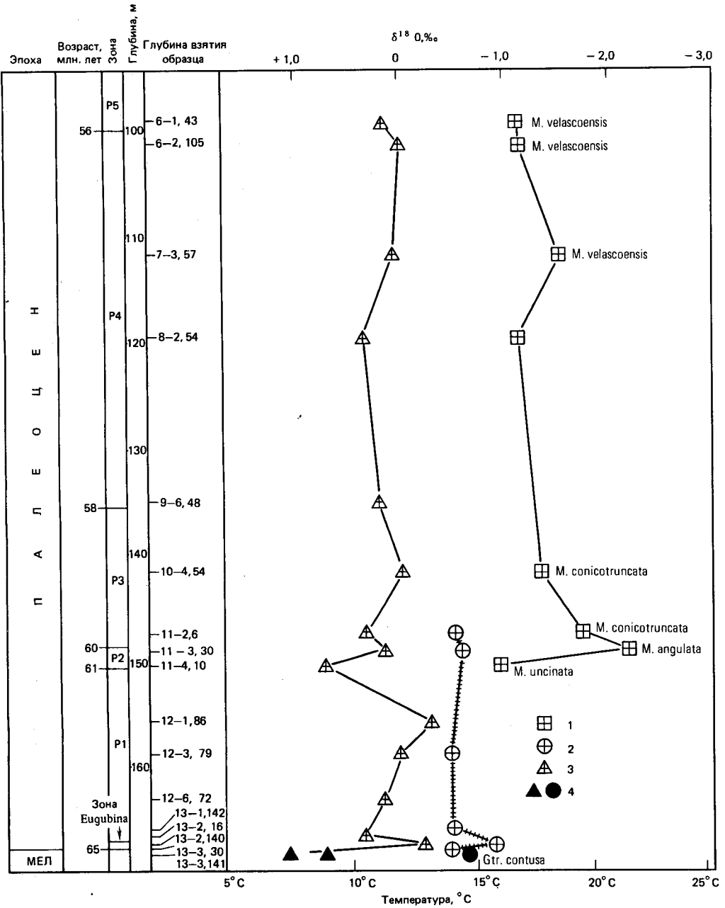
Рис. 19-7. Изотопно-кислородные кривые для границы мел-третичные отложения и палеоцена по скв. 384, Северо-Западная Атлантика. Значения \delta^{18}O бентосных фораминифер становятся легче при переходе от мела к палеоцену [112]: 1 - Morozovella ; 2 - Chilozembelina ; 3 - бентосные виды; 4 - меловые виды. \delta^{18}O дается относительно стандарта PDB.
