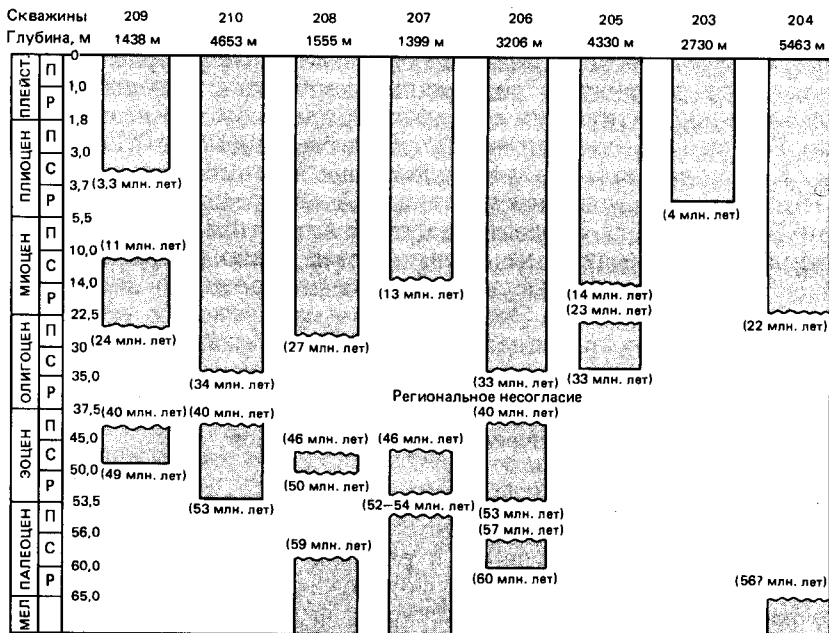
Рис. 18-18. Возраст осадков в скважинах глубоководного бурения из юго-западной части Тихого океана и положение перерывов [579]. Региональные перерывы в основном приурочены к раннему олигоцену. Р-ранний, С-средний, П-поздний.
