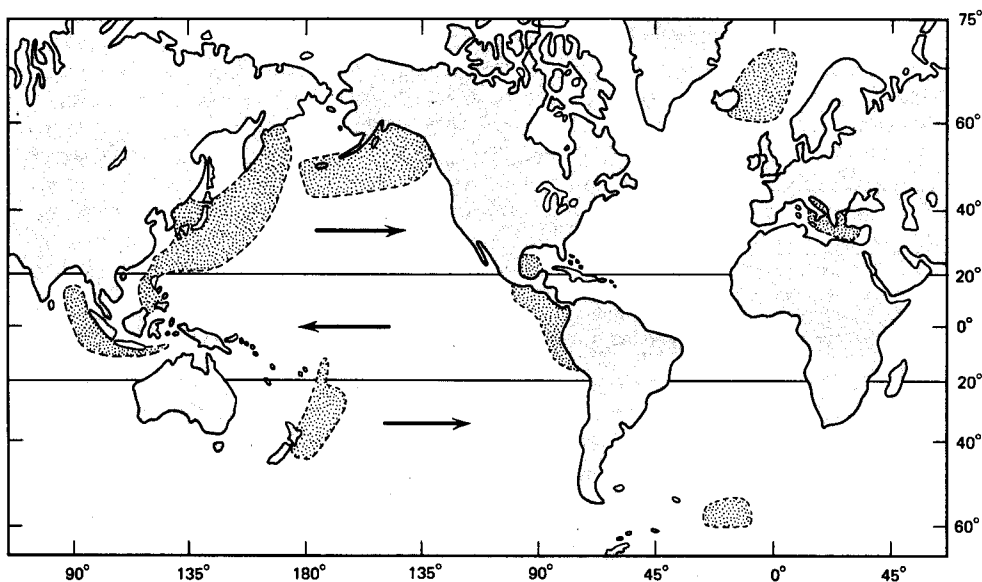
Рис. 13-19. Генерализованная схема главных ареалов современного распространения грубозернистого вулканического стекла на дне Мирового океана. Распространение стекла контролируется положением вулканических источников и направлением господствующих ветров в нижней тропосфере. Значительные различия направления ветра по вертикали в тропосфере, а также между тропосферой и стратосферой привели к более сложным контурам некоторых ареалов, не показанных на данной схеме. (Рисунок любезно предоставлен Д. Нинковичем.)
