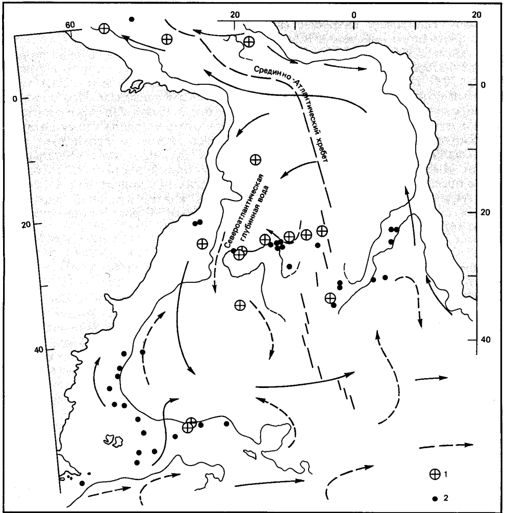
Рис. 18-11. Предполагаемая циркуляция в Южной Атлантике в эоцене [709]. Поверхностная циркуляция показана сплошными стрелками, придонная циркуляция – прерывистыми стрелками. 1 – места проходки скважин; 2 – места взятия колонок (поршневыми трубками).
