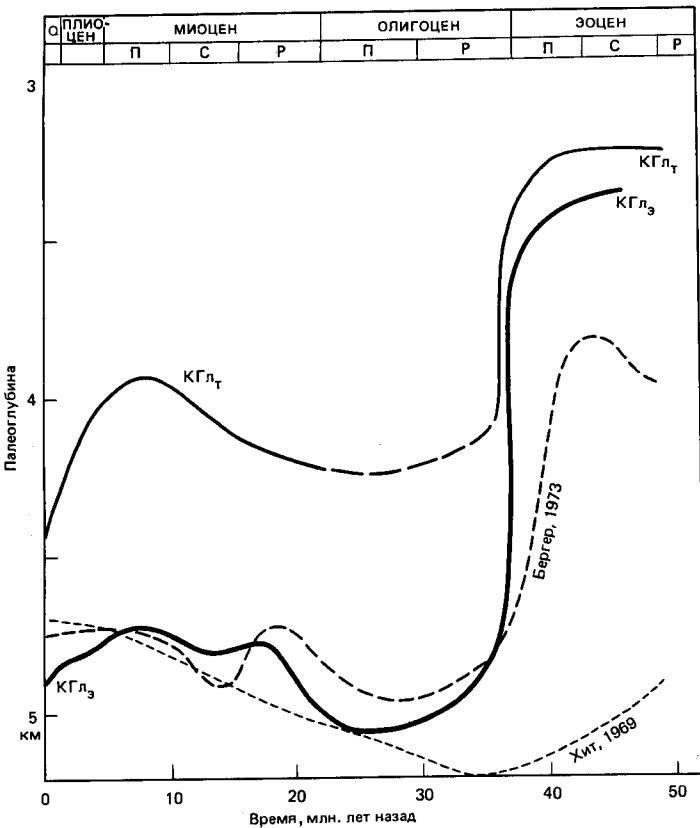
Рис. 19-14. Изменения компенсационной глубины карбоната (КГл) в кайнозое в экваториальной зоне, между 3° с. ш. и 3° ю. ш. (КГл 3 ), и в Тихом океане, севернее 4° с. ш. и южнее 4° ю. ш. (КГл 4 ) [1075]. Для сравнения приведены кривые колебания КГл, полученные Хитом [441] и Бергером [68]. На всех кривых видно резкое опускание КГл у границы эоцено-олигоцен [1075].
