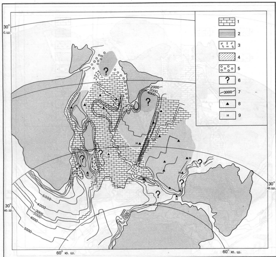
Рис. 18-13. Распространение осадков в Индийском океане в конце раннего эоцена [237, с. 43] на палеобатиметрической основе для 53 млн. лет назад [Sclater et al., 1976]. Условные обозначения см. на рис. 18-12.
