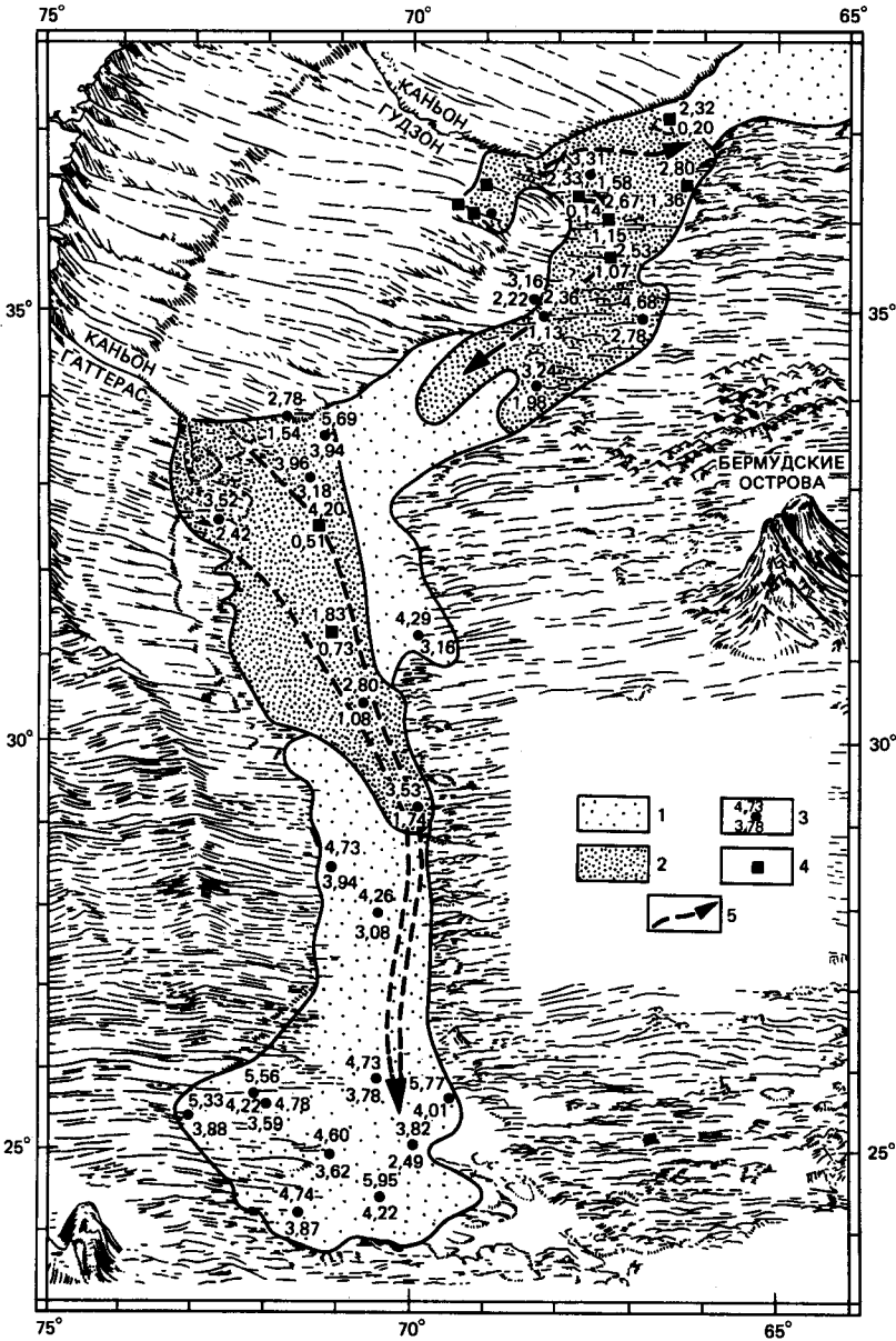
Рис. 13-12. Распространение песка и силта на абиссальной равнине Гаттерас у восточного побережья США, отложенных турбидными потоками, вытекающими из подводных каньонов. 1 - силт; 2 - песок; 3 - расположение колонок; цифрами обозначены медианный (верхняя) и максимальный (нижняя) диаметры зерен (в единицах фи) в наиболее грубозернистом базальном слое турбидита в каждой колонке; 4 - колонки с неградационными слоями; 5 - предполагаемые главные трассы турбидных потоков [488].
