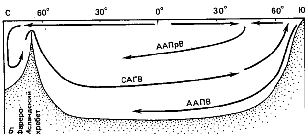
Рис. 19-21. Поперечное сечение водной толщи Атлантического океана, показывающее предполагаемую общую циркуляцию. А – домиоценовое время с поднятым Фареро-Исландским хребтом; Б – послемииоценовое время с погружившимся Фареро-Исландским хребтом, через который перетекают воды Норвежского моря [919]. ААПВ – антарктические придонные воды, ААПрВ – антарктические промежуточные воды, САПВ – североатлантические промежуточные воды, САГВ – североатлантические глубинные воды.
