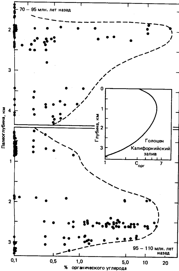
Рис. 14-20. Вариации содержания C_{\text{орг}} в осадках Южной Атлантики с глубиной (в км) для двух интервалов мелового периода (70–95 млн. лет назад и 95–110 млн. лет назад). На врезке показано изменение содержания C_{\text{орг}} с глубиной в современных осадках Калифорнийского залива. Обращает на себя внимание максимальное содержание C_{\text{орг}} на глубинах распространения промежуточных вод, связанных со слоем кислородного минимума в этом районе [1039].
