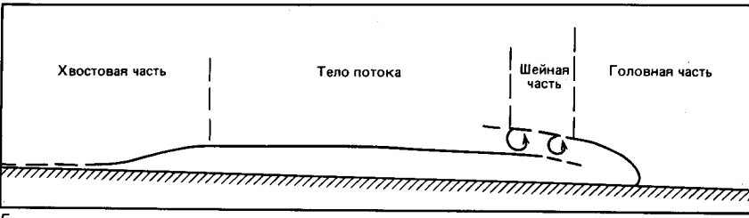
Рис. 13-6. Гидравлика турбидных потоков по лабораторным экспериментам в лотках. А. Волна турбидного потока, наблюдавшаяся в горизонтальном канале после спуска суспензии из шлюзовой камеры в одном его конце. Скорость головной части потока V зависит от толщины головной части ( d_2 ), разности плотностей суспензии в турбидном потоке и воды над ним ( \Delta\rho ), плотности воды \rho и ускорения силы тяжести g . Б. Стационарный однородный турбидный поток вниз по склону g . Средняя скорость потока u зависит от толщины потока d , разности плотностей, сил трения на границе с дном ( f_0 ) и с вышележащей водой ( f_i ). В. Характер движений внутри и вокруг головной части турбидного потока. Г. Схема расчленения турбидного потока на головную часть, тело и хвостовую часть [742].
