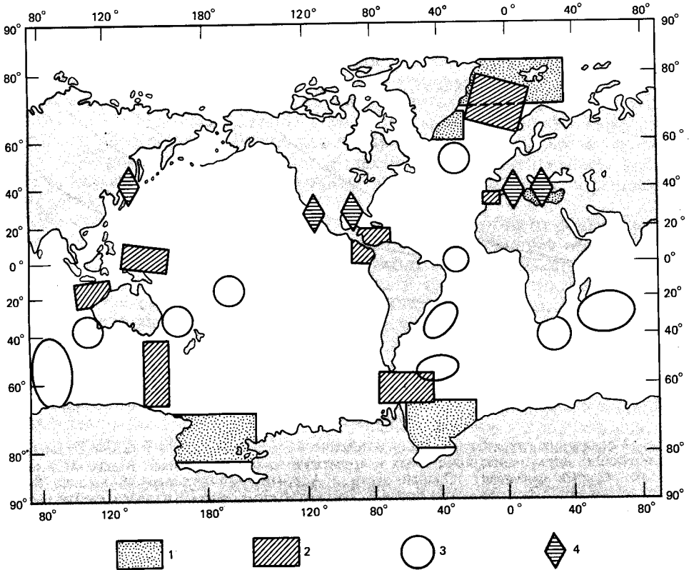
Рис. 17-4. Районы, игравшие особо важную роль в истории эволюции Мирового океана. 1—источники придонных вод; 2—важнейшие межконтинентальные проливы; 3—ключевые районы, влияющие на придонную циркуляцию; 4—окраинные моря, подверженные сильному влиянию континентов, как усилители палеоокеанологических процессов.
