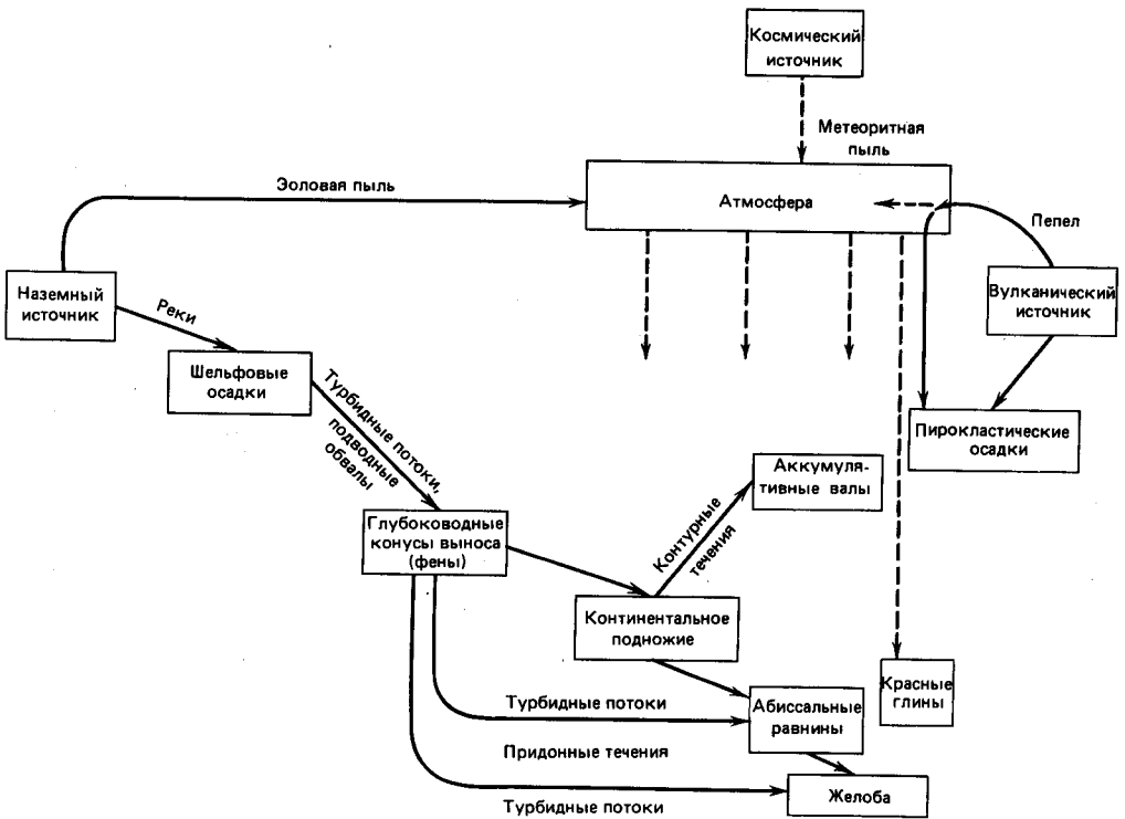
Рис. 17-7. Процессы механической седиментации ([429], публикуется с разрешения Общества разведочной палеонтологии и минералогии).
