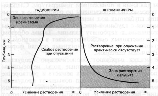
Рис. 14-1. Сравнение профилей растворения радиолярий и планктонных фораминифер, составленных по результатам натуральных экспериментов. Основная масса радиолярий (и диатомовых) растворяется в поверхностных водах. Напротив, растворение известковых микрофоссилий происходит главным образом на дне океана, на глубинах более 3,5 км [74].
