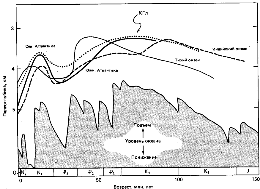
Рис. 18-16. Временные флуктуации КГл (компенсационной глубины карбоната) в Индийском, Тихом и Атлантическом океанах за последние 150 млн. лет [1072] и эвстатические колебания уровня [1068]. Q — плейстоцен, N 2 — плиоцен, N 1 — миоцен, P 3 — олигоцен, P 2 — эоцен, P 1 — палеоцен, K 2 — поздний мел, K 1 — ранний мел, J — юра.
