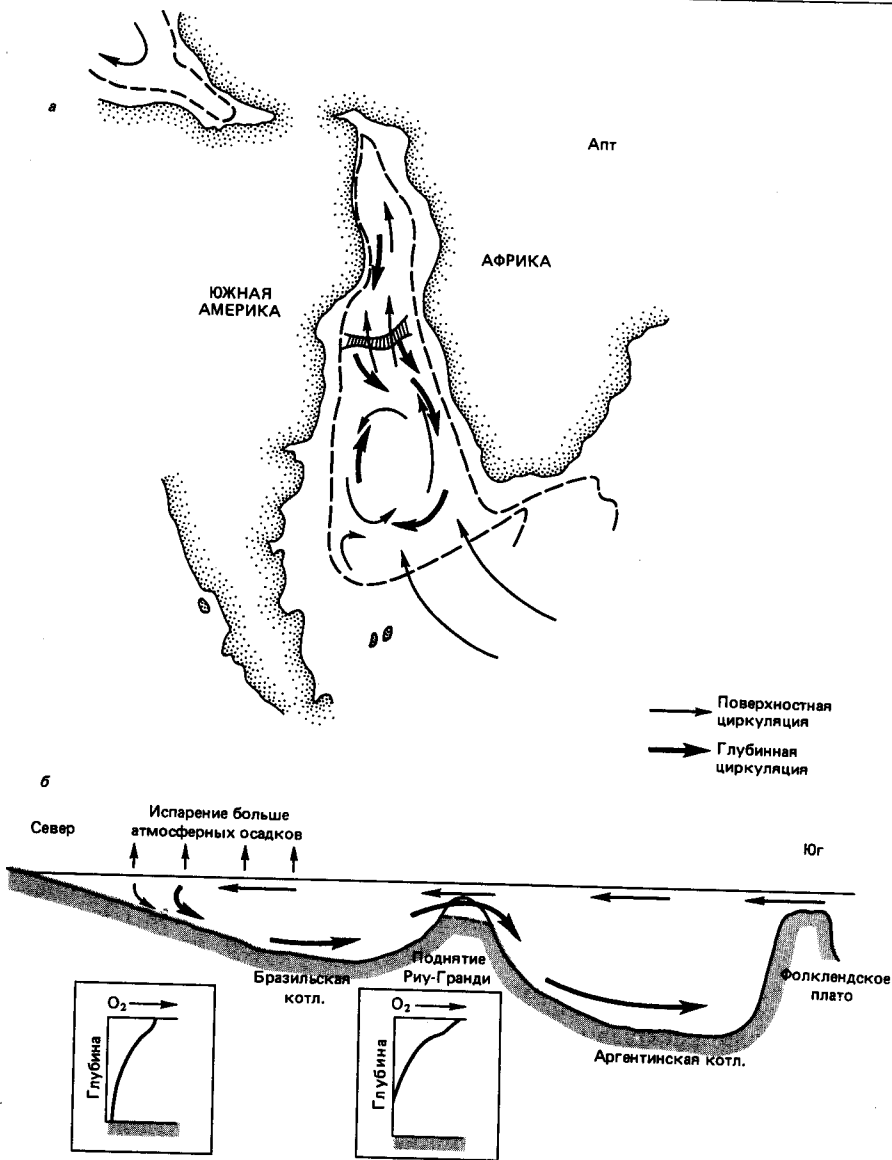
Рис. 18-6. Палеоциркуляция в Южной Атлантике в апте [709]. Полоса с поперечной штриховкой на рисунке а означает древнее поднятие Риу-Гранди. На рисунке б показаны предполагаемая меридиональная циркуляция и схематические профили вертикального распределения кислорода.
