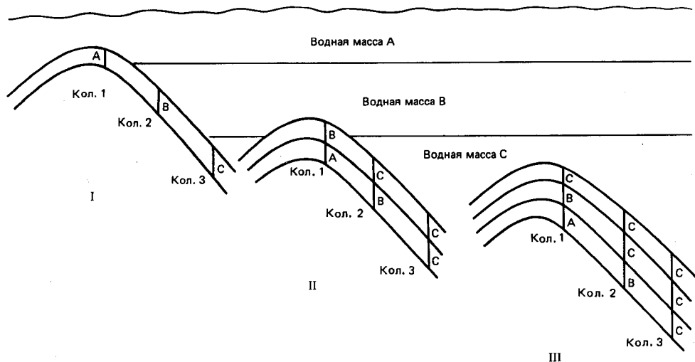
Рис. 17-2. Схема погружающегося океанского хребта для трех временных интервалов, показывающая влияние трех вертикально стратифицированных водных масс на осадконакопление на хребте: A, B, C — водные массы; 1, 2, 3 — колонки; I, II, III — временные интервалы.
