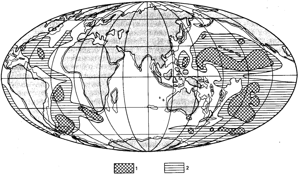
Рис. 14-25. Распространение железо-марганцевых конкреций в Тихом и Атлантическом океанах [218]. 1—плотное покрытие дна конкрециями, местами более 90%; 2—конкреции встречаются часто, хотя распределены неравномерно.
