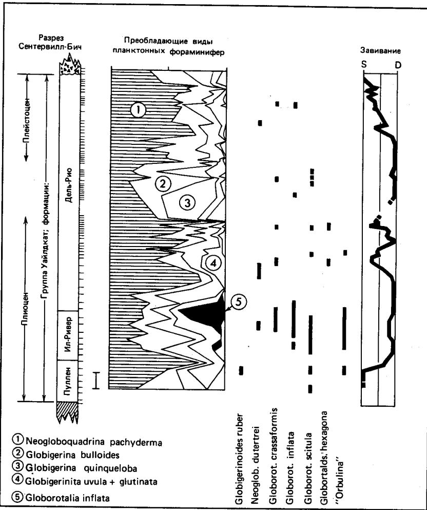
Рис. 17-15. Количественные вариации содержания планктонных фораминифер в плиоцен-плейстоценовых отложениях разреза Сентервилл-Бич в Калифорнии. Отмечено появление в среднем плиоцене комплекса переходной водной массы, для которой характерны Globorotalia inflata и S. puncticulata , указывающее на значительное повышение температур Калифорнийского течения, отразившееся в других районах северной части Тихого океана. Кроме того, показана смена направления завивания раковин Neogloboquadrina pachyderma : ось S – 100% левозавитой; ось D – 100% правозавитой. (Любезно предоставлено Дж. Инглom-старшим.)
