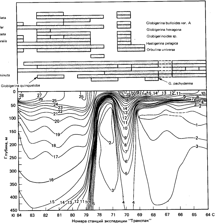
Рис. 16-3. Разрез верхней части водной толщи на границе между теплым течением Куроисио и холодным течением Ойясио, показывающий влияние этого раздела на распределение планктонных фораминифер в поверхностных водах ([125], с. 95). (Р 6503 1-3 мая 1965 г. от 2° с. ш. до 2° ю. ш. по 8° з. д.) Кружки — планктонные ловы.
