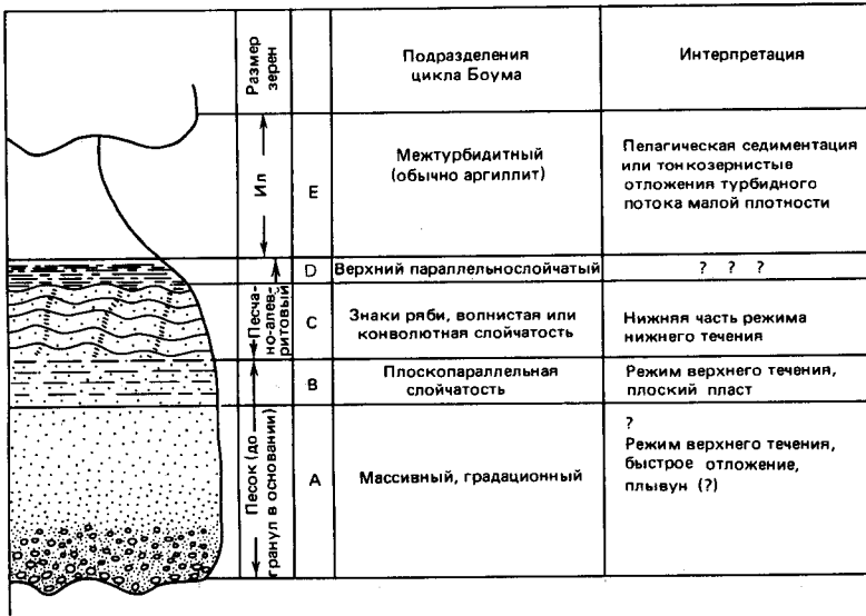
Рис. 13-7. Идеализованная последовательность слоев турбидита, часто именуемая циклом Боума (по фамилии Альфреда Боума, впервые установившего его связь с турбидным потоком). Справа дана интерпретация режима потока [742].
