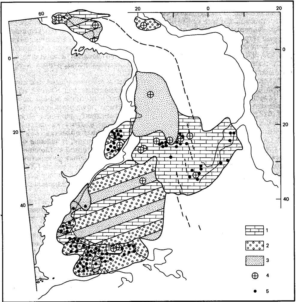
Рис. 18-10. Седиментация в Южной Атлантике в эоцене [709]. 1 — известковый ил; 2 — кремнистый ил; 3 — терригенные осадки; 4 — места проходки скважин; 5 — места взятия колонок (по-ршневыми трубками).
