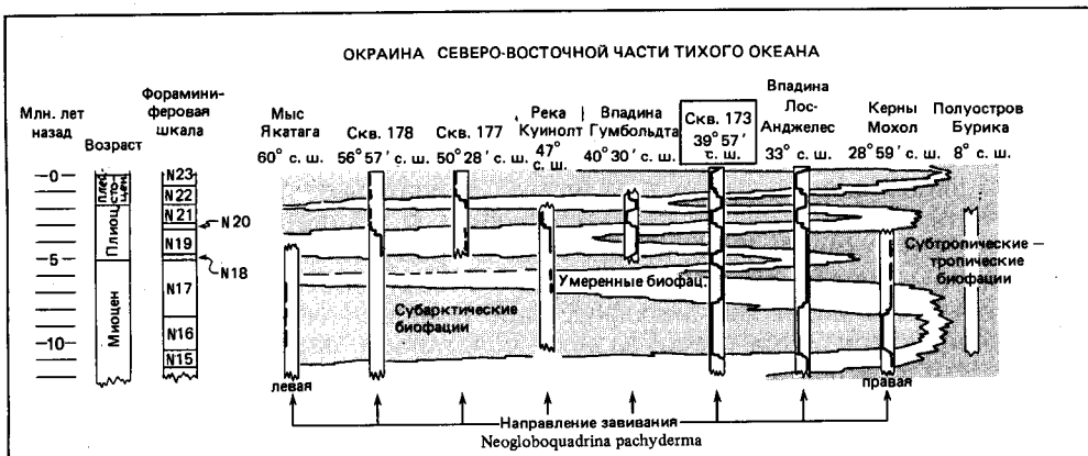
Рис. 17-18. Схема крупных неогеновых осцилляций чувствительных к температуре биофаций планктонных фораминифер в пределах Калифорнийского течения и в прилегающем к нему аляскинском круговороте по меридиональному профилю от 60 до 8° с.ш. Комплексы, содержащие только левозавитую Neogloboquadrina pachyderma , рассматриваются как индикаторы температур ниже 10°C, а комплексы, состоящие из правозавитых форм, соответствуют температурам выше 15°C. Граница между умеренной и субтропической-тропической биофациями сопоставляется с температурой 20° [511]. Скважины Проекта глубоководного бурения.
