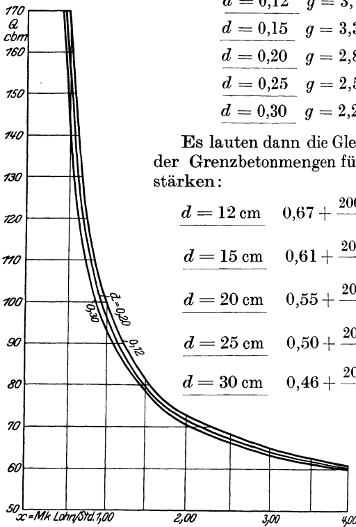
Abb. 29. Grenzbetonmengenkurven für Gußbetonhochbauten bei Verwendung einer 350-l-Gießmasthanlage.
