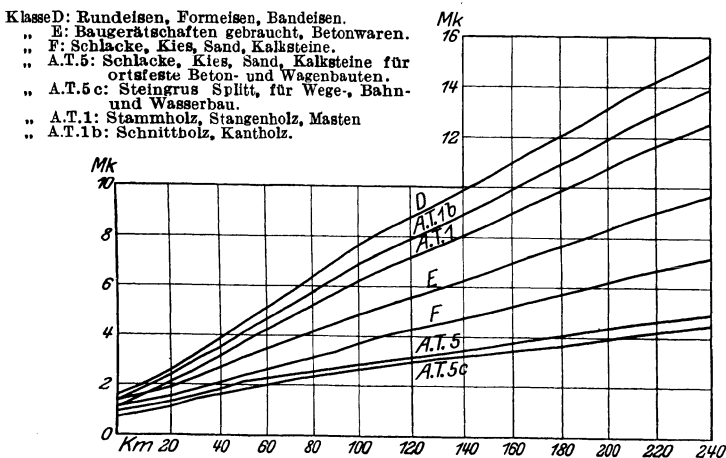
Abb. 2. Frachtkosten pro 1 t.
