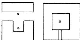
Abb. 28. Gußbetonanlagen im Hochbau bei verschiedenen Gebäudegrundrissen.
