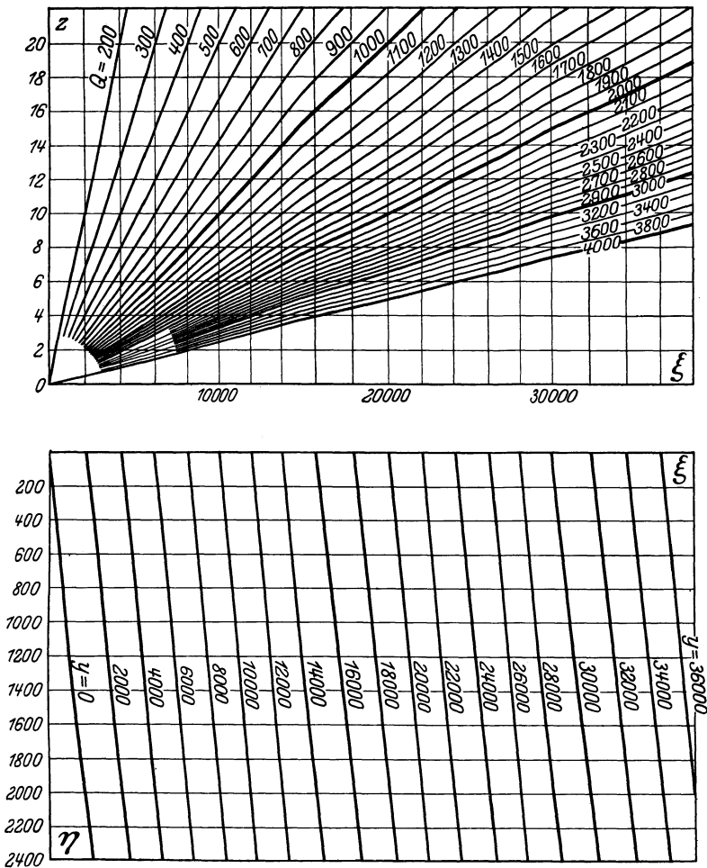
Abb. 32 b. Kostenersparnis im Gußbetonbau bei Verwendung einer 350-l-Gießmasteanlage. v = 1,0 m/Std.
