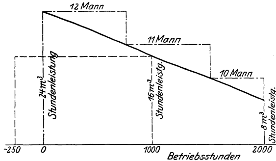
Abb. 37. Diagramm der Leistungen zur Dimensionierung von Gußbetonanlagen.
