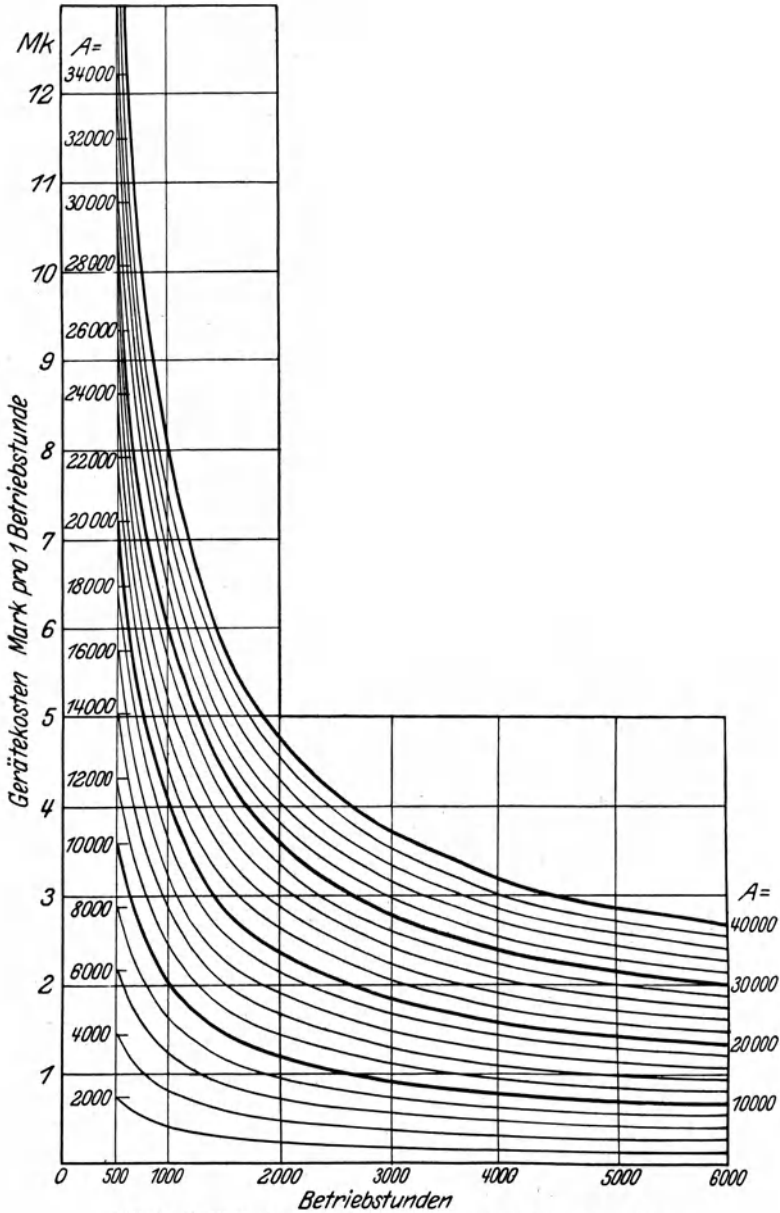
Abb. 5. Gerätekosten für den Abschreibungsgrundwert a_0 = 20\% .
