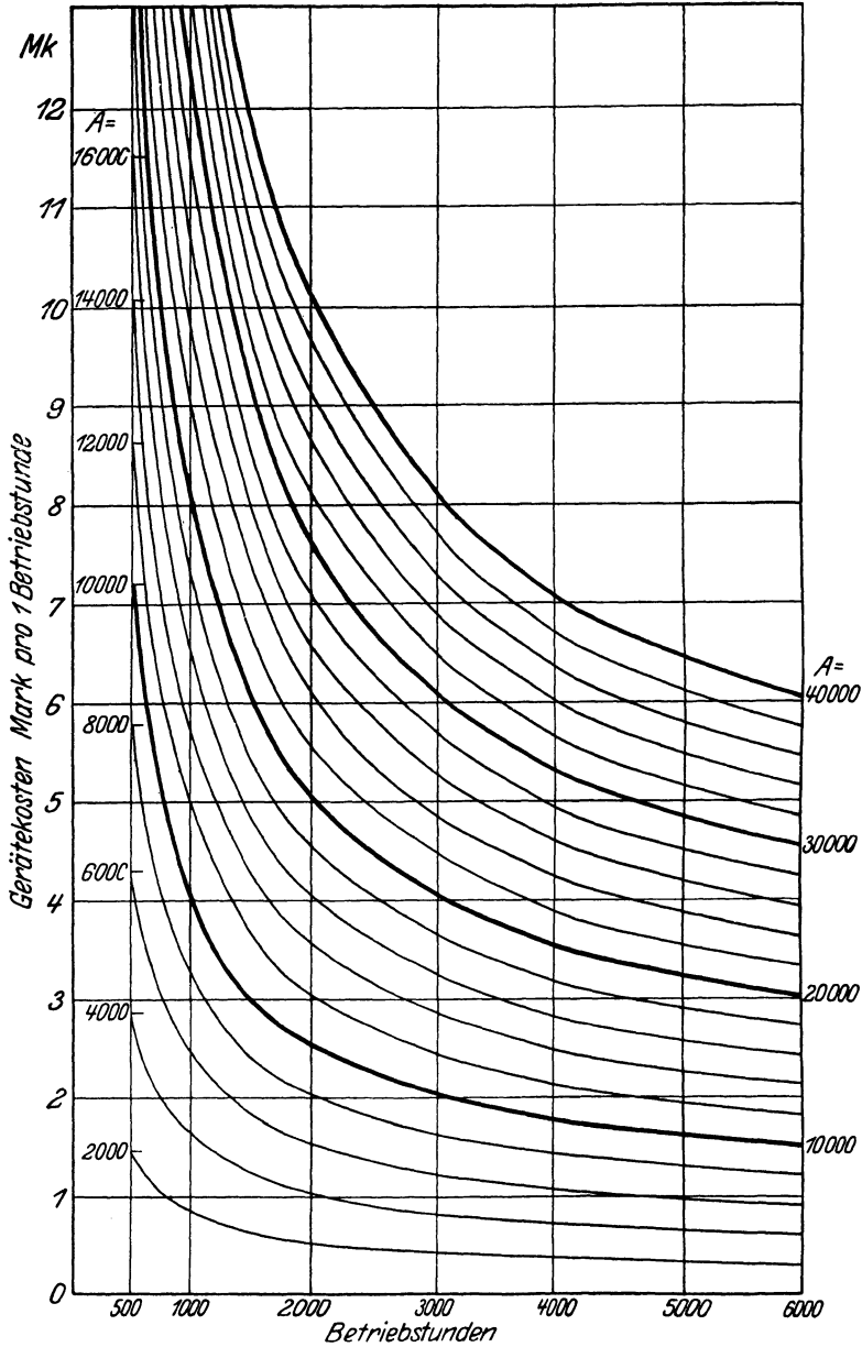
Abb. 7. Gerätekosten für den Abschreibungsgrundwert a_0 = 50\% .
