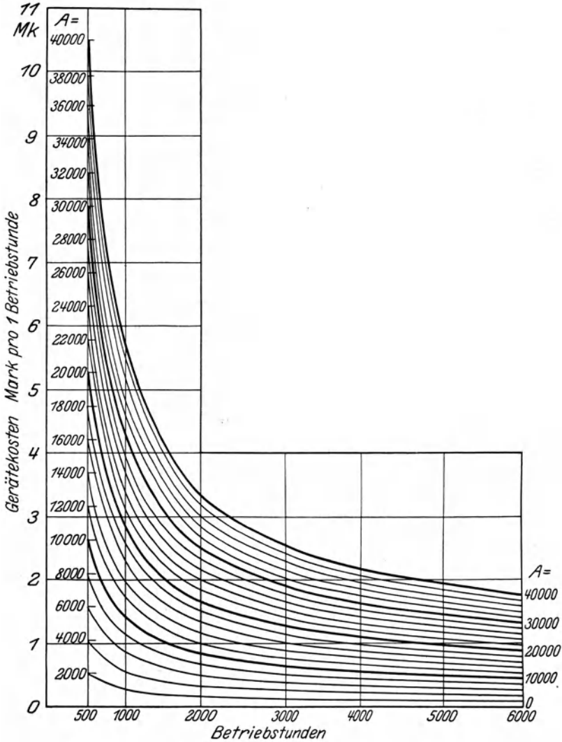
Abb. 3. Gerätekosten für den Abschreibungsgrundwert \alpha_0 = 12\% .
