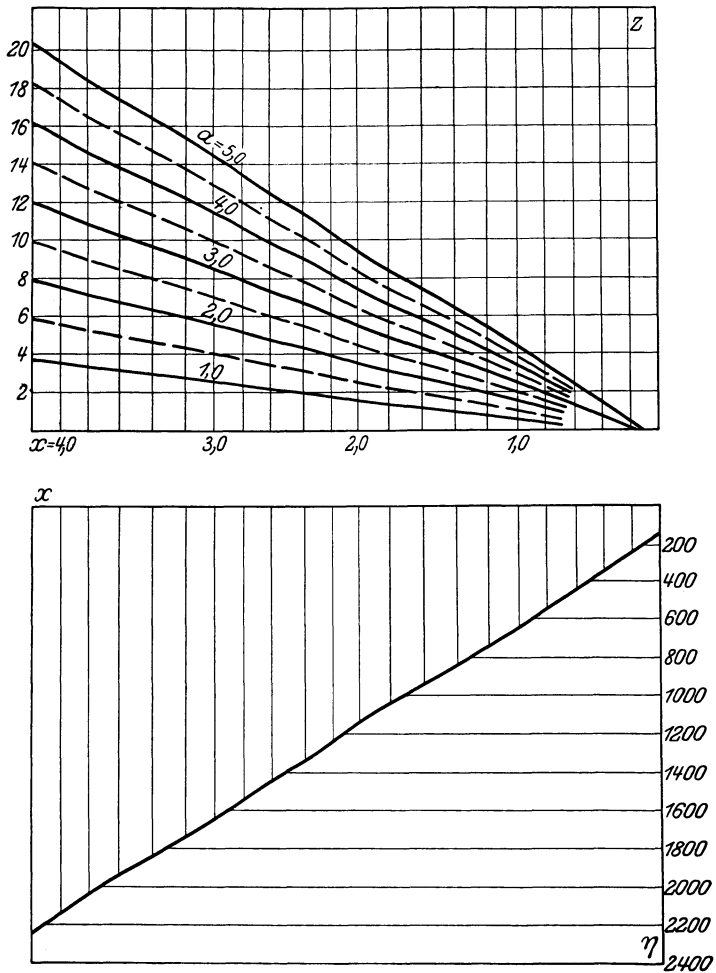
Abb. 32 a. Kostenersparnis im Gußbetonhochbau bei Verwendung einer 350-l-Gießmastanlage. v = 1,0 m/Sek.
