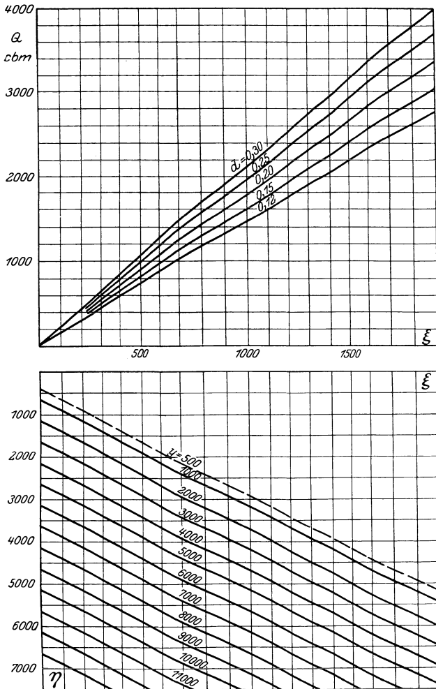
Abb. 34b. Kostenersparnis \eta im Gußbetonhochbau bei Verwendung eines 500-l-Gießturms. v = 0,5 \text{ m/Sek.}
