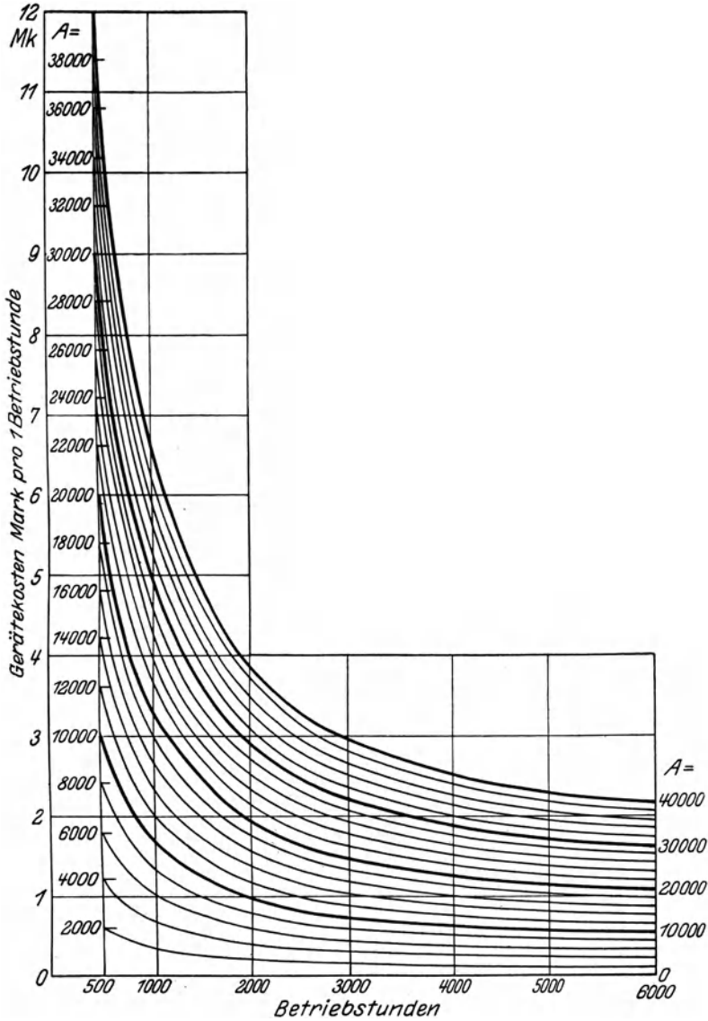
Abb. 4. Gerätekosten für den Abschreibungsgrundwert a_0 = 15\% .
