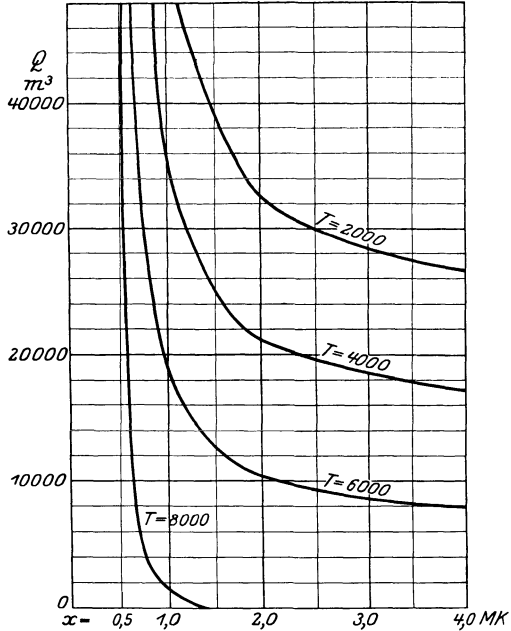
Abb. 42. Grenzbetonmengenkurven für Kabelkranbeton mit Kabelkran von 5,2 t Tragkraft und 300 m Spannweite.
