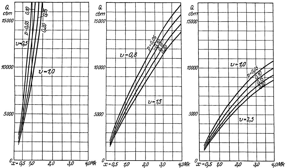
Abb. 36. Grenzbetonmengenkurven für Gießturmanlagen verschiedener Aufzugsgeschwindigkeit.
