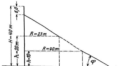
Abb. 14. Bestimmung des Arbeitsbereichs einer Gießmastanlage.
