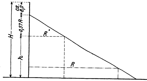
Abb. 16. Bestimmung des Arbeitsbereichs einer Gießturmanlage.
