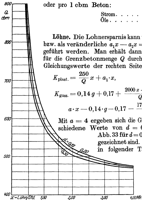
Abb. 33. Grenzbetonmengenkurven für Gußbetonhochbauten bei Verwendung einer 500-l-Gießturmanlage.
