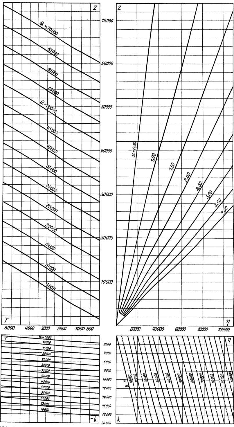
Abb. 27. Kostenersparnis \gamma bei Verwendung einer 750-l-Gießturmanlage bei Gußbetontiefbauten.
