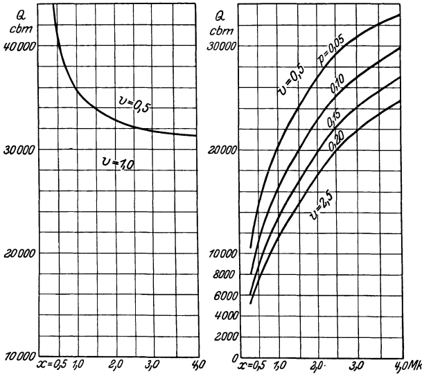
Abb. 35. Grenzbetonmengenkurven für Gießturmanlagen verschiedener Aufzugsgeschwindigkeit.
