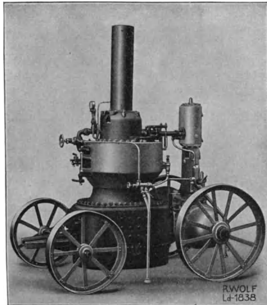
Abb. 25. Heißdampfmotorlokomobile Wolf (Magdeburg).
