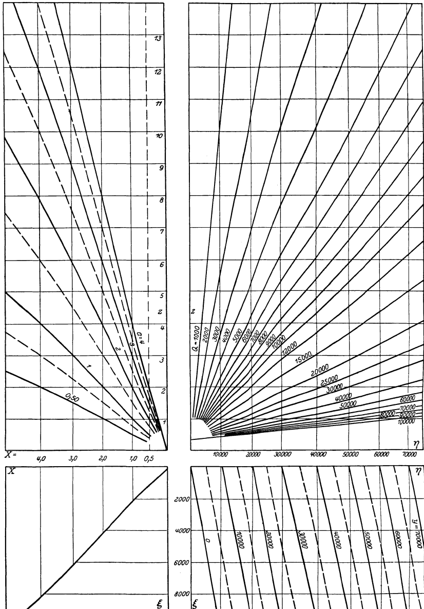
Abb. 19. Kostenersparnis y bei Verwendung einer 500-l-Gießturmanlage im Gußbetontiefbau.
