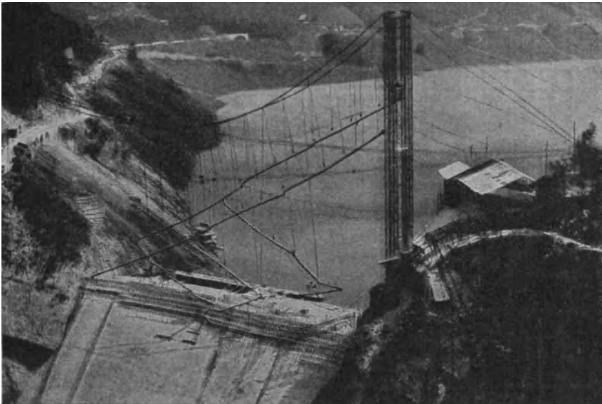
Abb. 17. Gießturmanlage an der Wäggitalsperre (Allied Machinery Co. of America, Zürich).
