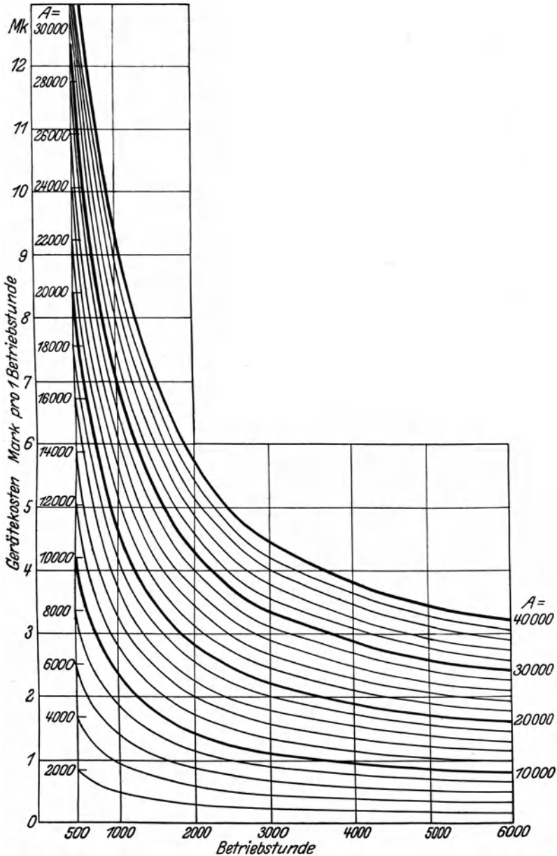
Abb. 6. Gerätekosten für den Abschreibungsgrundwert a_0 = 25\% . Baumeister, Gußbeton.
