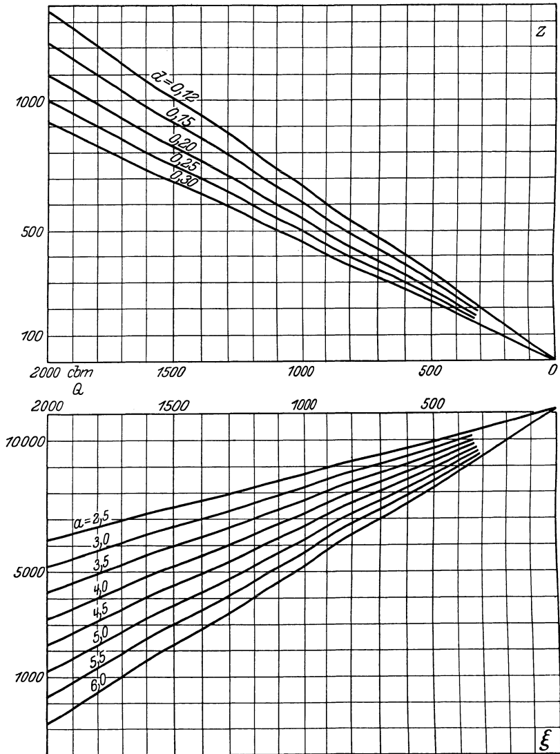
Abb. 30 a. Ersparnis \gamma im Gußbetonhochbau bei Verwendung einer 350-l-Gießmasteanlage v = 0,5 \text{ m/Sek.}
