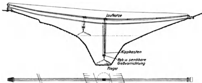
Abb. 43. Vereinigtes Kabelkran- und Gußbetonverfahren.
