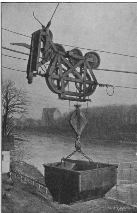
Abb. 41. Laufkatze einer Kabelbahn der Fa. Bleichert, Leipzig.
