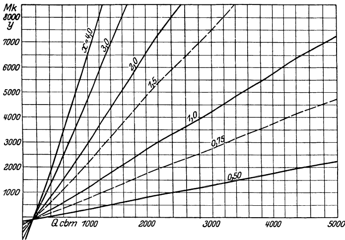
Abb. 9. Ersparnis y für Stampfbeton mit 250-l-Mischmaschine gegenüber Handmischung.
