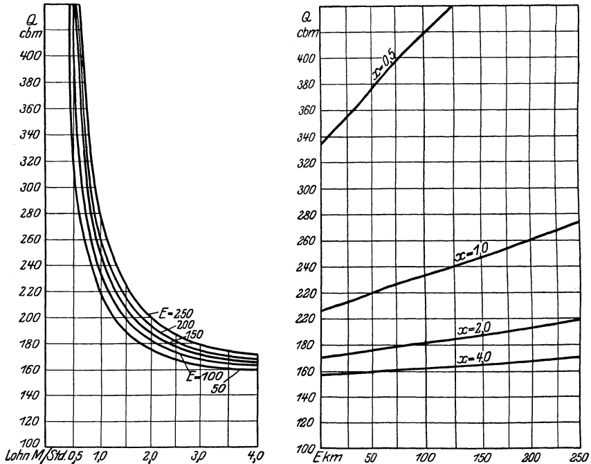
Abb. 8. Grenzbetonmengen für Stampfbeton mit 250-l-Mischmaschine gegenüber Handmischung.
