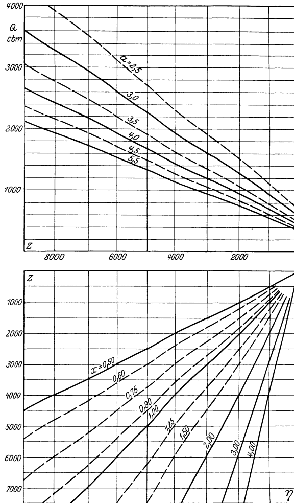
Abb. 34a. Kostenersparnis y im Gußbetonhochbau bei Verwendung eines 500-l-Gießturms. v = 0,5 \text{ m/Sek.}
