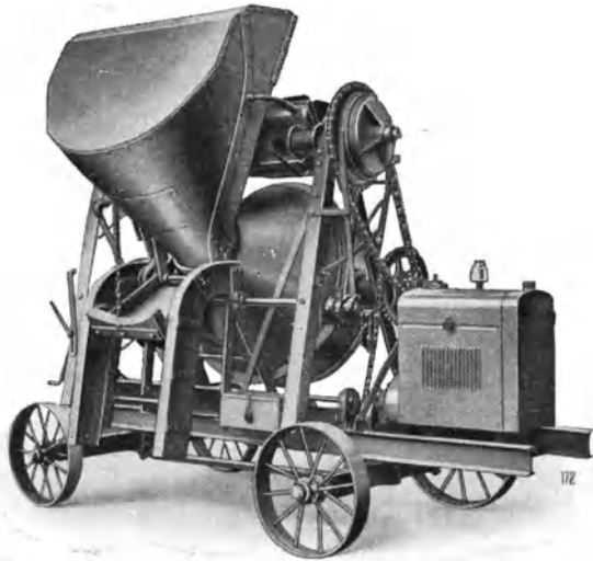
Abb. 22. Betonmischmaschine Patent Jäger der Vögele A.-G., Mannheim.
