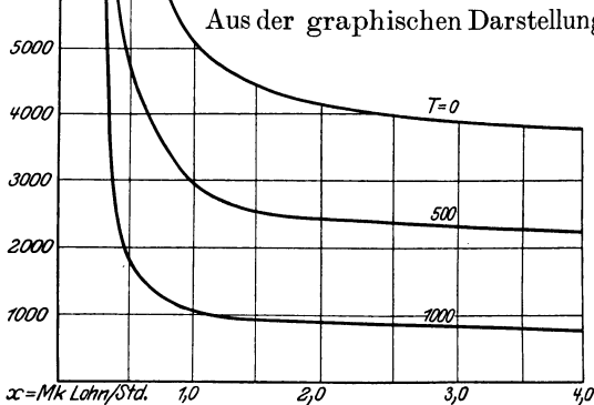
Abb. 26. Grenzbetonmengenkurve bei Verwendung einer 750-l-Gießturmanlage im Gußbetontiefbau.
