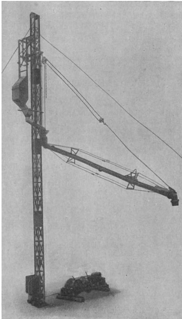
Abb. 11. Gießmastanlage 350 I (Ibag, Neustadt).
