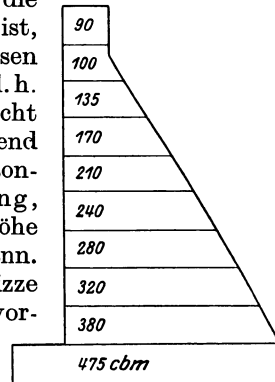
Abb. 10. Tägliche Gußleistungen bei einer Schleusenmauer.
