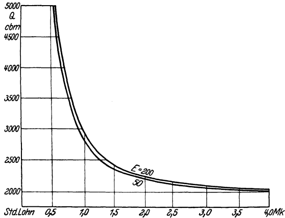
Abb. 18. Grenzbetonmengenkurven für Gußbetontiefbauten bei Verwendung einer 500-l-Gießturmanlage.
