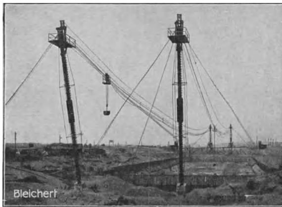
Abb. 39. Kabelkrananlage beim Bau der Schleuse I am Rheinhernekanal (Bleichert).
