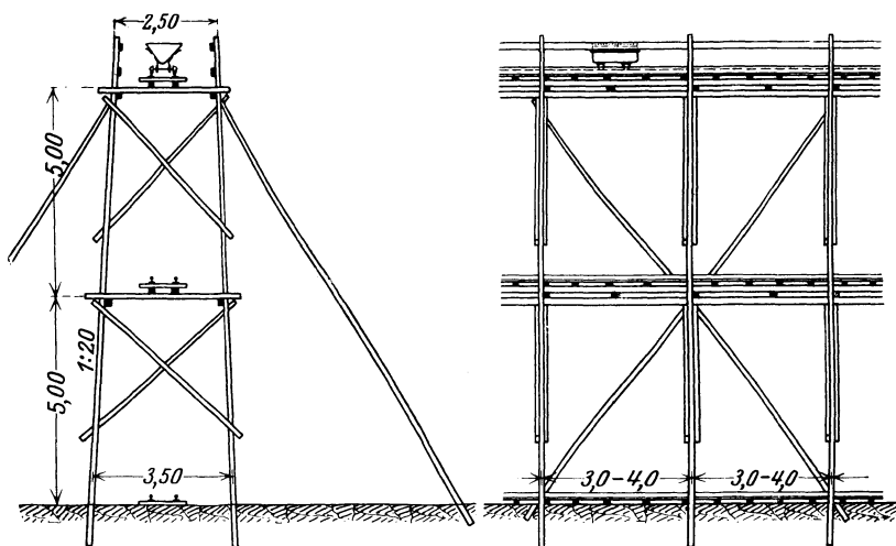
Abb. 23. Stangengerüst für den Betontransport.
