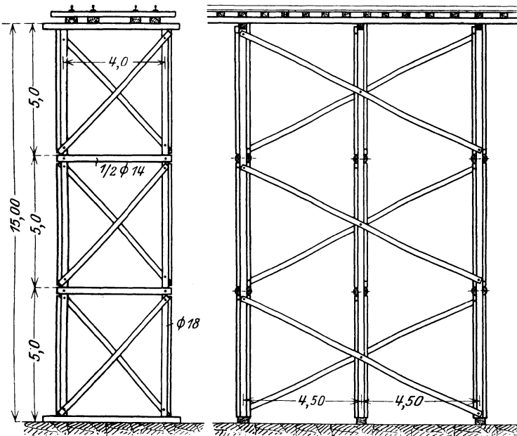
Abb. 24. Zweigleisiges Betontransportgerüst.
