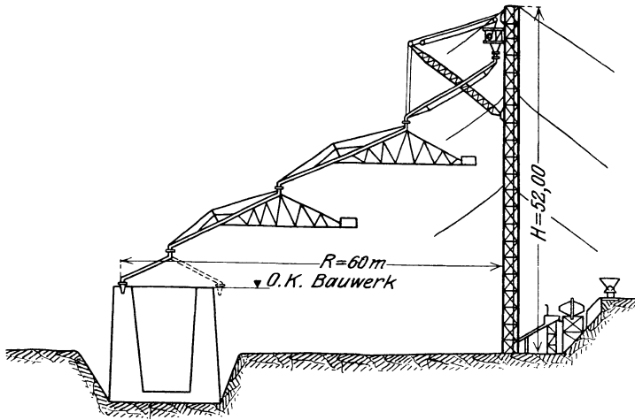
Abb. 20. 750-l-Gießturmanlage mit 60 m Arbeitsradius.
