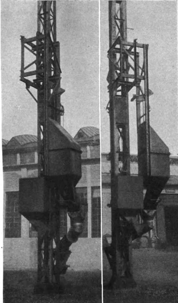
Abb. 12. Gießmasteanlage 350 l (Ibag, Neustadt).
