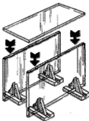
Приклеивание дна.
