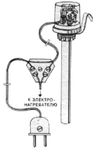
Терморегулятор РТА-3.
