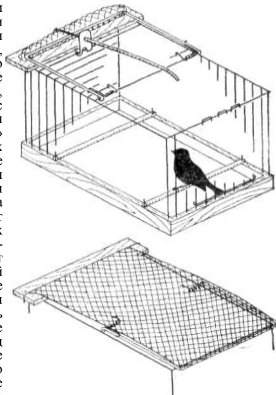
39. Лучок-самолов на клетке хорошо ловит те виды птиц, которые боятся залезать внутрь бойков. Шнуры, продетые по краям сети, сильно натягиваются в захлопнутом положении лучка.
