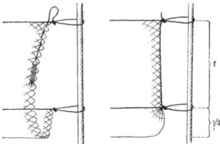
15. Боковой шнур паутинной сети крепится неподвижным узлом к каждому продольному шнуру, его длина равна расстоянию между продольными шнурами.
