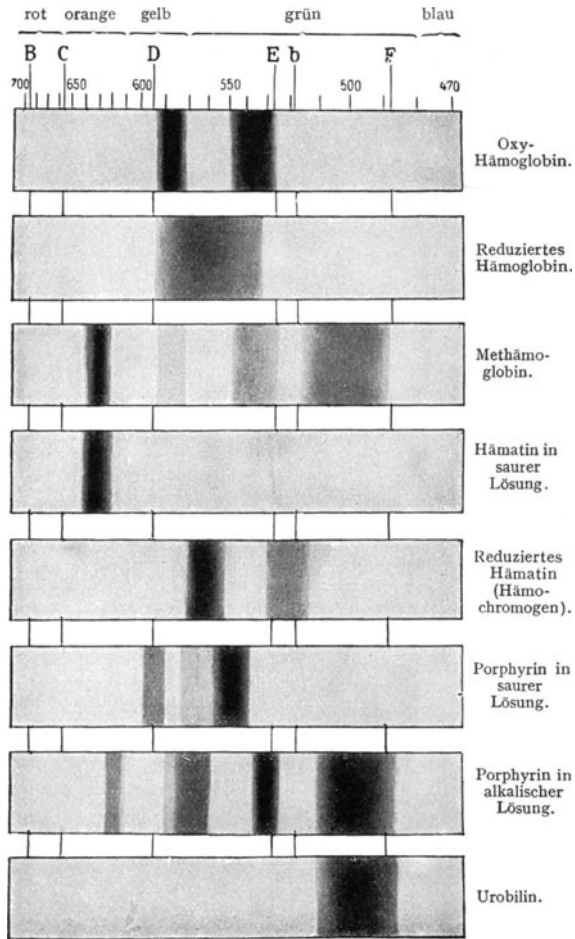
Abb 59. Spektraltafel.
