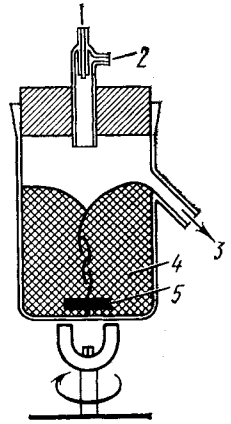
Рис. II.14. Простейшая схема аппарата непрерывного культивирования
