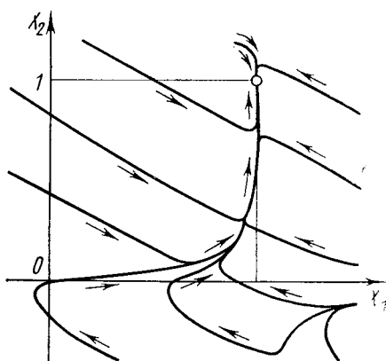
Рис. IV.10. Фазовый портрет системы (IV.3—4) при k_0 \neq 0 (световой процесс окисления: k_1=1 ; k_2=10 ; k_0=5 ; k_i=2 )
