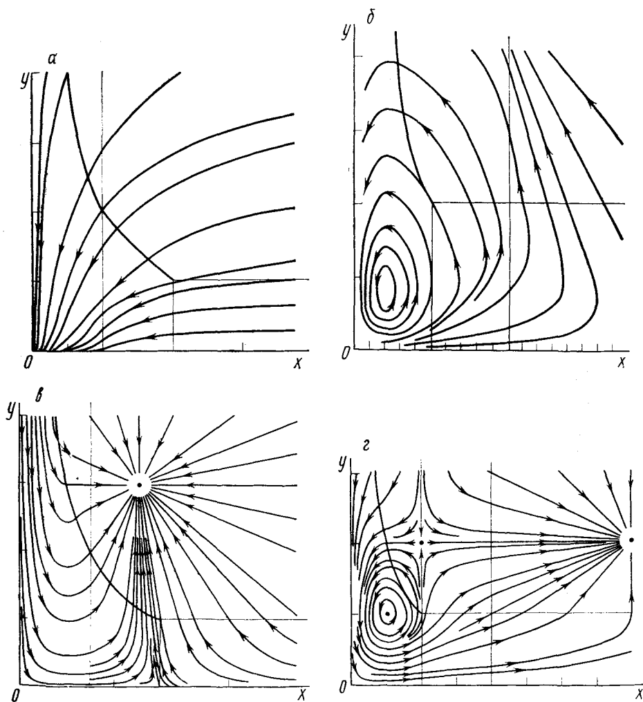
Рис. П.12. Фазовый портрет системы с лимитирующими факторами (П.8—8), описывающей взаимодействие хищника и жертвы при различных значениях параметров ( а, б, в, г ) (Поletaев, 1973а)
