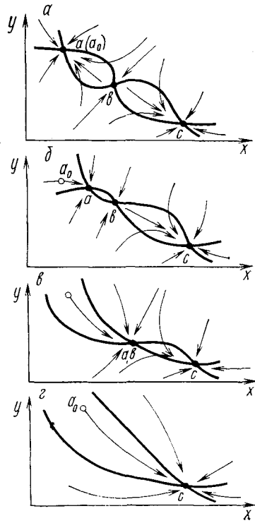
Рис. 1.30. Процесс параметрического переключения триггерной системы на фазовой плоскости ( a, б, в, г ; пояснения в тексте)
