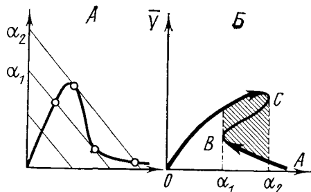
Рис. III.11. Характеристики реакции с субстратным угнетением и обратной реакцией притока субстрата в зависимости от параметра \alpha (скорости притока субстрата):
