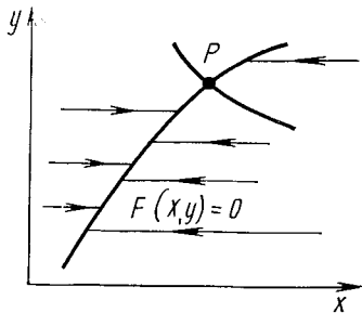
Рис. I.46. Фазовый портрет полной системы (I.9—2)
