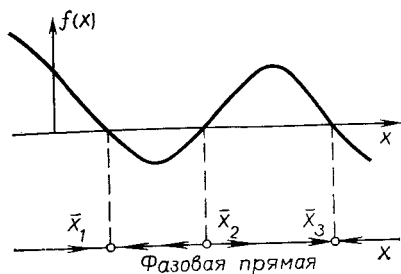
Рис. 1.4. Вспомогательная плоскость x, \dot{f}(x) для уравнения (1.2—1)
