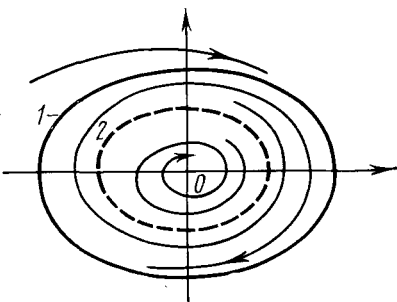
Рис. I.38. Фазовый портрет системы, имеющей устойчивый (пунктир) и неустойчивый (сплошной) предельные циклы
