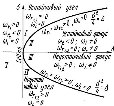
Рис. I.20. Плоскость параметров \Delta , \sigma для системы уравнений (I.4—1)
