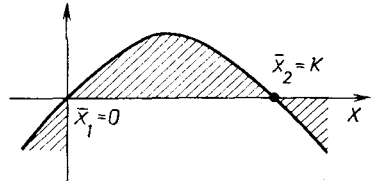
Рис. 1.7. График функции f(x) для уравнения (1.2-7)
