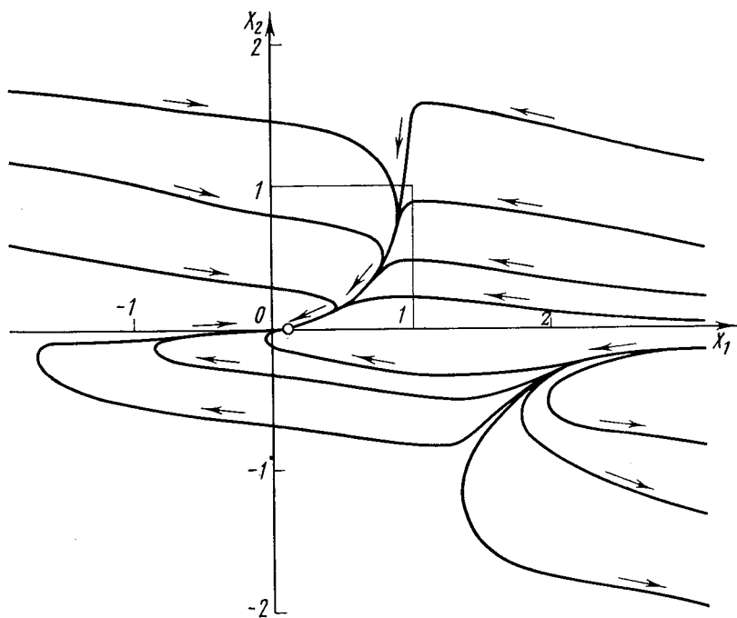
Рис. IV.10. Фазовый портрет системы (IV.3—4) при k_0 \neq 0 (световой процесс окисления: k_1=1 ; k_2=10 ; k_0=5 ; k_i=2 )
