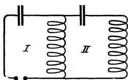
Abb. 26. Galvanische Koppelung.
