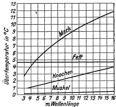
Abb. 83. Einfluß der Wellenlänge auf die Erwärmung verschiedener Gewebe nach Gebert. Zwischen 3—6 m wird die Erwärmung homogen.
