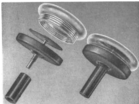
Abb. 47. Elektroden nach Schliephake (Siemens-Reiniger-Werke).
