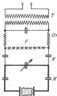
Abb. 33. Schaltbild eines Funkenstreckenapparates mit galvanischer Koppelung (Koch u. Sterzel).
