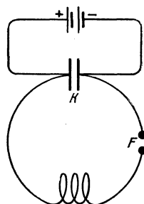
Abb. 30. Schwingungskreis mit Funkenstrecke.
