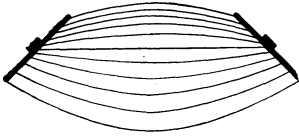
Abb. 61. Feldlinienverlauf bei geneigten Elektroden.
