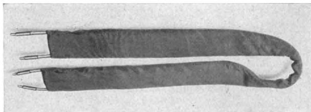
Abb. 130. Schleifenelektrode zur Hyperthermiebehandlung im Spulenfeld (Abb. 130).
