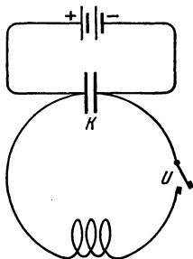
Abb. 29. Schwingungskreis mit Handunterbrecher.
