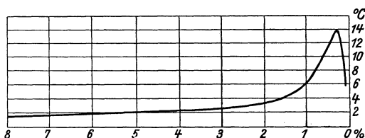
Abb. 81. Erwärmung verschieden konzentrierter Kochsalzlösungen im Felde einer 5 m-Welle.
