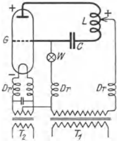
Abb. 41. Schaltbild eines Röhrenapparates.
