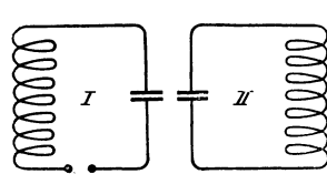
Abb. 28. Kapazitive Koppelung.
