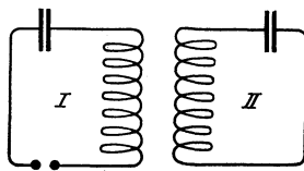
Abb. 27. Induktive Koppelung.
