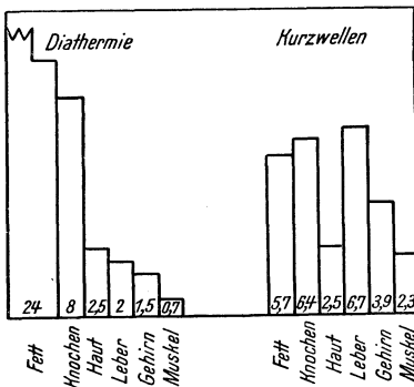
Abb. 82. Erwärmung verschiedener Gewebe durch Diathermie und Kurzwellen (3 m-Welle) nach Schliephake.
