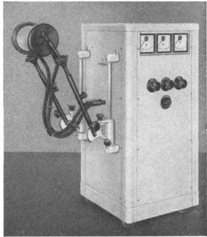
Abb. 45. Kurzwellenapparat für 1 m Wellenlänge und 700 Watt Leistung (Siemens-Reiniger-Werke).
