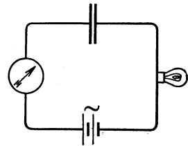
Abb. 7. Ein Kondensator in einem Wechselstromkreis bedeutet keine Unterbrechung, sondern nur einen Widerstand (kapazitiver Widerstand).
