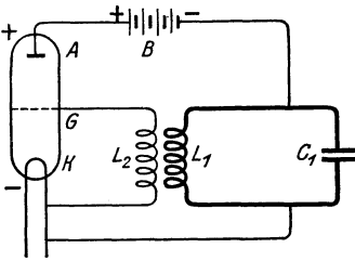
Abb. 40. Die Dreielektrodenröhre als Schwingungserreger.
