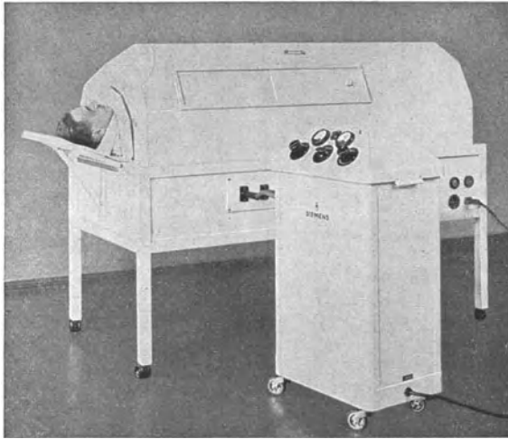
Abb. 132. Behandlung in der Fieberkabine (Siemens-Reiniger-Werke).
