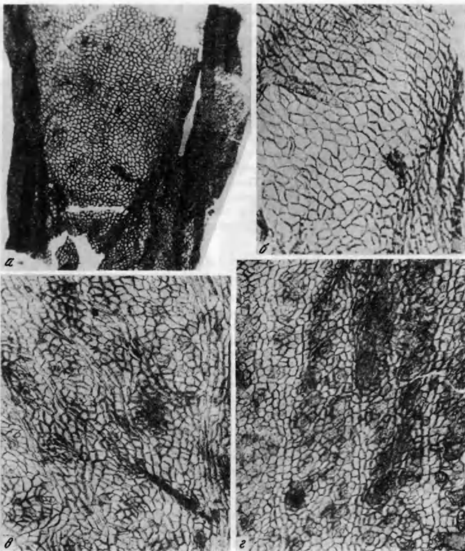
Рис. 24. Peltaspermopsis ? sp. AVG-3 (а, б) и Tatarina olferievii S. Meyen (в, г): а — верхняя эпидерма одного сектора, преп. N 3773/1534-A пункт 1, \times 50 ; б — эпидерма ножки с беспорядочным расположением клеток, преп. N 3773/1649-С, пункт 2, \times 100 ; в, г — голотип, преп. N 3765/93и-37д, \times 50 ; в — нижняя эпидерма, г — верхняя эпидерма; Вязовка (а, б), Луптюг (в, г)
