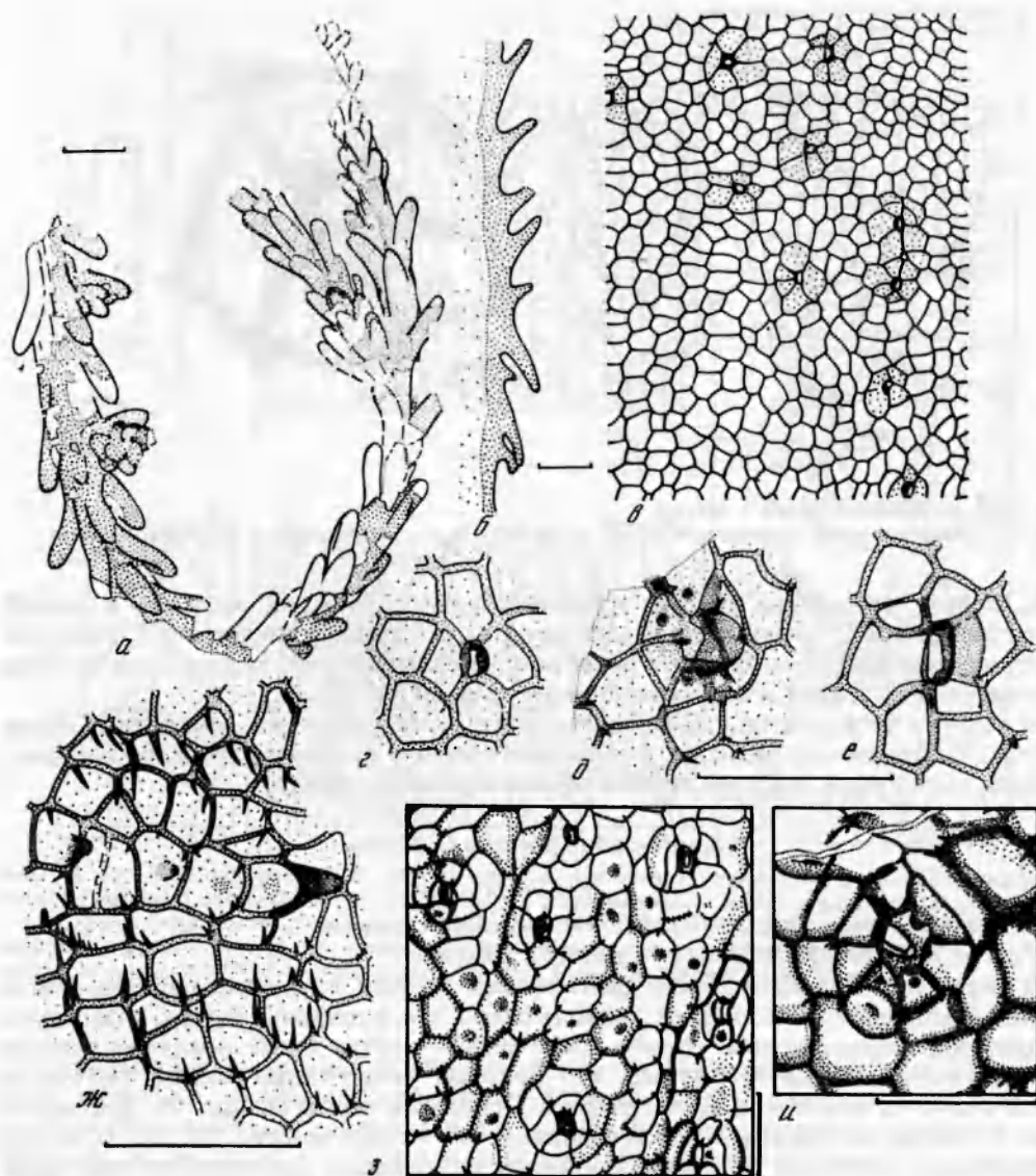
Рис. 72. Quadrocladus dvinensis S. Meyen:
