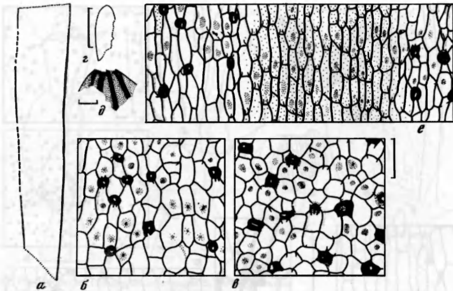
Рис. 53. Phylladoderma (Aequistomia) annulata sp. nov.:
