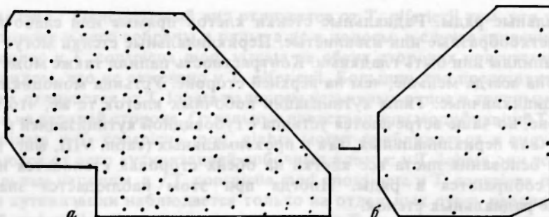
Рис. 37. Распределение устьиц у Tatarina conspicua mod. virgata , прен. N 3765/91-1: а — верхняя эпидерма; б — нижняя эпидерма; длина линейки 500 мкм; Луптюг
