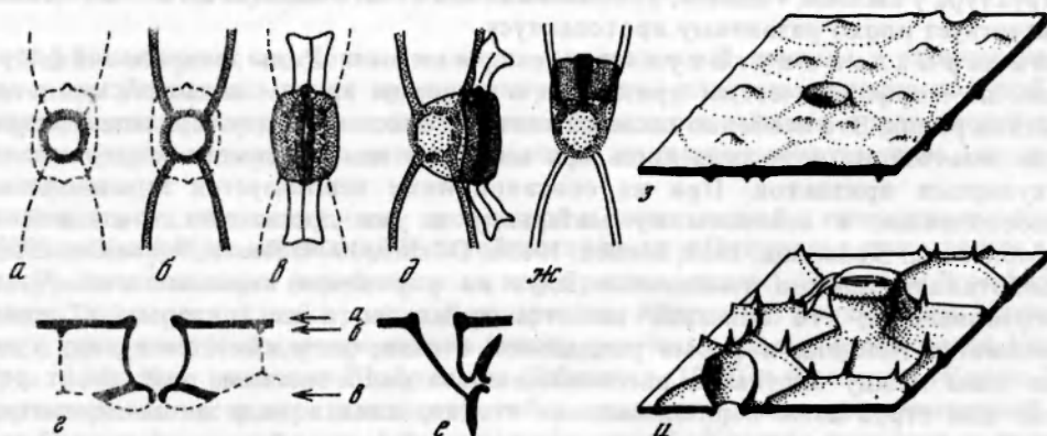
Рис. 14. Погруженные устьица Aequistomia (схематическое изображение кутикулы):
