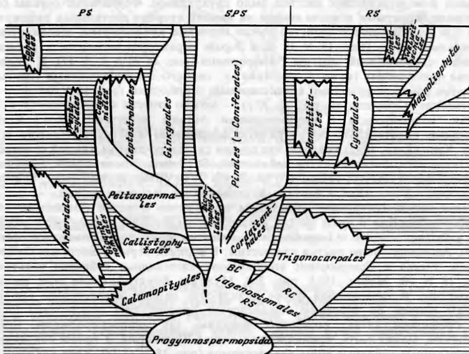
Рис. 16. Филогенетические отношения основных групп голосеменных:
