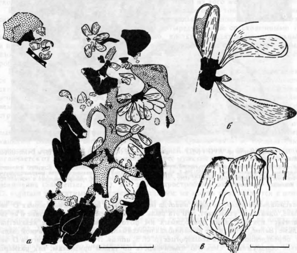
Рис. 70. Dvinostrobos sagittalis sp. nov., голотип N 4552/494-1:
