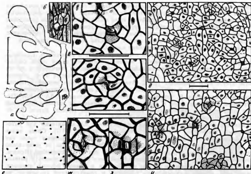
Рис. 62. Rhabdopteria antiqua sp. nov., голотип (а) и эпидермальное строение его рахиса (б), нижней (с—д) и верхней (е—и) сторон листа:
