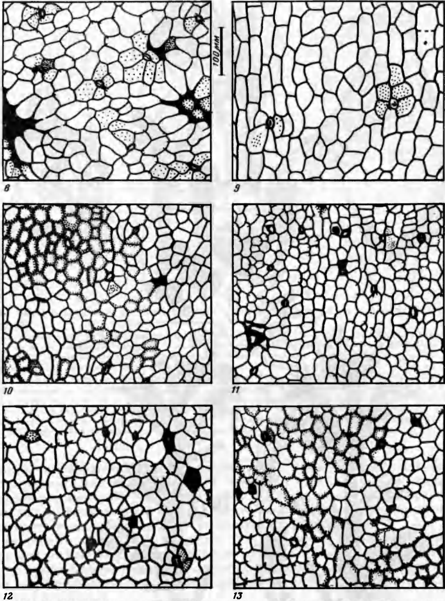
Рис. 69. Sashinia borealis S. Meyen, голотип:
