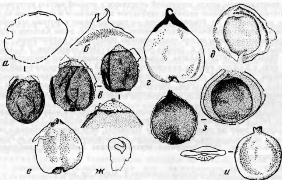
Рис. 45. Salpingocarpus bicornutus sp. nov., отпечатки, мацерированные фитолеймы и немацерированная фитолейма (u), на мацерированных фитолеймах мегаспоровая мембрана, нуцеллюс и интегумент показаны точками разной густоты, фитолейма на отпечатках зачернена:
