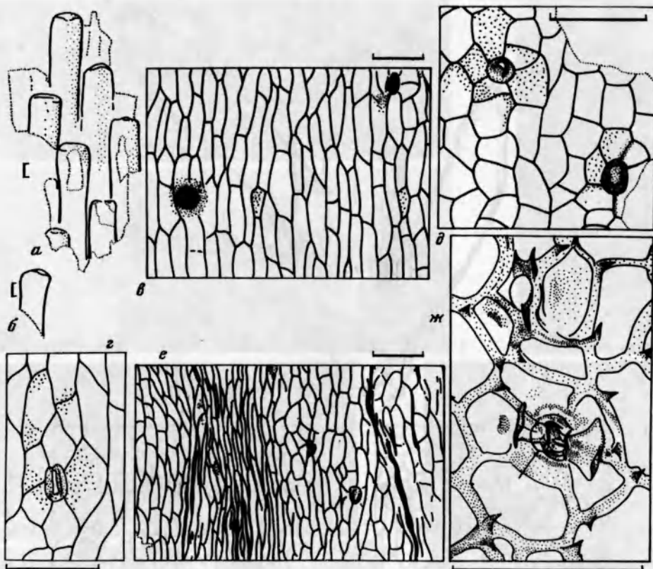
Рис. 74. Quadrocladus borealis S. Meyen, кора с листовыми подушками (а, б), эпидермальное строение листовой подушки (в—г), устьица листа с сохранившимися замыкающими клетками (ж):
