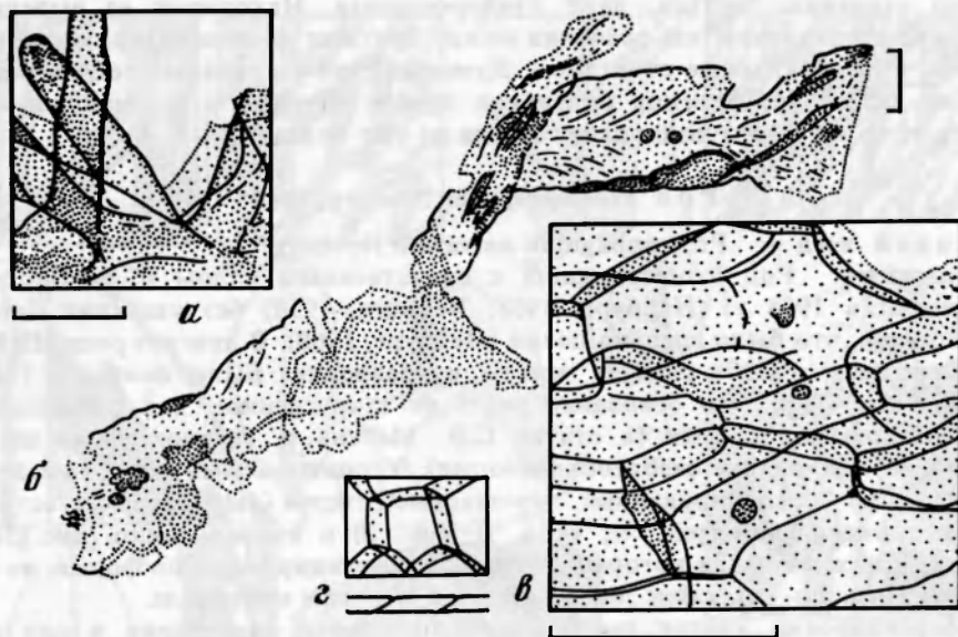
Рис. 4. Pelliiothallites tataricus sp. nov.:
