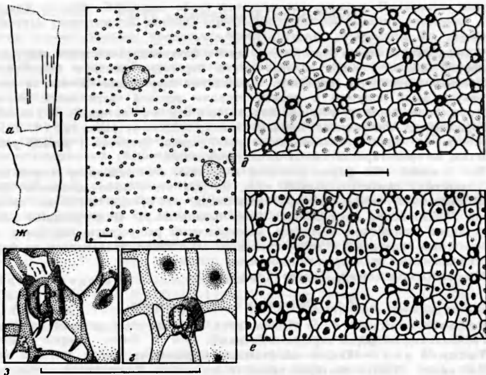
Рис. 57. Phylladoderma (Aequistoma) tatarica sp. nov., голотип (а—е) и паратип (ж, з):
