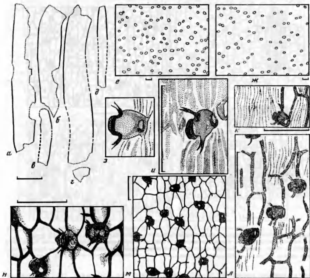
Рис. 54. Phylladoderma (Acquistomia) rastorguevii sp. nov., паратипы (а—в, д) и голотип (з, е—н): а — экз. N 3981/47-15; б — экз. N 3981/47в-11; в — экз. N 3981/55-6; з — голотип N 3981/64в-3; д — экз. N 3981/55-7; е, ж — распределение устьиц на верхней (е) и нижней (ж) сторонах листа, преп. N 3981/64-3, пункты 2 и 1; з—л — устьица и ребристость кутикулы нижней стороны листа, тот же преп., пункт 1 (см. табл. XIII, фиг. 4); м, н — верхняя эпидерма, тот же преп., пункты 5 и 3; длина линейки — 1 см (а—з), 100 мкм (д—ж); Исады
