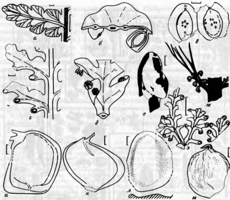
Рис. 17. Представители Calamopityales (а—д) и примитивных Peltaspermales (е—м):
