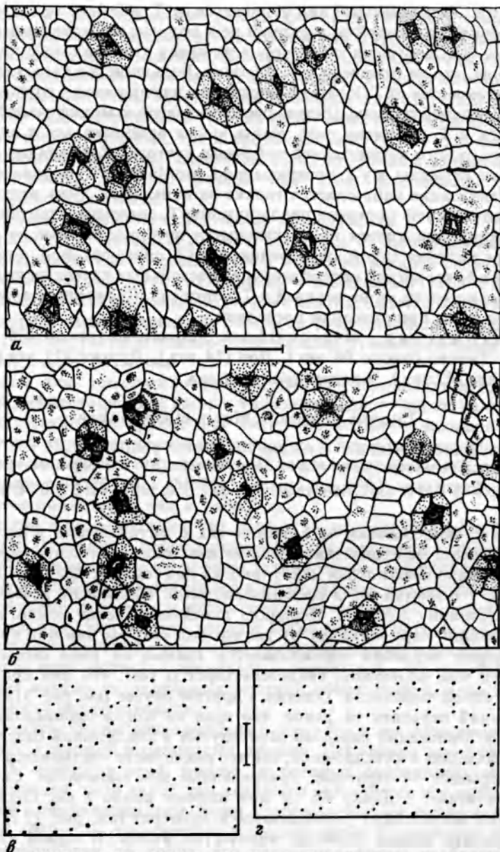
Рис. 38. Tatarina pinnata S. Meyen et Gomankov, голотип, преп. N 4552/466:
