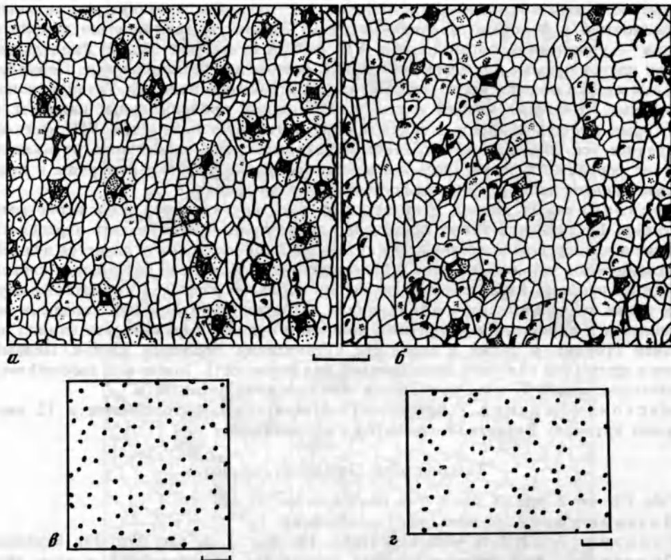
Рис. 39. Tatarina mira sp. nov., голотип, преп. N 4388/62-1:
