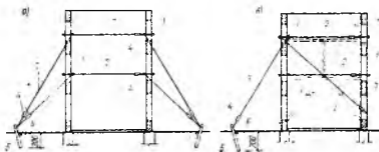
Рис. 16. Крепление стен растяжками
