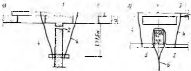
Рис. 18. Крепление отклонившихся или выпучившихся стен доутами-скрутками а — к поперечной стене; б — к колонне; 1 — простенок; 2 — трещина; 3 — поперечина диаметром 10—15 см; 4 — проволоочная скрутка диаметром 5—6 мм; 5 — колонна; 6 — растяжка или расчалка диаметром 16 мм
