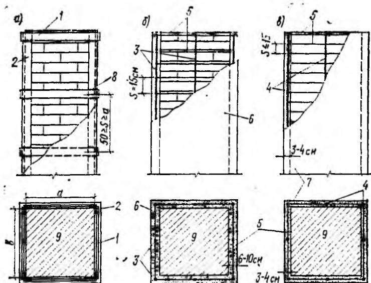
Рис. 1. Схема усиления поврежденных простенков и столбов обоями а — стальной; б — железобетонной; в — армированной раствором; 1 — l(x) планки 35×5—60×12 мм; 2 — уголки; 3 — стержни диаметром 5—12 мм; 4 — стержни диаметром 6—12 мм; 5 — хомуты диаметром 4—10 мм; 6 — бетон марки М 150—200; 7 — раствор марки 75—100; 8 — сварга; 9 — кладка
