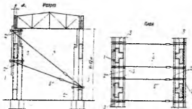
Рис. 15. Крепление отклонившейся или выпучившейся стены стальными стяжками (расчалками)
