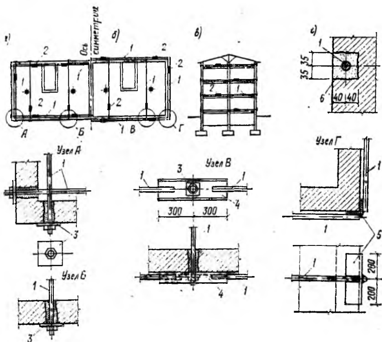
Рис. 6. Крепление стен металлическими тяжами в уровне перекрытий а — внутри здания; б — снаружи здания; в — разрез; г — вариант укладки тяжей в штрабу; 1 — тяж; 2 — муфта натяжения; 3 — металлическая подкладка; 4 — швеллер № 16—20; 5 — уголок; 6 — цементный раствор марки 100
