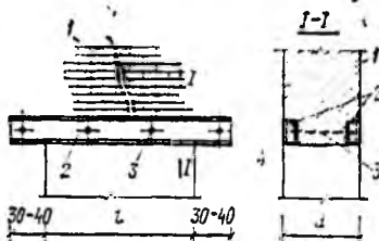
Рис. 10. Усиление рядовых и клинчатых перемычек
