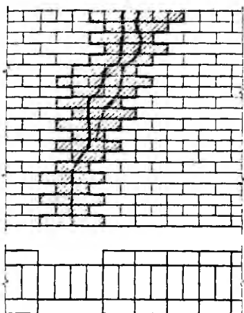
Рис. 9. Заделка трещин с разборкой старой кладки
