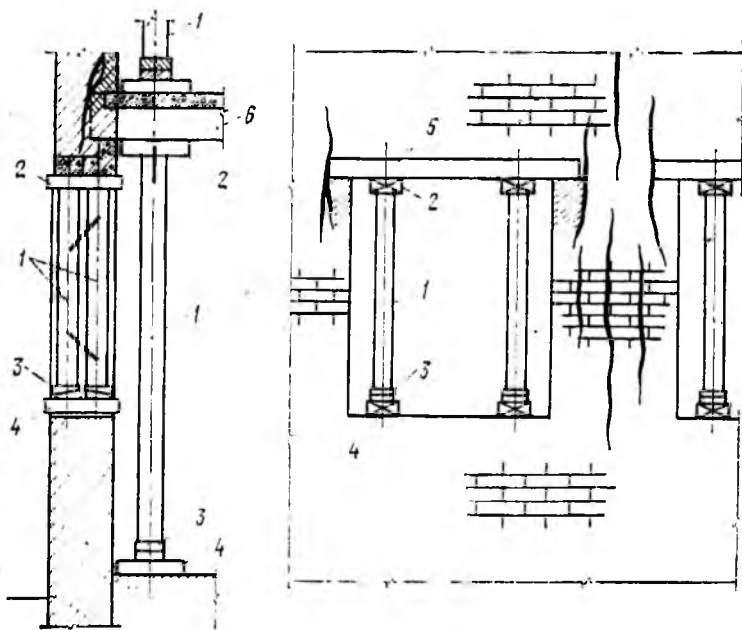
Рис. 5. Укрепление и разгрузка от массы перекрытий поврежденных простенков стойками
