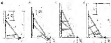
Рис. 14. Схемы крепления отклонившихся и выпучившихся стен подкосами а, б — при высоте стен до 6 м; в, г — при высоте стен 6—12 м; 1 — подкосы диаметром 16—20 см; 2 — подкладка диаметром 16—20 см; 3 — стойка диа- метром 16—20 см; 4 — свастики; 5 — лежень диаметром 18—22 см; 6 — клинья; 7 — подкладка; 8 — упорный столб диаметром 18—22 см; 9 — штырь
