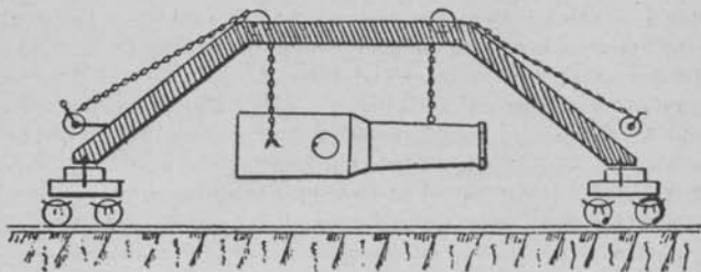
FIG. 12.—Carrier.
