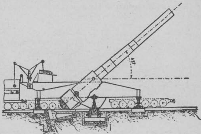
FIG. 7.—340-mm. gun.
