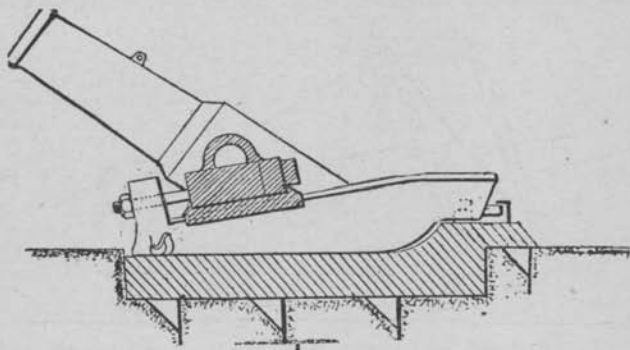
FIG. 11.—Filloux 370-mm. mortar.
