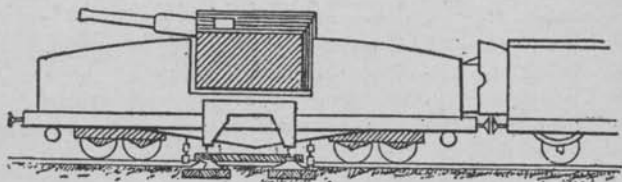
FIG. 1.—19-cm. gun, 1870-1893 model.
