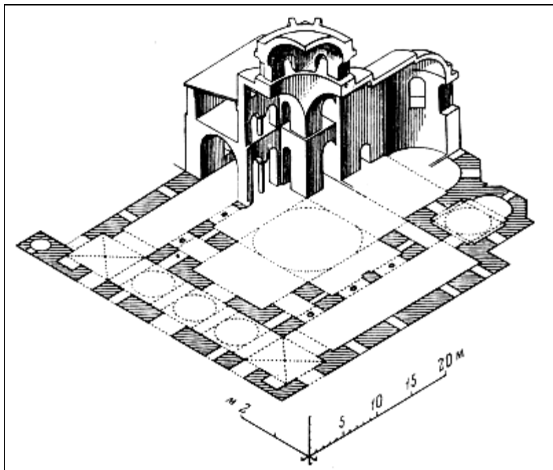
План и разрез церкви св. Софии в Фессалонике
