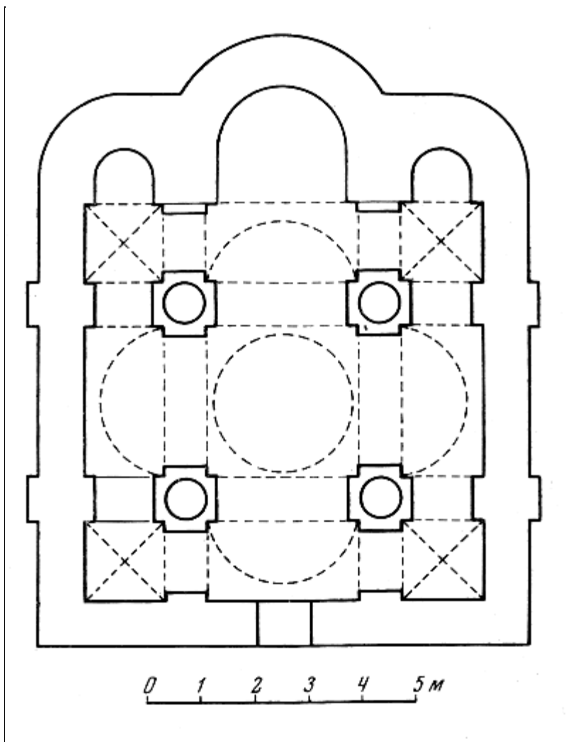
План церкви Иоанна Предтечи в Керчи
