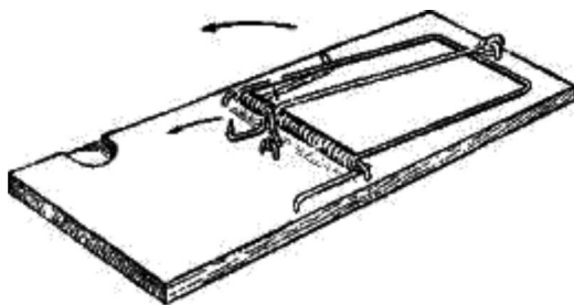
Рис. 39. Давилка Геро (из Ралля).
