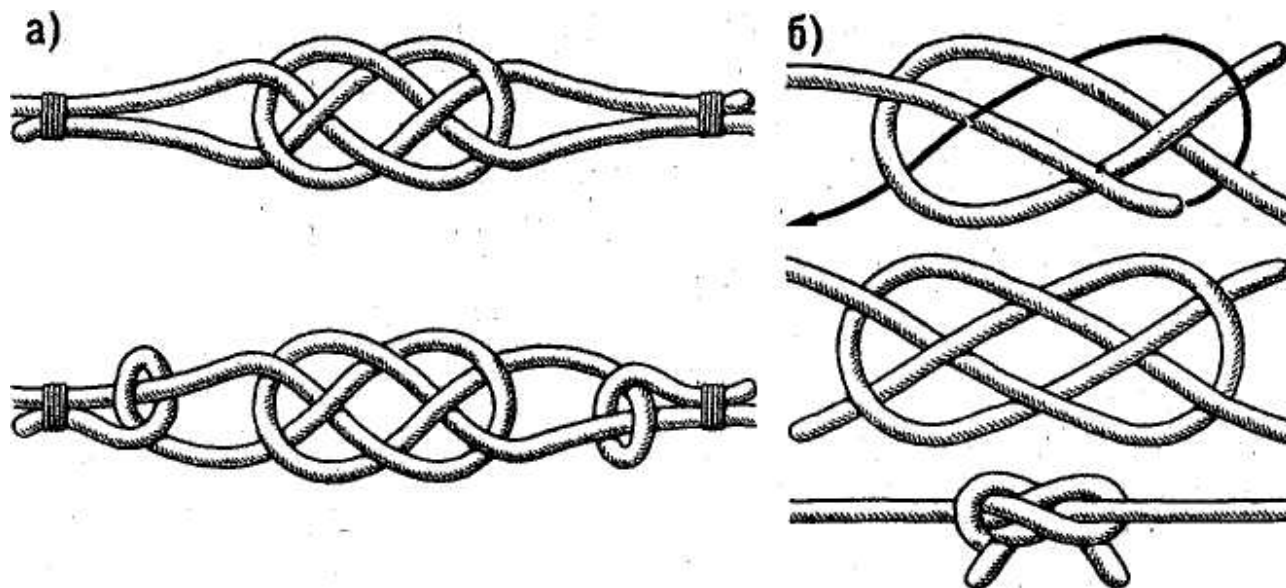
▲ Рис. 29. Плоский узел: a — первый способ вязки; б — второй способ вязки
