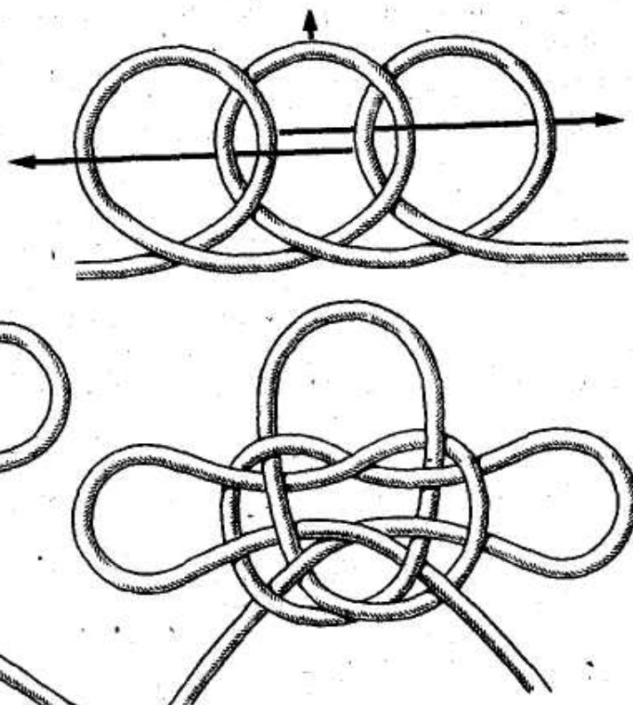
Рис. 80. Топовый узел
