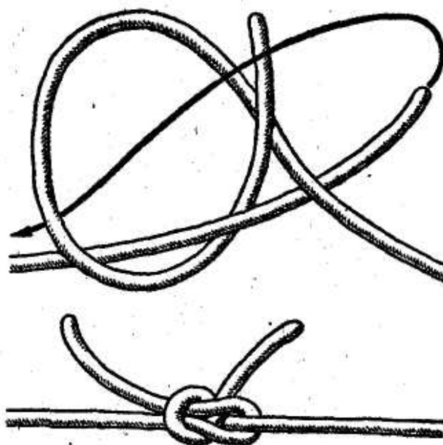
Рис. 35. Ткацкий узел
