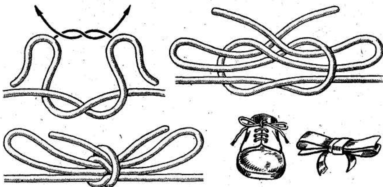
Рис. 95. Двойной рифовый узел
