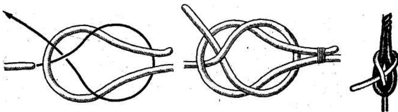
Рис. 38. Шкотовый узел
