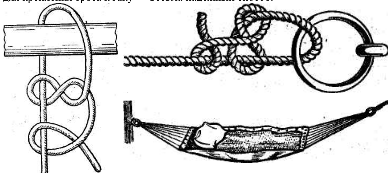
Рис. 11. Кочный штык
