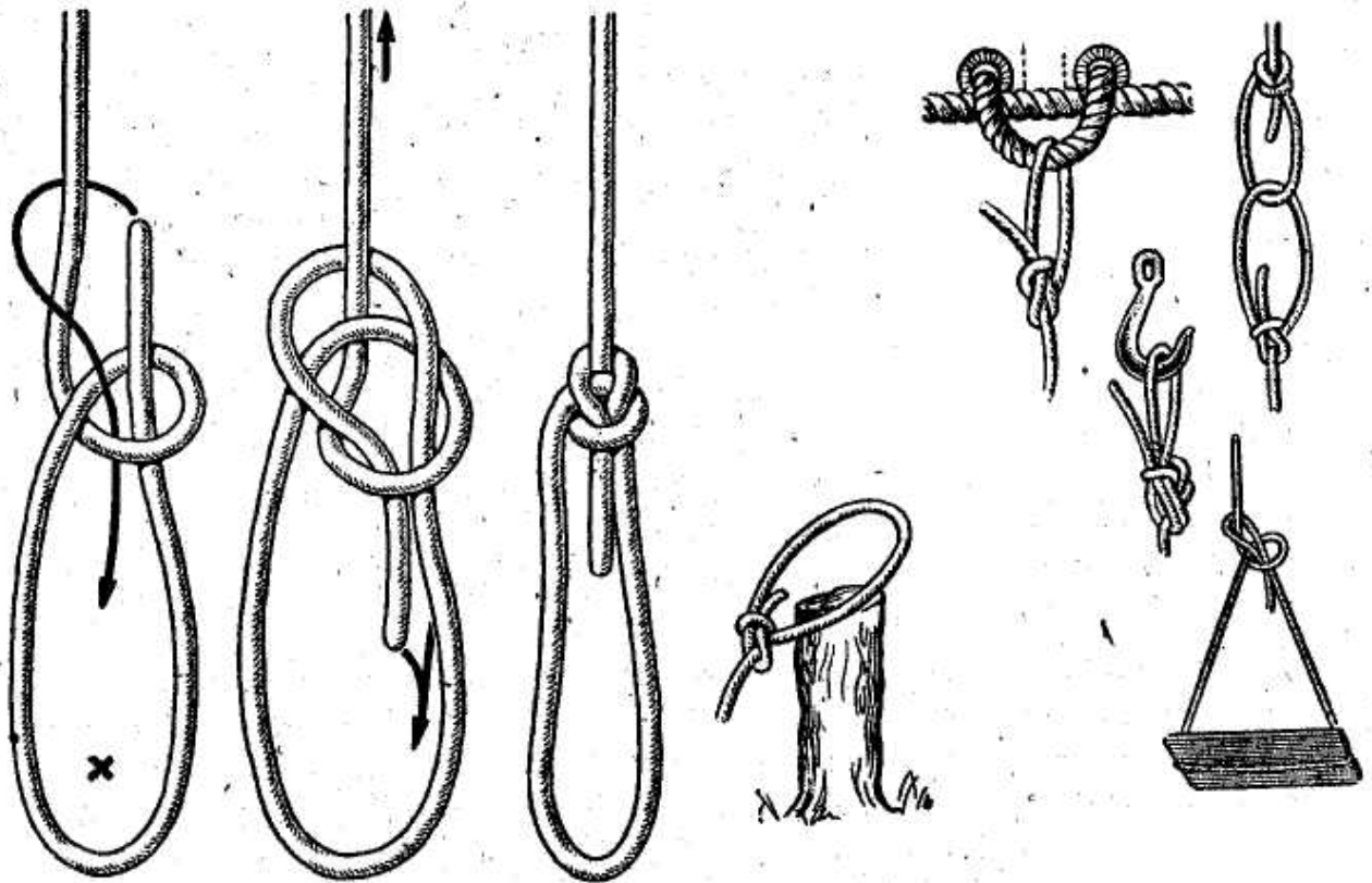
▲ Рис. 76. Беседочный узел
