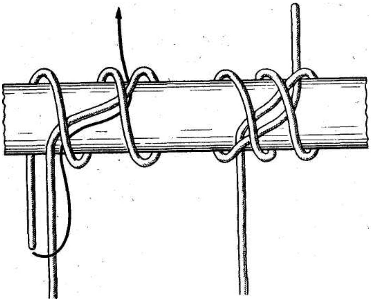
Рис. 51. Двойной «констриктор»
