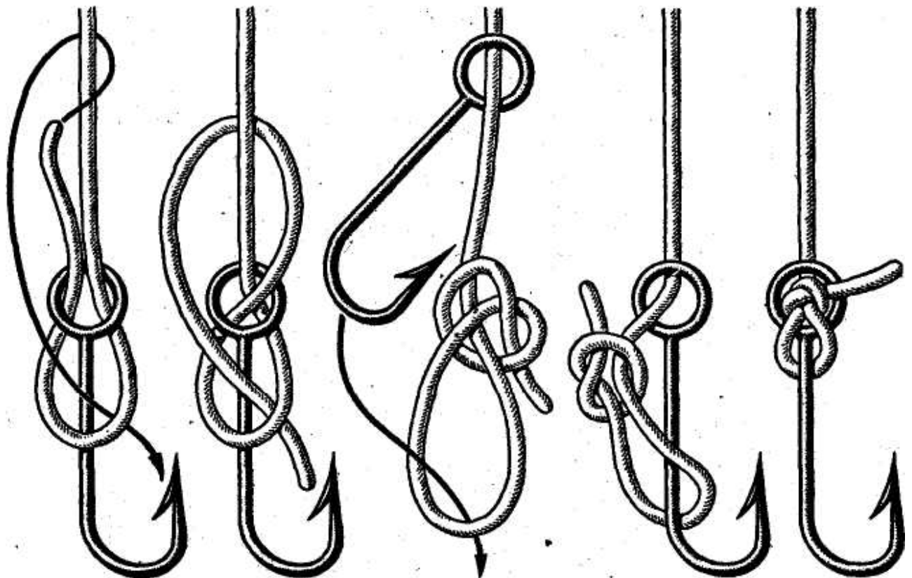
Рис. 122. Рыбацкая восьмерка
