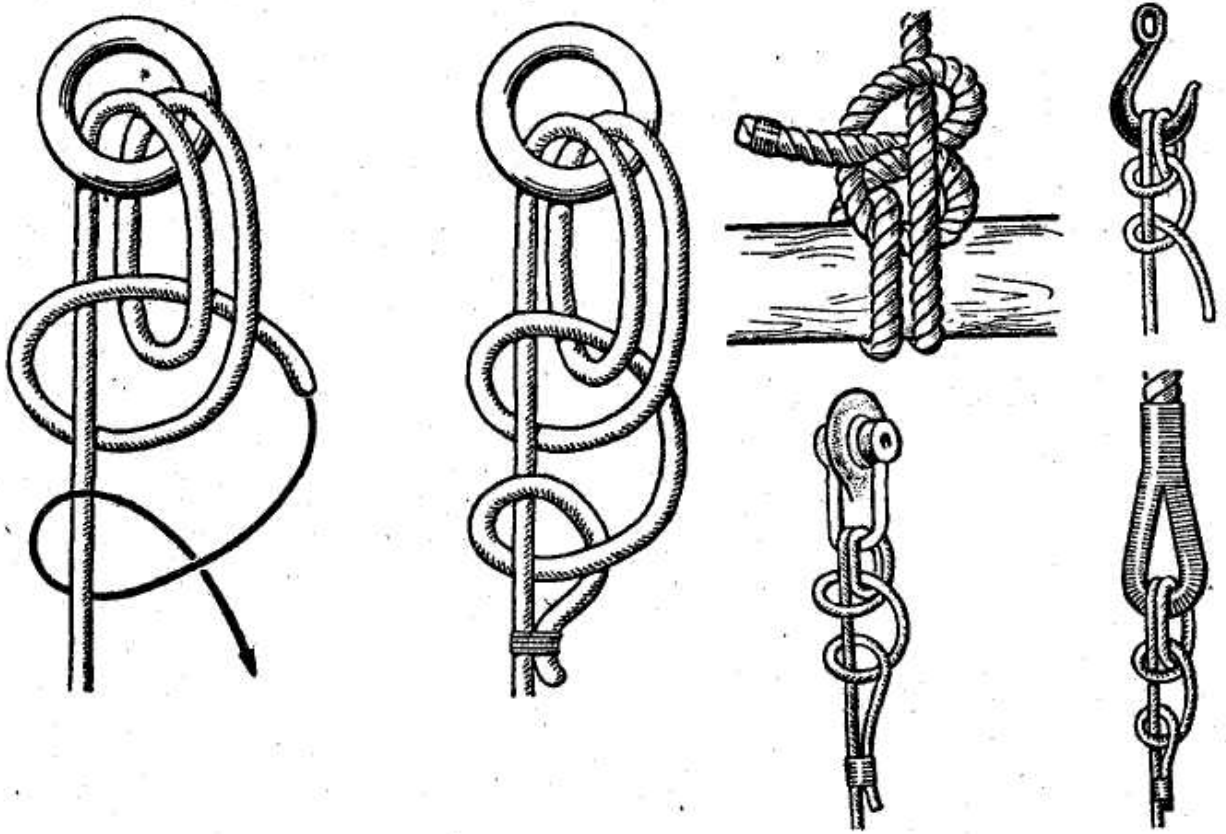
▲ Рис. 15. Рыбацкий штык (якорный узел)
