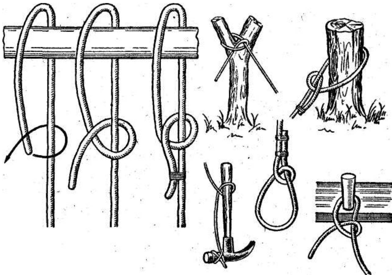
Рис. 9. Простой полуштык
