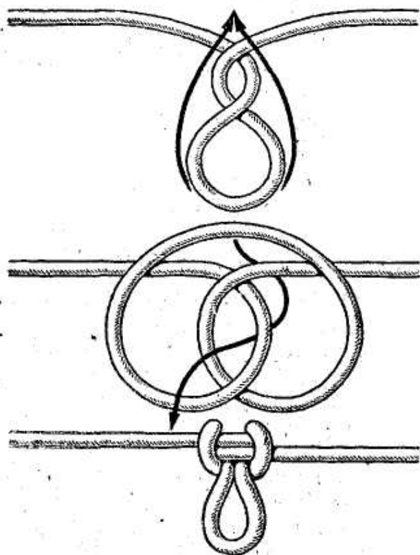
Рис. 74. Ездовая петля
