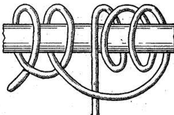
Рис. 59. Верблюжий узел
