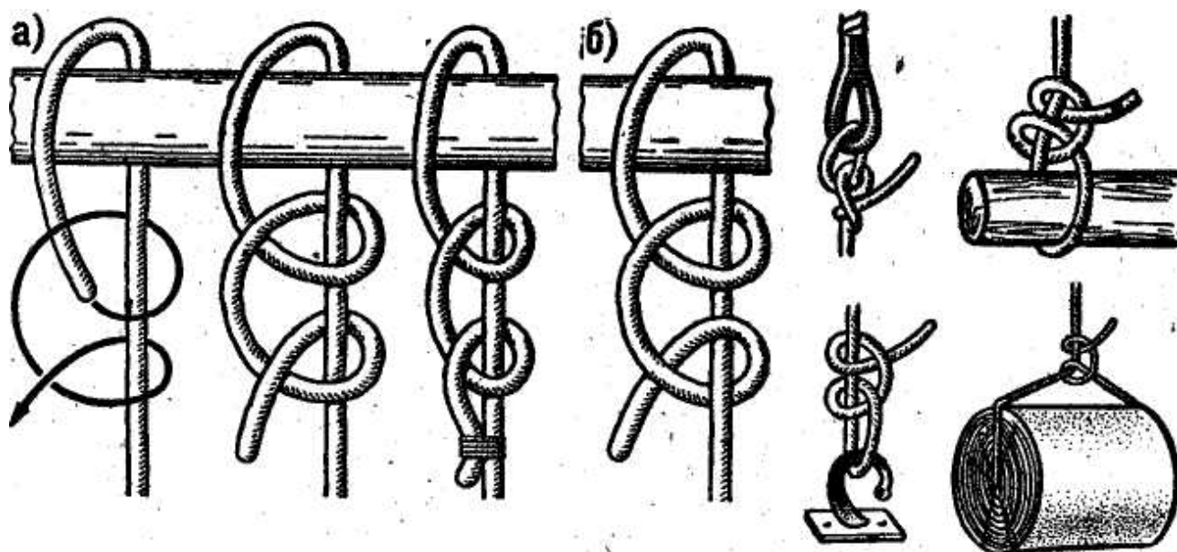
Рис. 10. Простой штык: а - правильно завязанный; б — перевернутый (неправильный)
