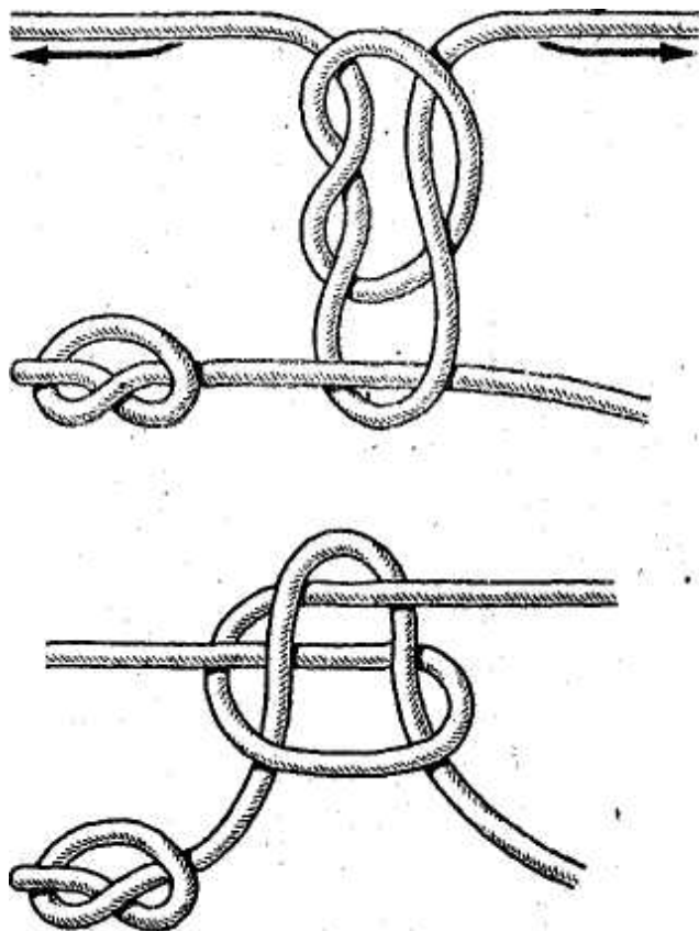
Рис. 131. Поводковый на основе бегущего узла
