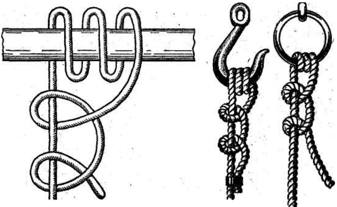
Рис. 13. Простой штык с двумя шлагами
