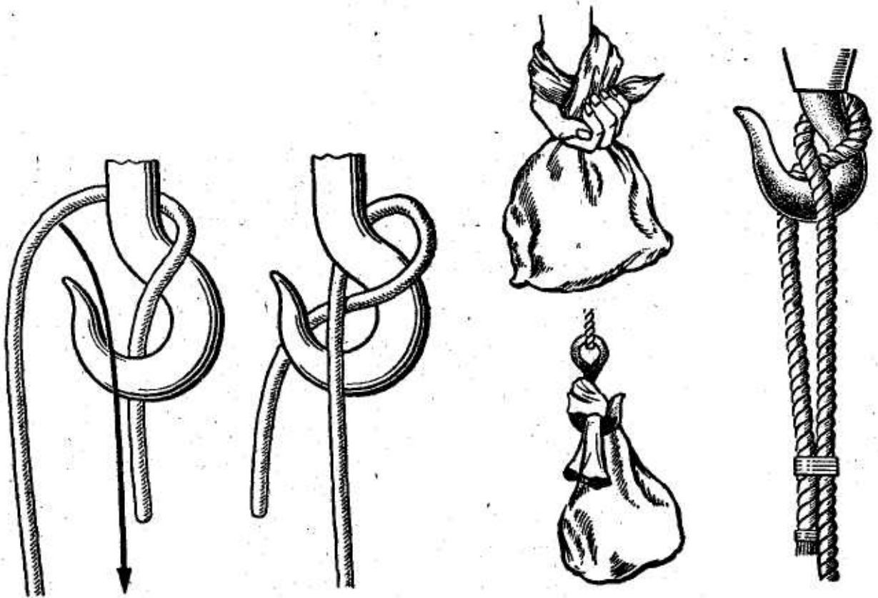
Рис. 105. Гачный узел
