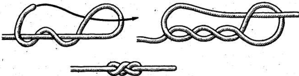
Рис. 4. Стивидорный узел
