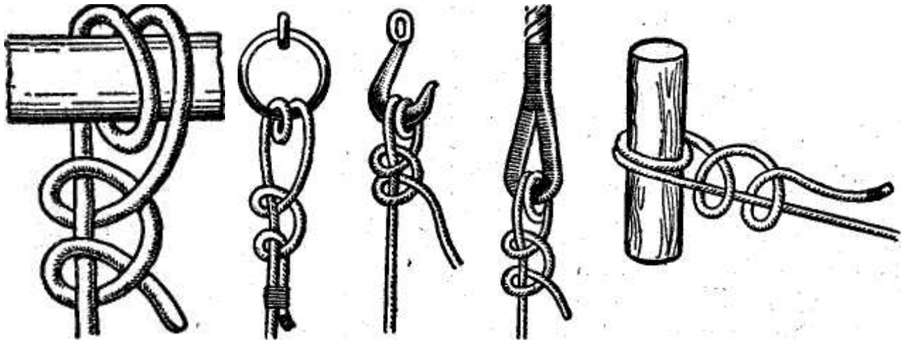
Рис. 12. Простой штык со шлагом
