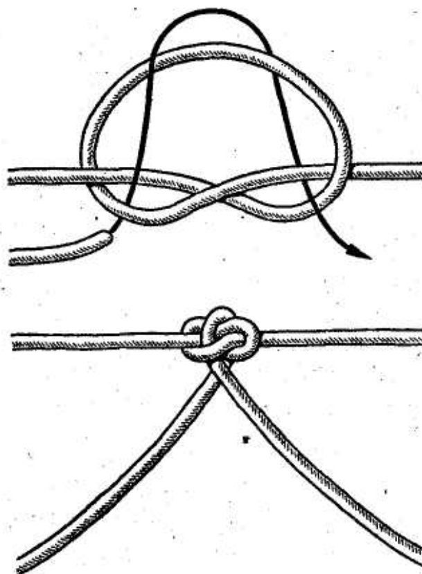
Рис. 130. Поводковый на основе простого узла
