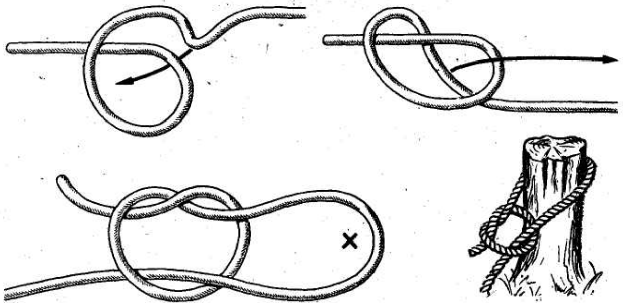
Рис. 82. Бегущий простой узел
