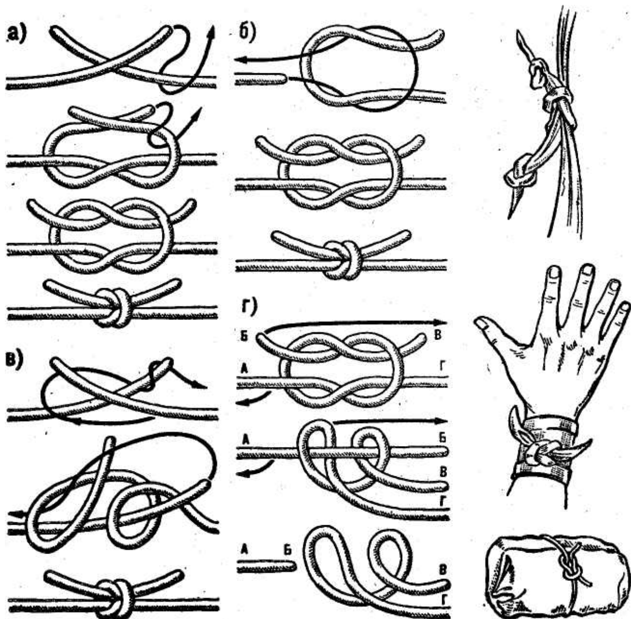
Рис. 25. Прямой узел:
