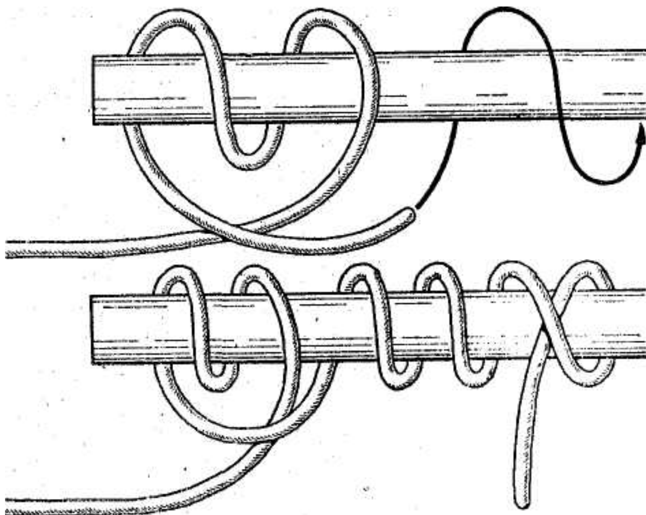
Рис. 60. Стопорный узел
