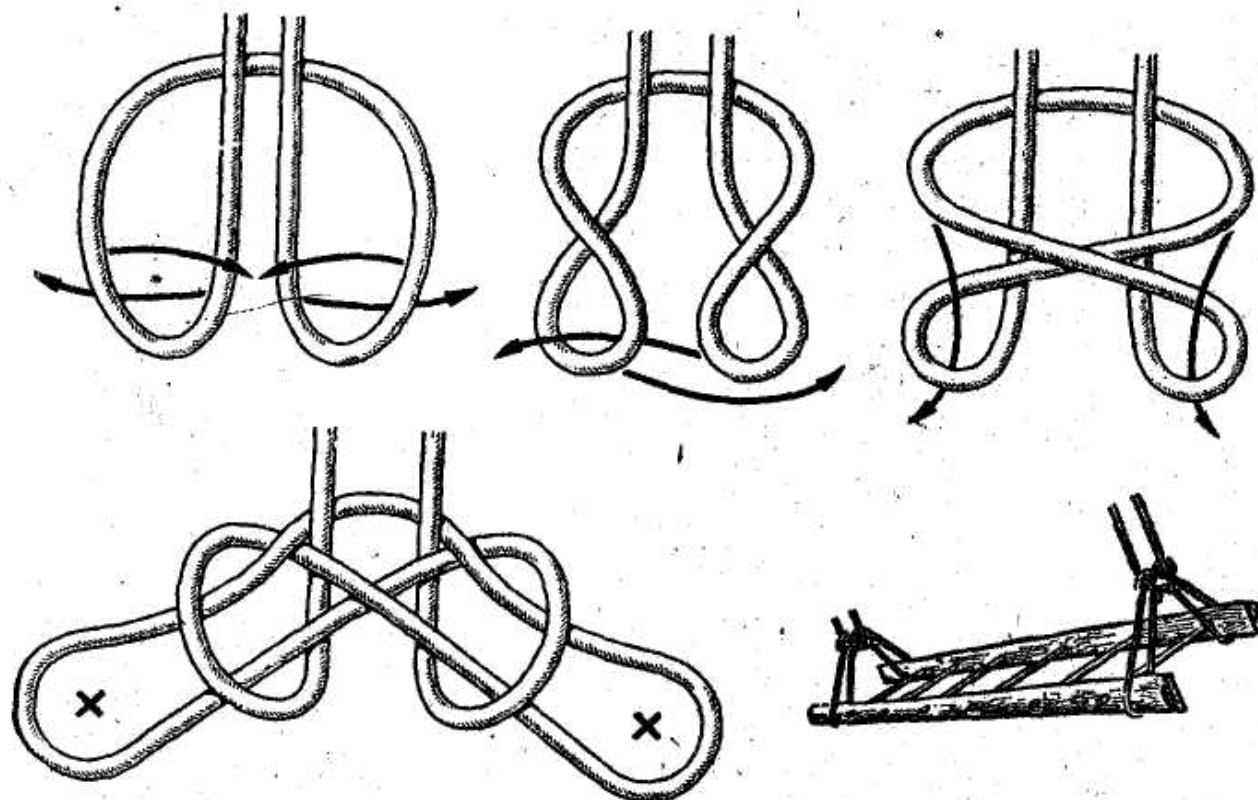
Рис. 78. Боцманский узел (испанский беседочный)
