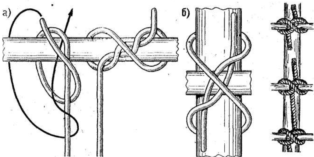
Рис. 52. Питонов узел: a — первый способ вязки; б — второй способ вязки
