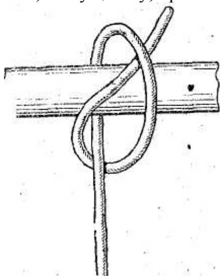
Рис. 44. Самозатягивающийся узел
