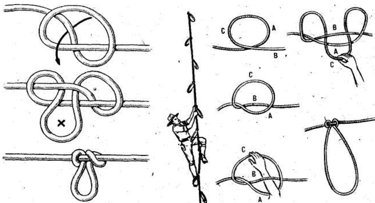
▲ Рис. 73. Бурлацкая петля
