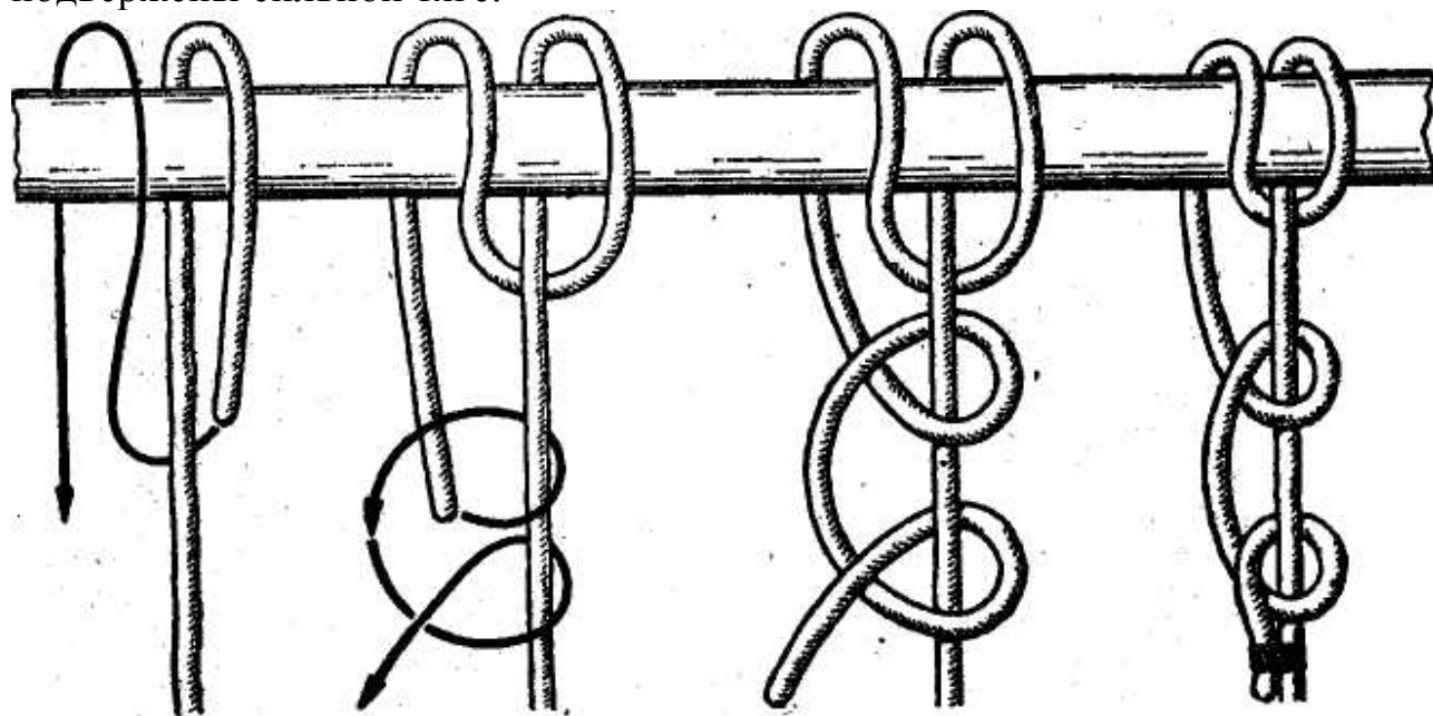
Рис. 14. Штык с обносом
