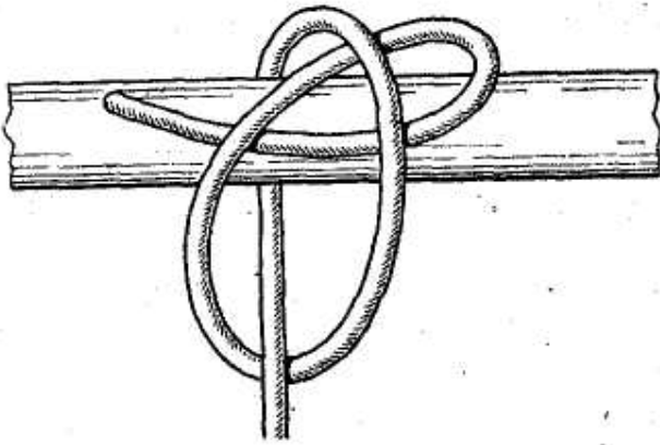
Рис. 98. Развязывающийся самозатягивающийся узел
