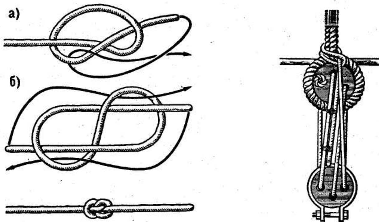
Рис. 5. Юферсный узел: а — первый способ вязки; б — второй способ вязки
