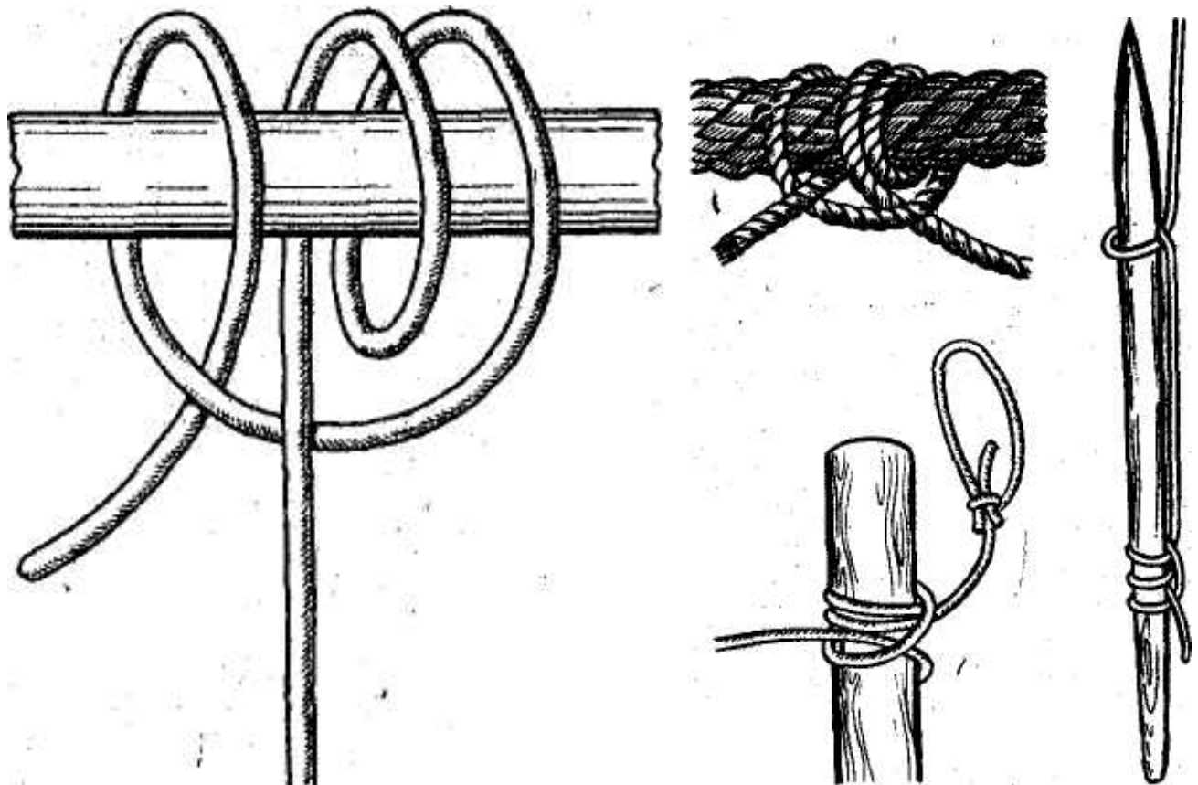
Рис. 49. Задвижной штык
