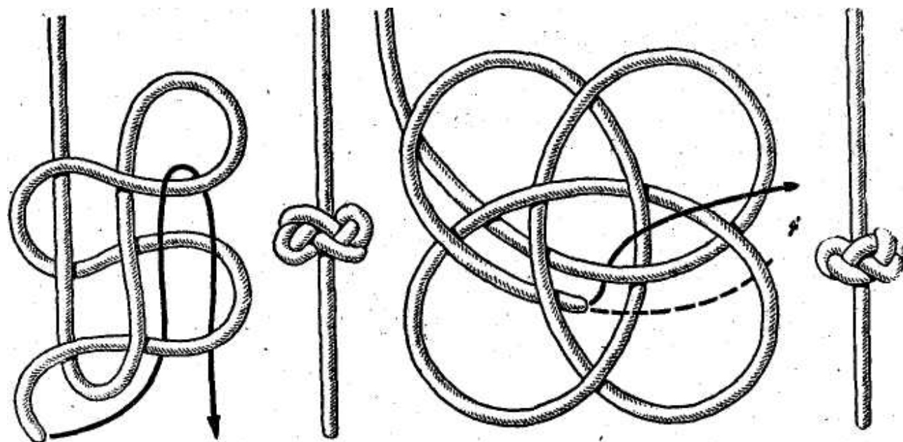
Рис. 137. Кордовый узел
