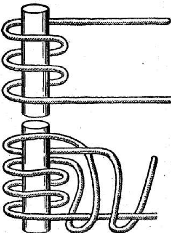
Рис. 19. Портовый узел
