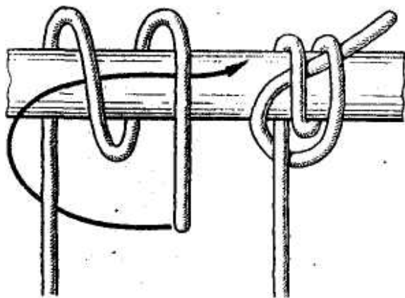
Рис. 55. Гафельный узел
