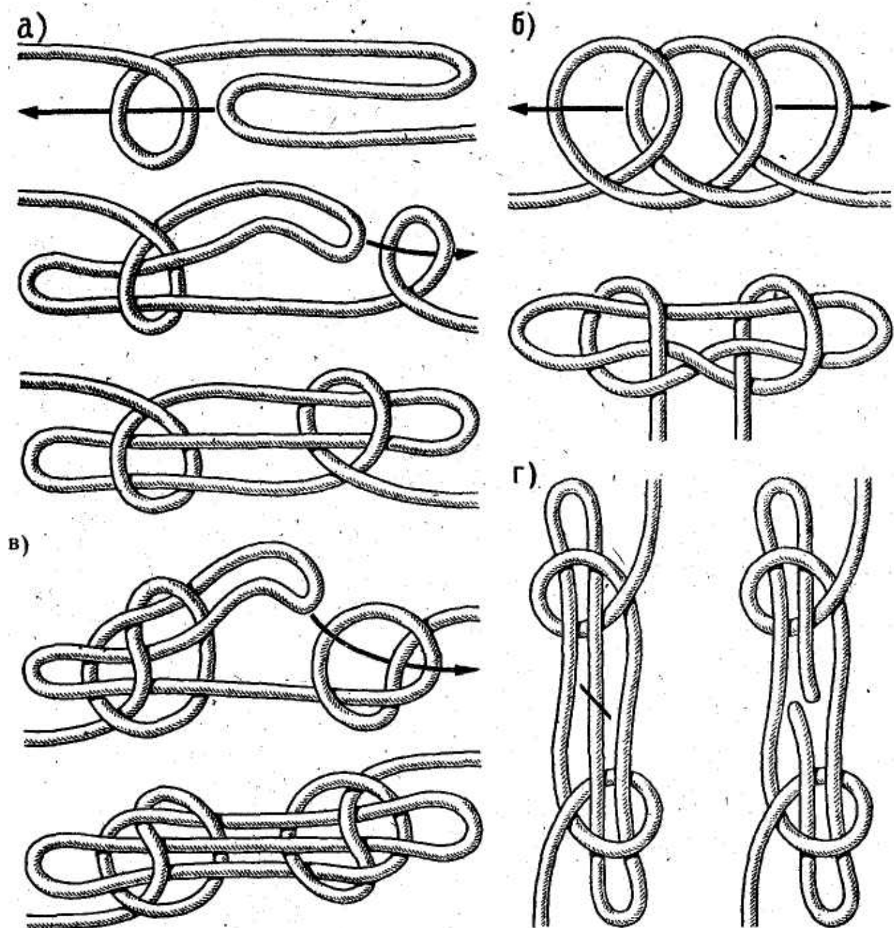
Рис. 113. «Баранья нога»:
