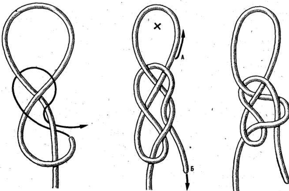
Рис. 118. Кабестановая петля
