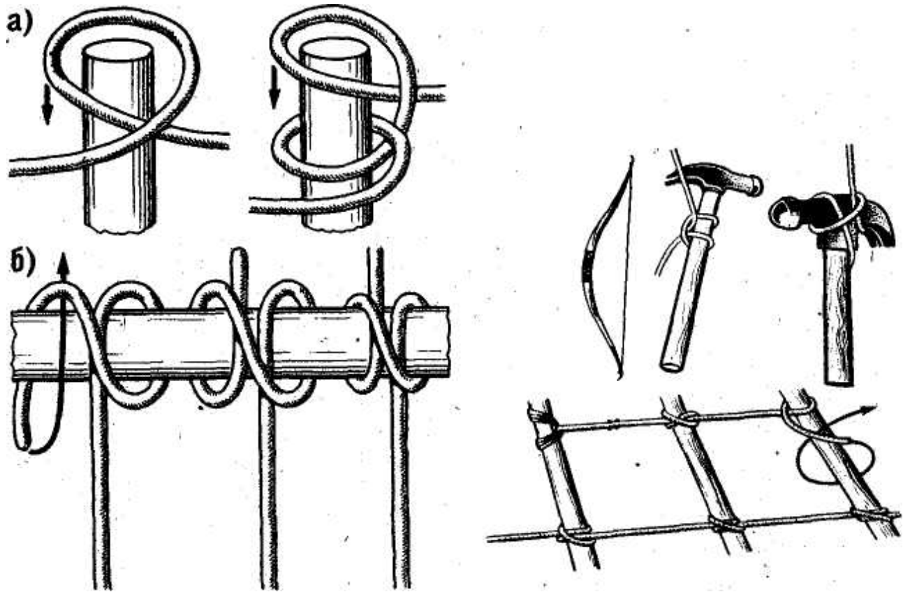
▲ Рис. 48. Выбленочный узел: a — первый способ вязки; б — второй способ вязки
