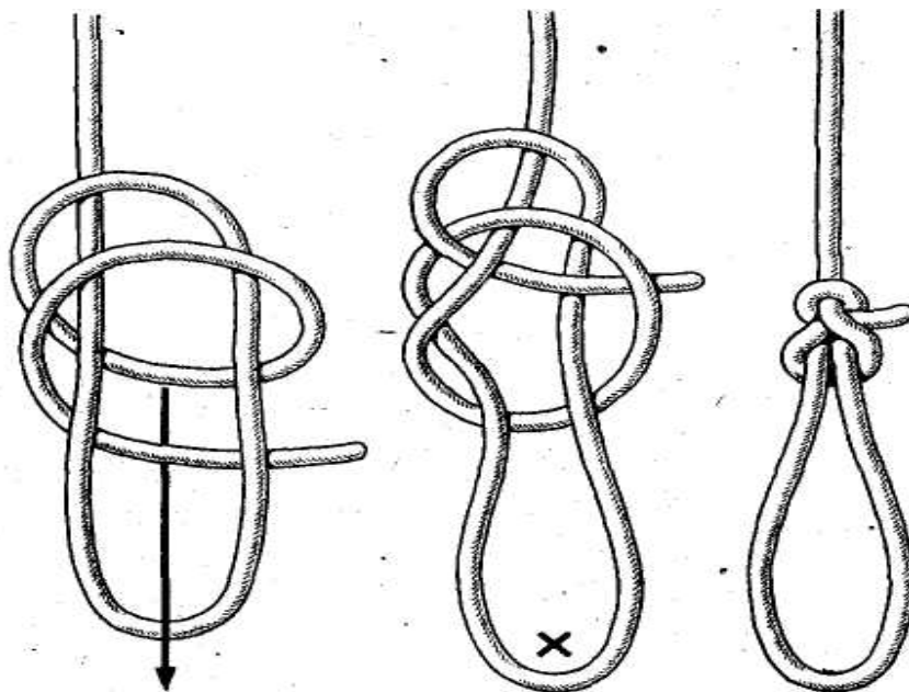
Рис. 71. Совершенная петля
