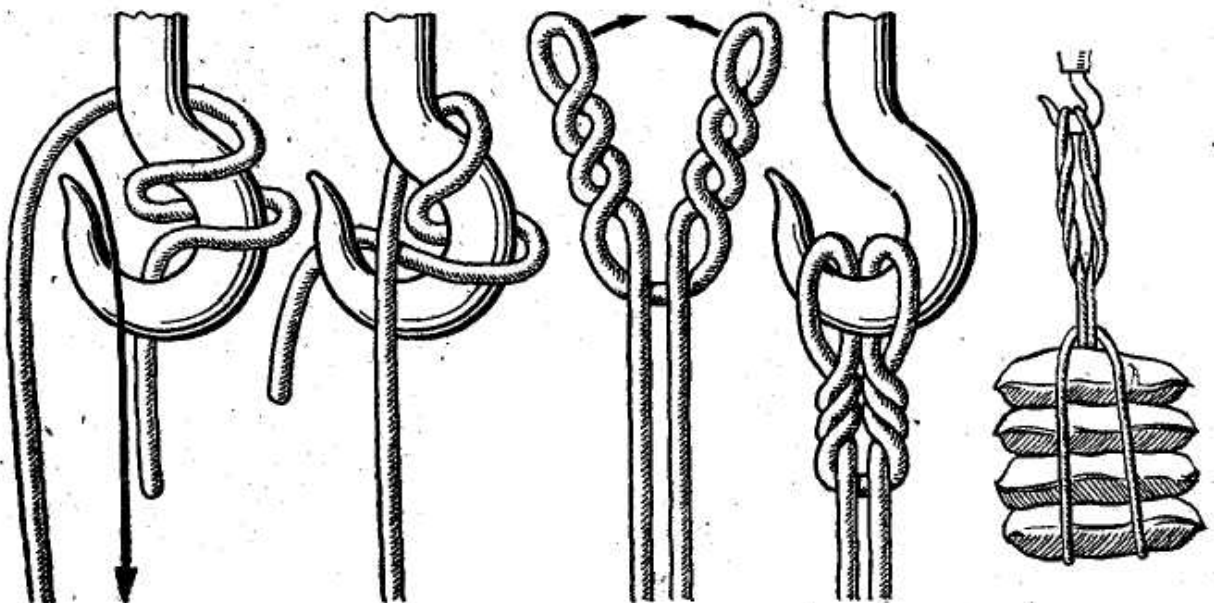
Рис. 106. Гачный узел со шлагом
