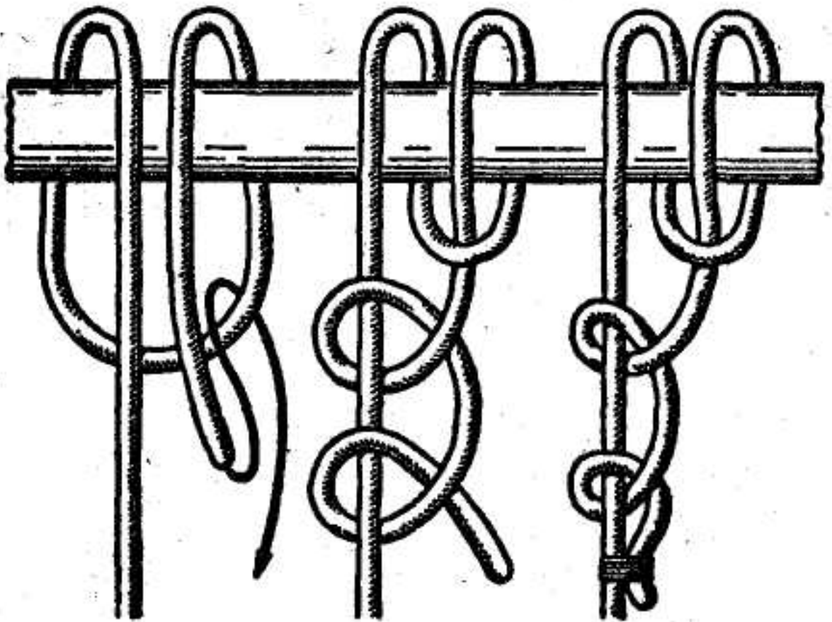
Рис. 16. Обратный штык
