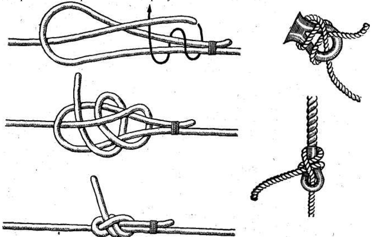
▲ Рис. 39. Брамшкотовый узел
