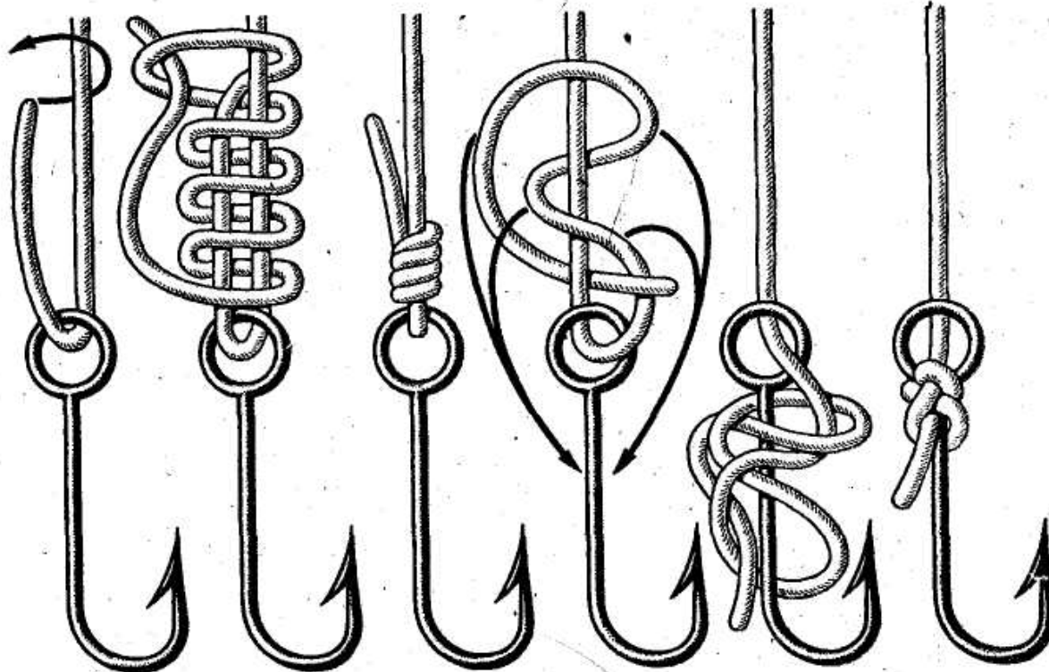
Рис. 127. Акулий узел
