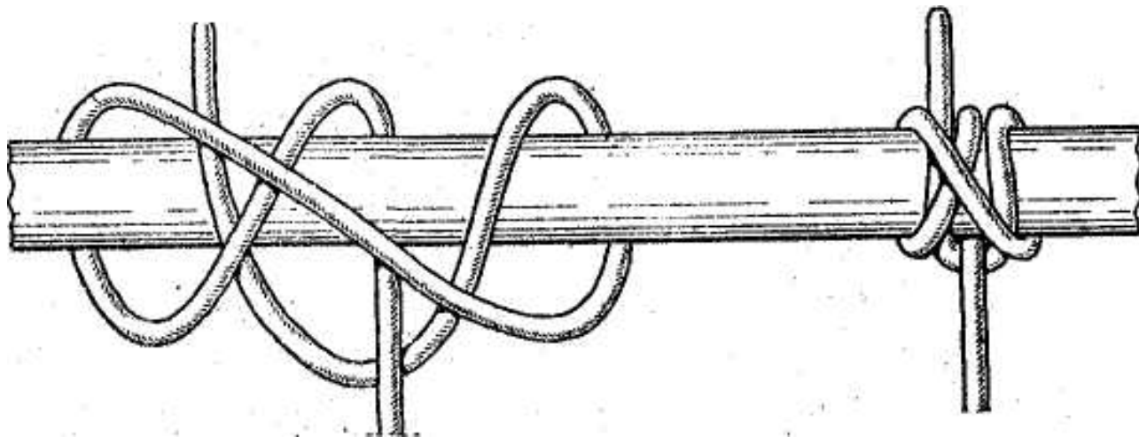
Рис. 61. Качельный узел
