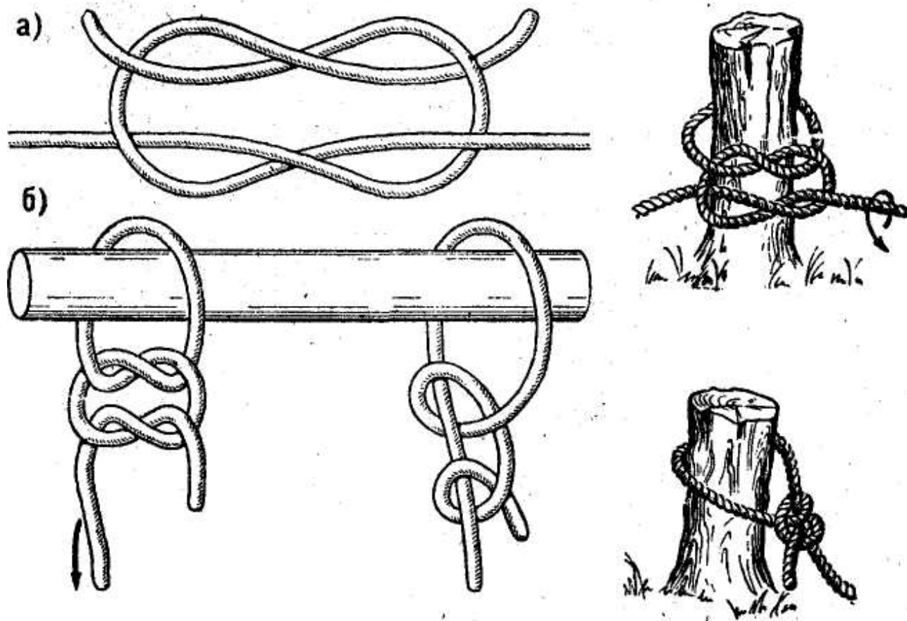
Рис. 23. Бабий узел:
