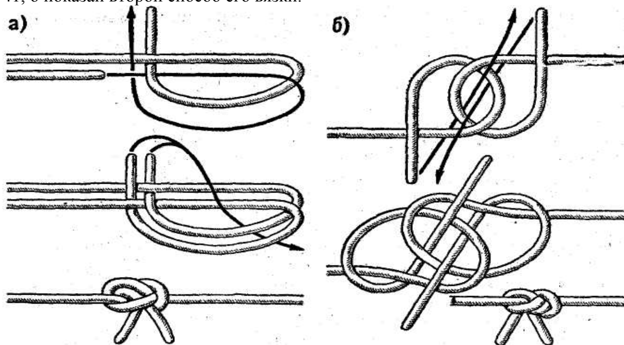
Рис. 41. Скорняжный узел: а — первый способ вязки; б — второй способ вязки
