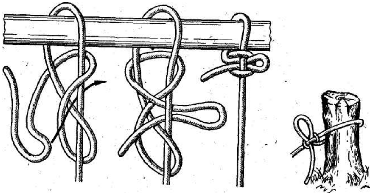
Рис. 102. Курьерский узел
