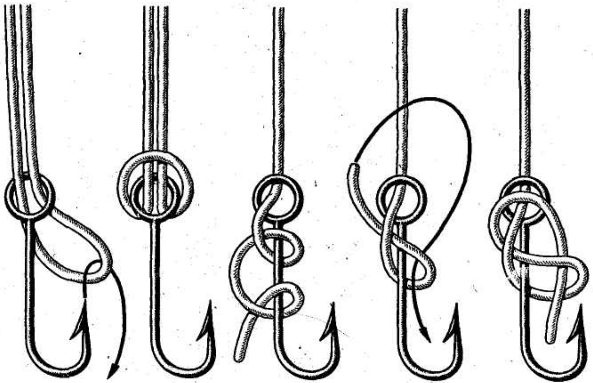
Рис. 119. Глухой узел
