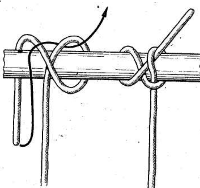
Рис. 54. Пикетный узел
