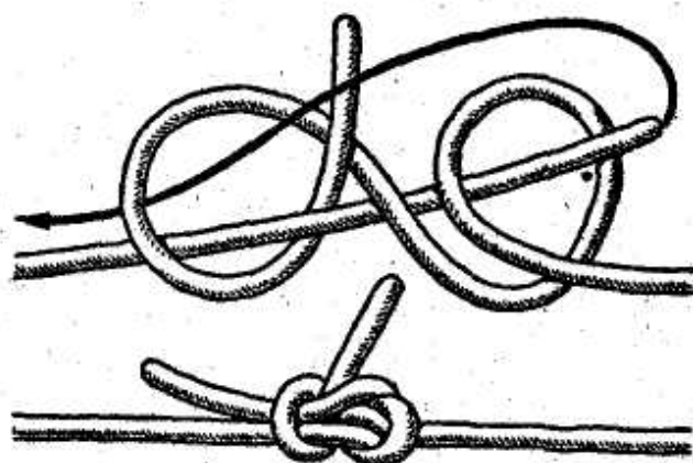
Рис. 37. Польский узел
