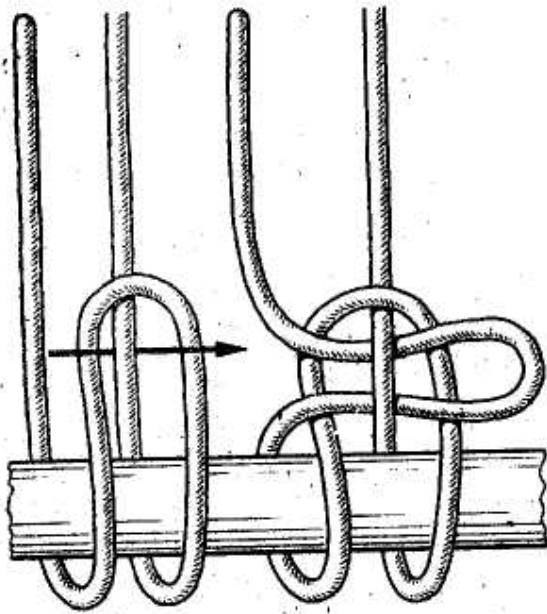
Рис. 103. Ведерный узел
