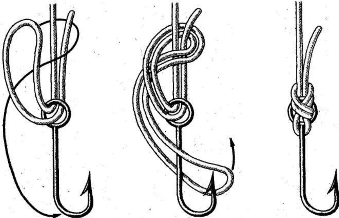
Рис. 124. Калифорнийский узел
