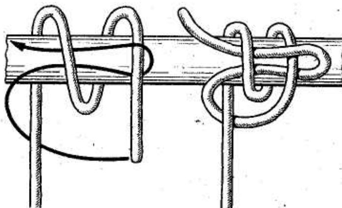
Рис. 56. Лисельный узел
