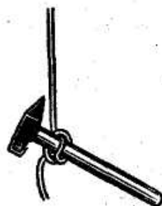
Рис. 110. Сваечный узел
