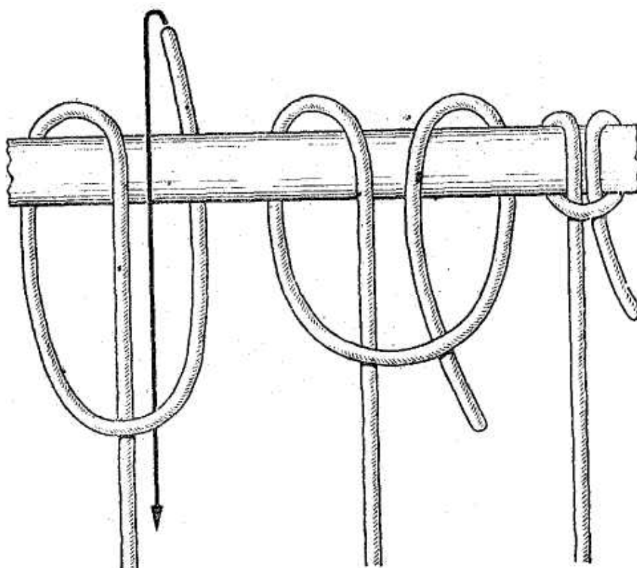
Рис. 46. Коровий узел
