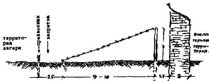
Поперечный разрез зоны спецлагеря или лагеря КТР.
