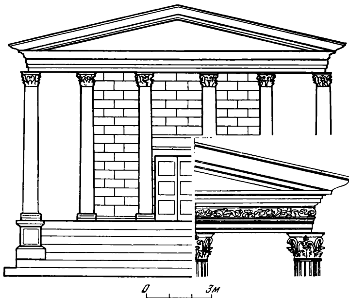
Рис. 5. Фасад коринфского периптера. Горгишия. Реконструкция автора
