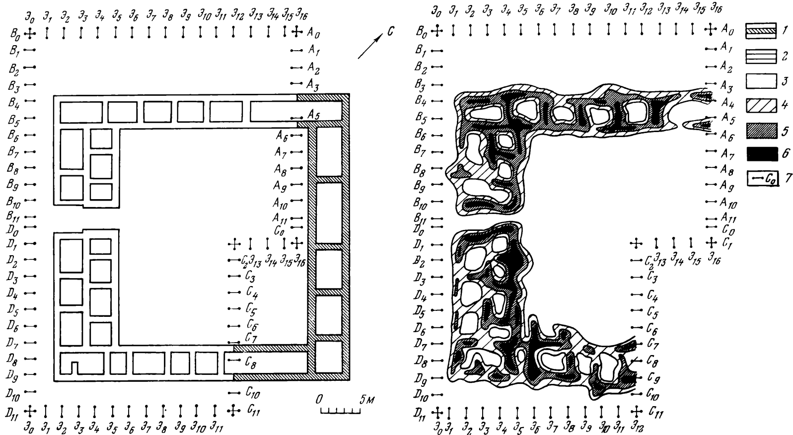
Рис. 2. Результаты электропрофиллирования методом срединного градиента
