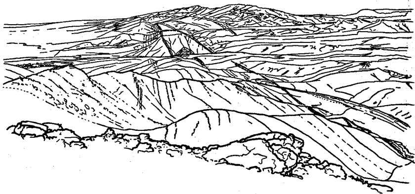
Рис. 7. Обнаженная полоса палеогена и неогена (от алайского до масагетского яруса) в Южной Фергане. (Рисунок по полевой зарисовке).
