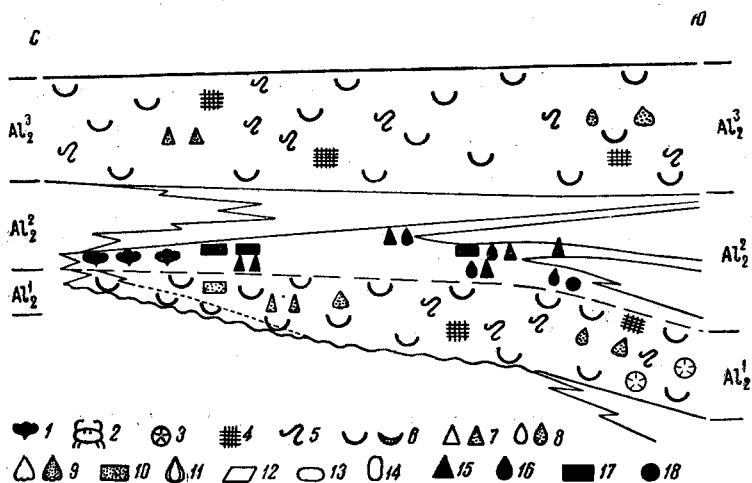
Рис. 10. Схема распределения фауны и флоры верхнеалайского времени ( Al_2 ) в северной части Ферганского залива (палеоэкологический профиль).
