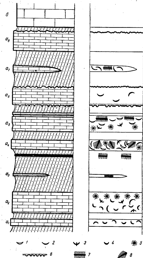
Рис. 3. Различная палеоэкологическая и био- стратомическая характеристика отдельных слоев из- известняков (1—8) при сохранении видового состава фауны. Толща переслаивания «а» нижнего карбо- на на р. Мсте выше г. Боровичи.
