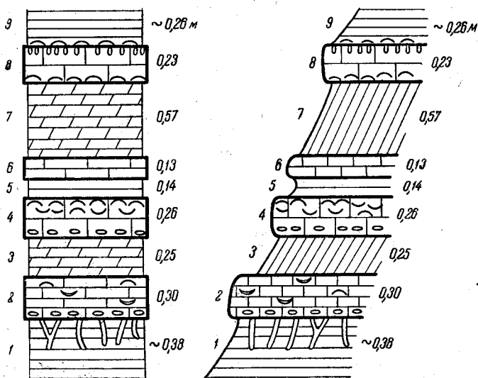
Рис. 4. Два различных способа схематического изображения разрезов.
