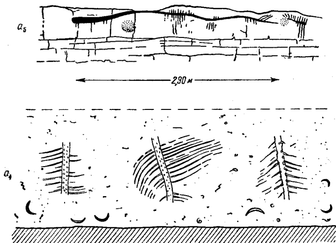
Рис. 5. Различно ориентированные створки Gigantoproductus и стигмарины в обнажениях (вертикальных стенках) двух слоев известняка ( a_4 и a_5 ) разреза нижнего карбона на р. Мсте выше г. Боровичи; см. рис. 3. (Полевые зарисовки).
