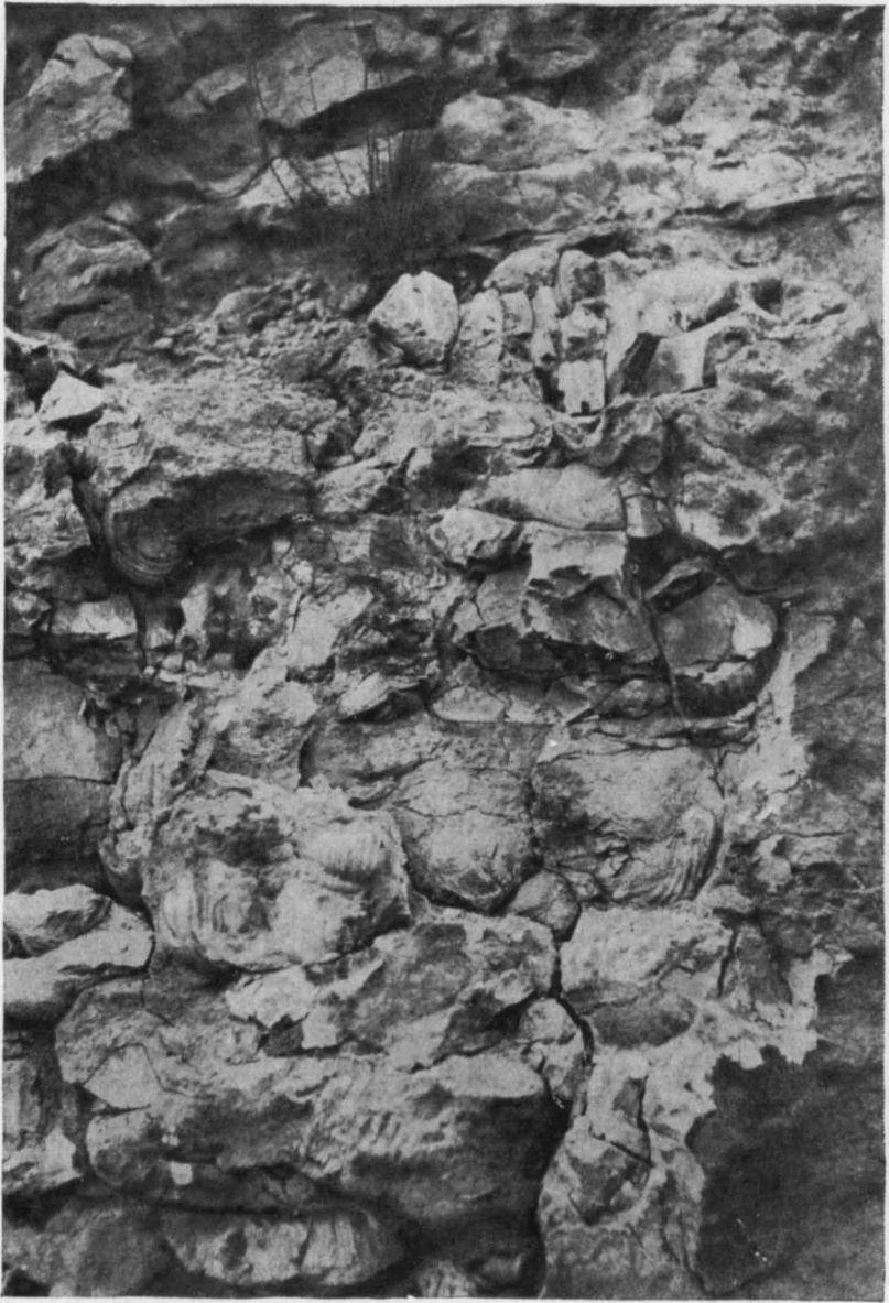
Банка, образованная раковинами Gigantoproductus giganteus (Mart.) с раковинами, сохранившимися с обеими створками в прижизненном положении. Нижний карбон. Стена карьера у д. Баранова Гора в верховьях Волги.
