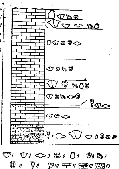
Рис. 8. Схематическое изображение части разреза артинских известняков Косого Камня на р. Юрезани с указанием распределения в нем фауны.
