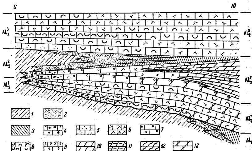
Рис. 9. Схема распределения осадков верхнеалайского времени ( Al_2 ) в северной части Ферганского залива (профиль осадков).
