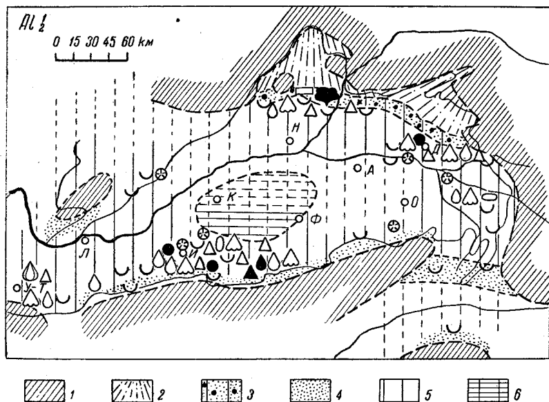
Рис. 12. Схематическая фациальная карта Ферганского залива в начале верхнеалайского времени ( Al_2^1 ) палеогеновой эпохи.
