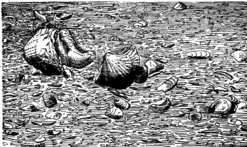
Рис. 6. Устричник, образованный раковинами Fatina и Flemingostrea . Крупные раковины Fatina с обеими створками; створки Flemingostrea разрознены. Южная Фергана, р. Исфара. (Полевой рисунок).
