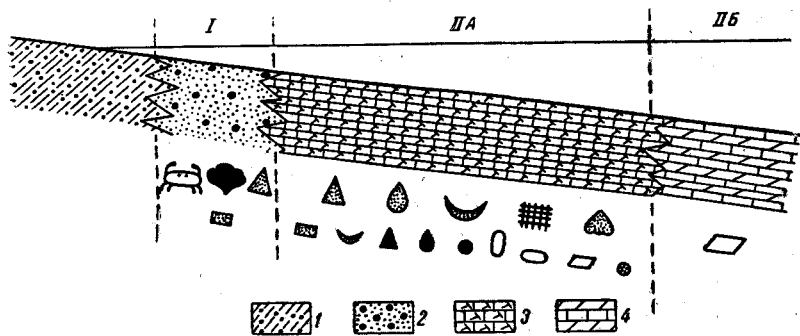
Рис. 11. Схема зонального и фаціального распределения фауны и флоры в Ферганском заливе в начале и в конце верхнеалайского времени ( Al_2^1 и Al_2^3 ) палеогеновой эпохи.
