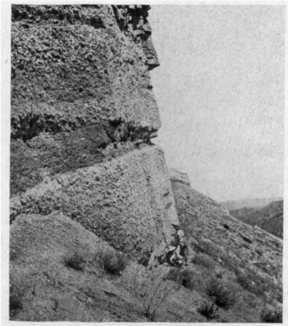
1. Обнажение с мощными слоями устричников, образованных раковинами Fatina . Туркестанский ярус палеогена в Северной Фергане.
