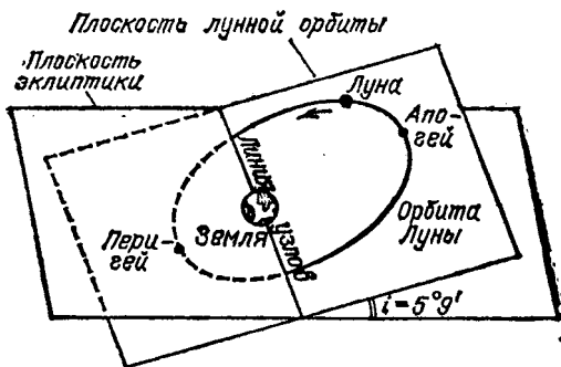
Рис. 38. Эллипс лунной орбиты
