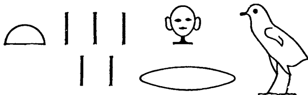
Рис. 74. Изображение эпагомен
