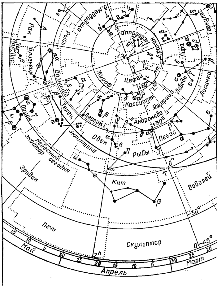
Рис. 26. Положение точки весеннего равноденствия сегодня (♈) и около 4000 г. до н.э. (♈'). Даты у края выполненной в форме круга карты звездного неба показывают положение Солнца на эклиптике в наше время; его определяем, двигаясь по прямой линии (по кругу склонений) от числа месяца к центру карты (к Северному полюсу мира) до пересечения с эклиптикой.
