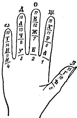
Рис. 95. Расположение букв и чисел на правой руке для определения круга Луны и исправной буквы
