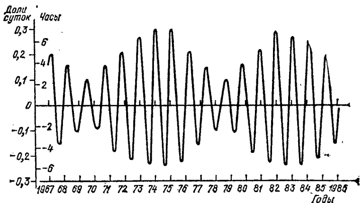
Рис. 36. Отклонение продолжительности синодических месяцев в 1967—1986 гг. от среднего значения
