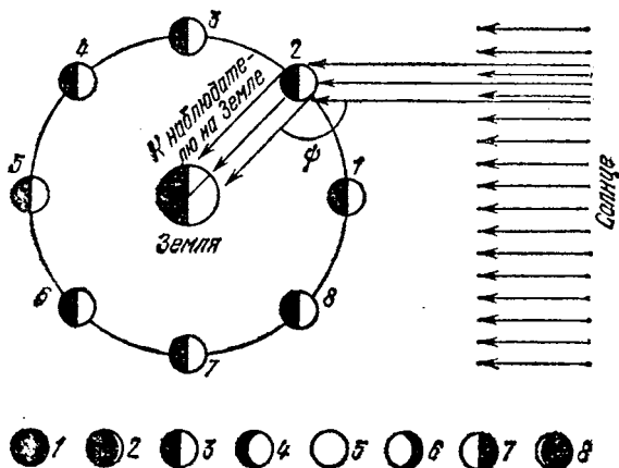
Рис. 35. Конфигурации (1 — конъюнкция, 8 и 7 — квадратуры, 5 — Противостояние) и фазы Луны (1 — новолуние, 3 — первая четверть, 5 — полнолуние, 7 — последняя, или третья четверть; 2, 4, 6, 8 — промежуточные фазы)
