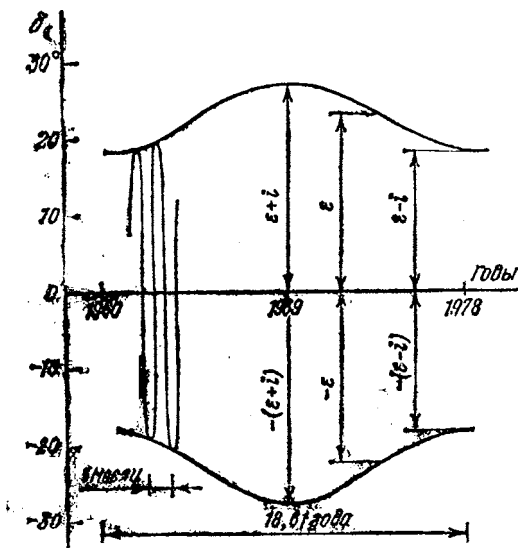
Рис. 39. Пределы изменения склонения Луны на протяжении 18,61 года
