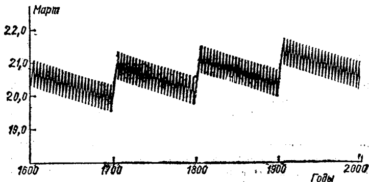
Рис. 48. Смещение моментов весеннего равноденствия от года к году в XVII—XX вв.; в каждые последующие 400 лет картина повторяется, сдвигаясь, однако, в целом вниз на 0,12 d
