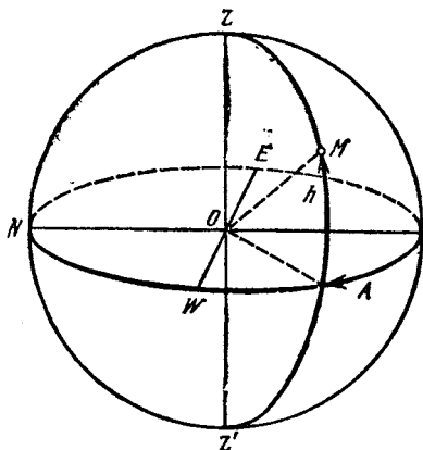
Рис. 6. Направление отсчета азимута A и высоты h светила
