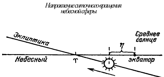
Рис. 9. Положение истинного Солнца и среднего экваториального солнца в момент их прохождения вблизи точки весеннего равноденствия
