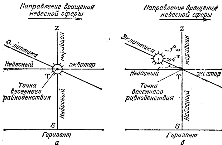
Рис. 20. К объяснению различия в продолжительности звездных и солнечных суток: если 20 марта центр диска Солнца находится в точке весеннего равноденствия \varphi в момент ее верхней кульминации (а), то за сутки к полудню 21 марта Солнце сдвинется к востоку почти на 1^\circ и поэтому центр его диска пройдет через небесный меридиан на 3 мин 56 с позже, чем точка \varphi (б)
