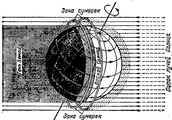
Рис. 7. Смена дня и ночи на Земле как следствие ее вращения вокруг своей оси
