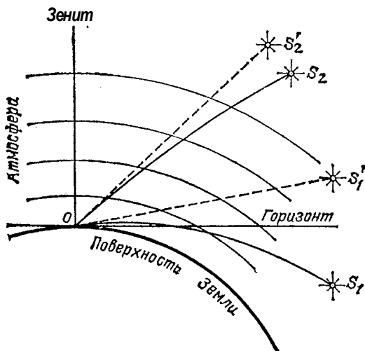
Рис. 13. Атмосферная рефракция. Луч, исходящий от светила 5 изгибается в земной атмосфере настолько, что оно видно и после того, как на самом деле уже находится за горизонтом
