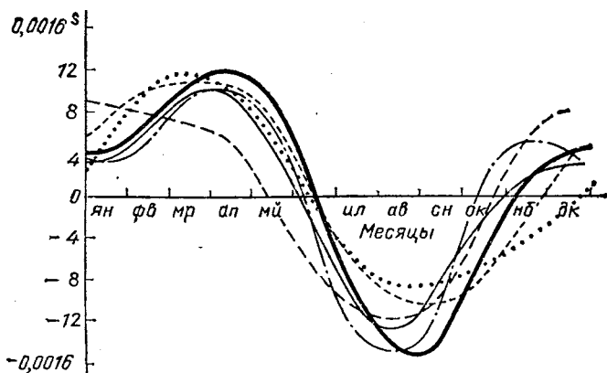
Рис. 15. Колебание продолжительности суток в течение года по данным различных служб времени (сглаженные кривые)
