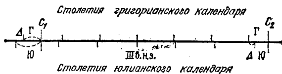
Рис. 89. К объяснению знака расхождения \Delta между датой \Gamma григорианского и датой \text{Ю} юлианского календарей: \Gamma = \text{Ю} + \Delta . Начала обеих систем совпадали в III в. н.э., в более отдаленное время начало года юлианского календаря, имеющего в среднем большую длительность года, удалено в прошлое дальше, чем начало года григорианского календаря.
