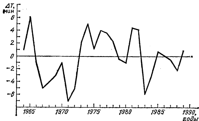
Рис. 25. Отклонение промежутка времени между двумя последовательными прохождениями центра диска Солнца через точку весеннего равноденствия от продолжительности тропического года в 1964—1989 гг.
