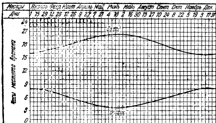
Рис. II. Изменение моментов восхода и захода Солнца и продолжительности дня в течение года для географической широты \varphi = 50^\circ
