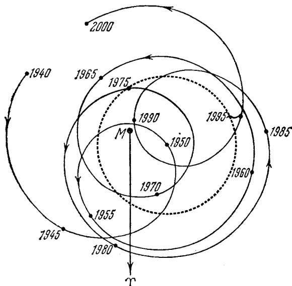
Рис. 32. Движение центра Солнца относительно центра масс Солнечной системы с 1940 по 2000 г. Пунктирный круг — положение Солнца в 1950 г. Центр масс отмечен точкой М; стрелка указывает направление на точку весеннего равноденствия в том же году
