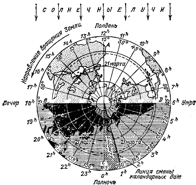
Рис. 21. Линия перемены даты
