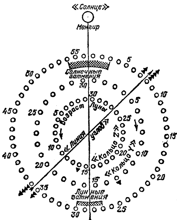
Рис. 58. Схема, объясняющая возможное использование лунок Стоунхенджа для предвычисления солнечных и лунных затмений. Указано положение «каменной узлов», «каменя возраста Луны» (в кольце Z) и «каменя поправок в положении узлов» (в кольце Y) на 44-й день после солнечного затмения
