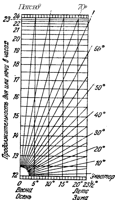
Рис. 12. Номограмма для графического определения продолжительности дня (подробности в тексте)
