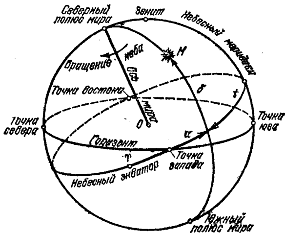
Рис. 9. Направление отсчета экваториальных координат \alpha и \delta , а также часового угла t звезды
