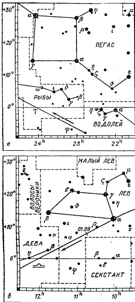
Рис. 3. Положение точки весеннего равноденствия \varphi (а) и точки осеннего равноденствия \Omega (б) на небесной сфере. По горизонтали отложено прямое восхождение \alpha , по вертикали — склонение \delta ; стрелкой указано направление движения Солнца по эклиптике; дата 01.09 на рис. б указывает положение Солнца на начало сентября
