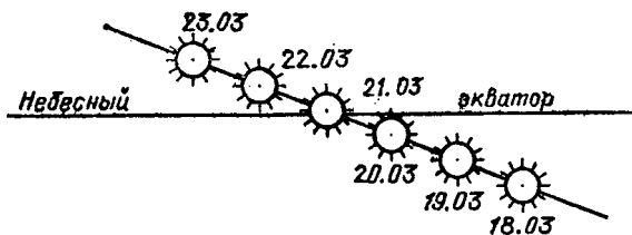
Рис. 4. Переход Солнца через точку весеннего равноденствия \varphi
