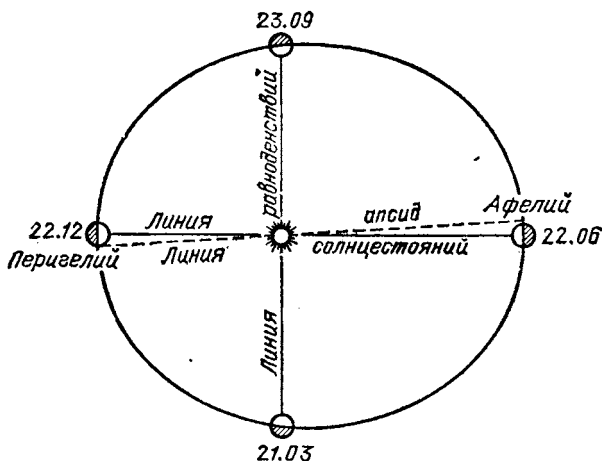
Рис. 31. Положение линии апсид земной орбиты относительно линии солнцестояний в наши дни
