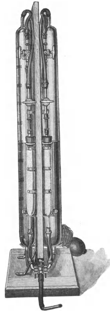
Abb. 20. Pneumothoraxapparat nach v. MURALT. Seitenansicht.
